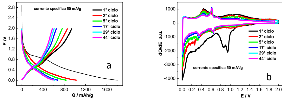
Fig. 25. Profili E vs Q (a) e dQ/dE vs E (b) dell'elettrodo \text{SnO}_2/\text{RGO}/\text{PAA} .
