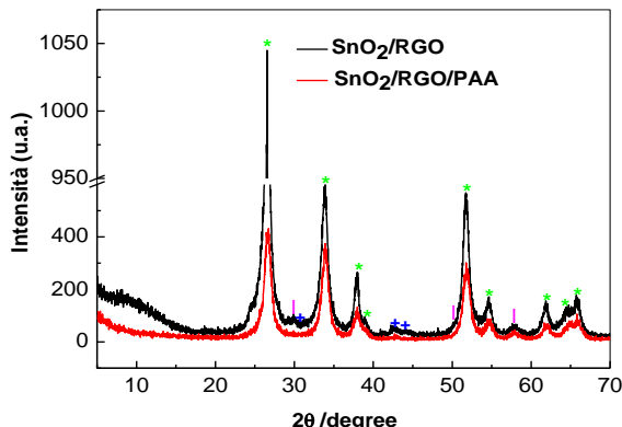
Fig. 19. Diffrattogrammi dei prodotti SnO 2 /RGO/PAA e SnO 2 /RGO. Sorgente Cu Kα, λ=1.54 Å.
