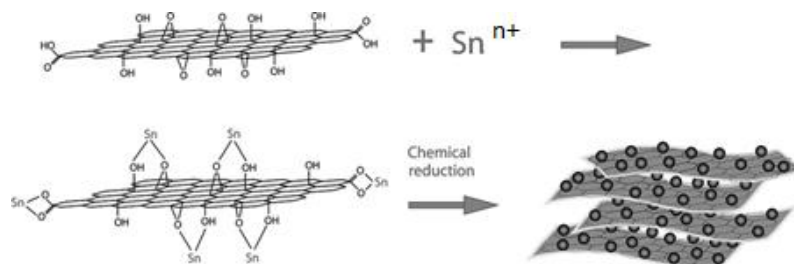
Figura. 10. Composito \text{SnO}_x/\text{RGO} .
