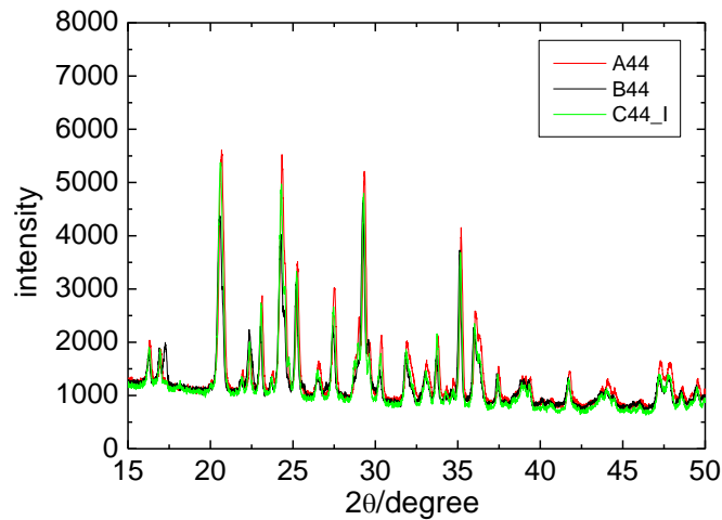
Figura 24 25. XRD delle polveri 0,6 \text{ LiMnPO}_4 \cdot 0,4 \text{ Li}_3\text{V}_2(\text{PO}_4)_3 da sintesi A, B e C
