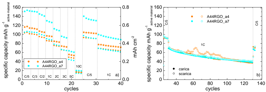
Figura 19. (a) Capacità specifica (cerchio, \text{mAh g}^{-1}_{\text{LMVP}} ) e capacità su \text{cm}^2 (stella) vs. numero di cicli durante i test con carica CC(C/5)-CV e scarica CC a diverse C-rate e (b) capacità specifica di carica e scarica durante i test di stabilità CC(1C)-CV/CC(1C) in LP30 a 30°C tra 2,5 V e 4,5 V degli elettrodi A44/RGO/C65_a4 ( 5,64 \text{ mg cm}^{-2} ) e A44/RGO/C65_a7 ( 7,22 \text{ mg cm}^{-2} ).
