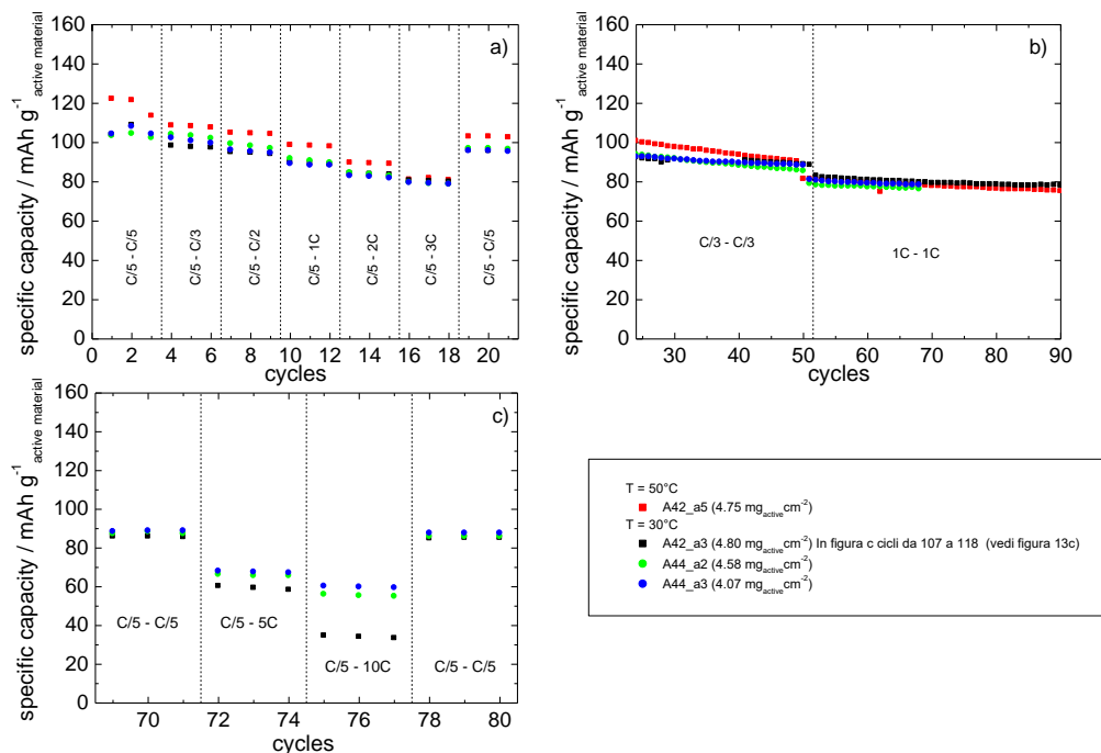
Figura 20. Capacità di scarica ( \text{mAh g}^{-1}_{\text{LMVP}} ) vs. numero di cicli degli elettrodi A42_a3 e A44_a3 a 30°C e A42_a5 a 50°C durante i test di discharge capability (a) e di stabilità a ripetuti cicli (b) e degli elettrodi A42_a2, A44_a4 e A44_a3 durante i test di discharge capability ad elevate C-rate (c) a 30°C in LP30 con cariche CC-CV e scariche CC tra 2,5 V e 4,5 V.
