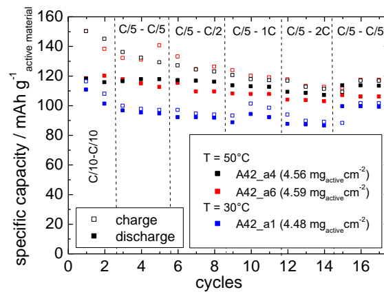
Figure 11. Capacità di carica e scarica (mAh g -1 LMVP ) vs. numero di cicli durante i test con carica CC(C/5)-CV e scarica, con scariche a diverse C-rate, tra 2,5 e 4,5 V in LP30 degli elettrodi A42_a4 e A42_a6 a 50°C e A42_a1 a 30°C. L'elettrodo A42_a6 ha effettuato cariche CC a partire dal 7° ciclo, l'elettrodo A42_a1 a partire dal 1° ciclo.
