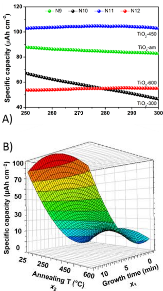
Figura 8. A) Valori di capacità specifica misurati a 0,1 \text{ mA cm}^{-2} per celle a ioni sodio assemblate con tappetini di NT \text{TiO}_2 come elettrodi (tempo di crescita 10 min) tra il 250° e il 300° ciclo; B) Curva di superficie raffigurante l'effetto della temperatura di ricottura e il tempo di crescita sulla capacità specifica al 250° ciclo in celle al sodio su scala da laboratorio.
