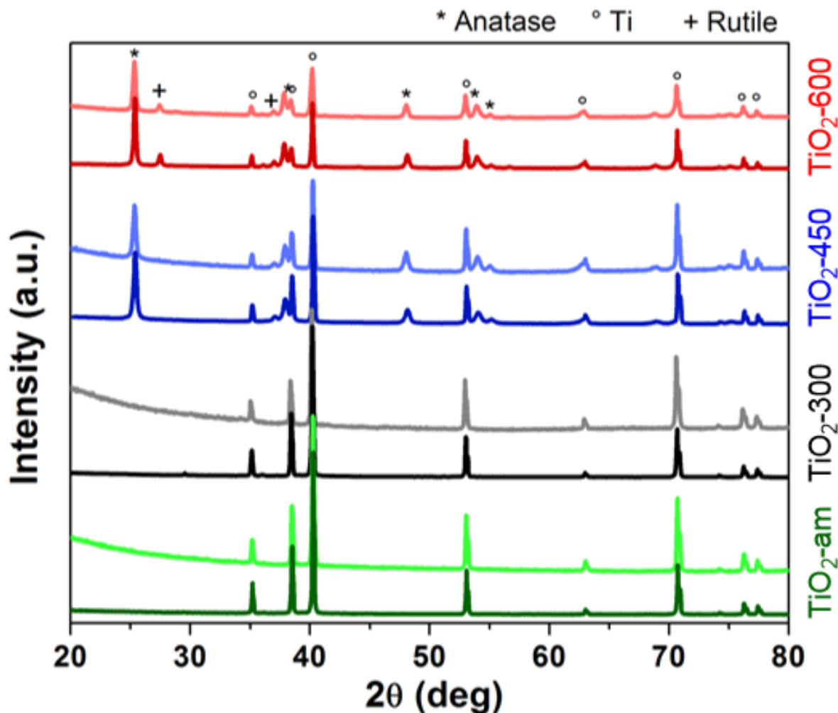
Figura 3. Pattern XRD di campioni di NT TiO 2 non trattati termicamente oppure trattati a 300, 450, 600 °C. I toni di colore più scuri indicano i campioni prima della ciclazione galvanostatica, mentre quelli più chiari indicano gli elettrodi dopo la ciclazione. Il tempo di crescita per anodizzazione è stato mantenuto costante e pari a 5 min.
