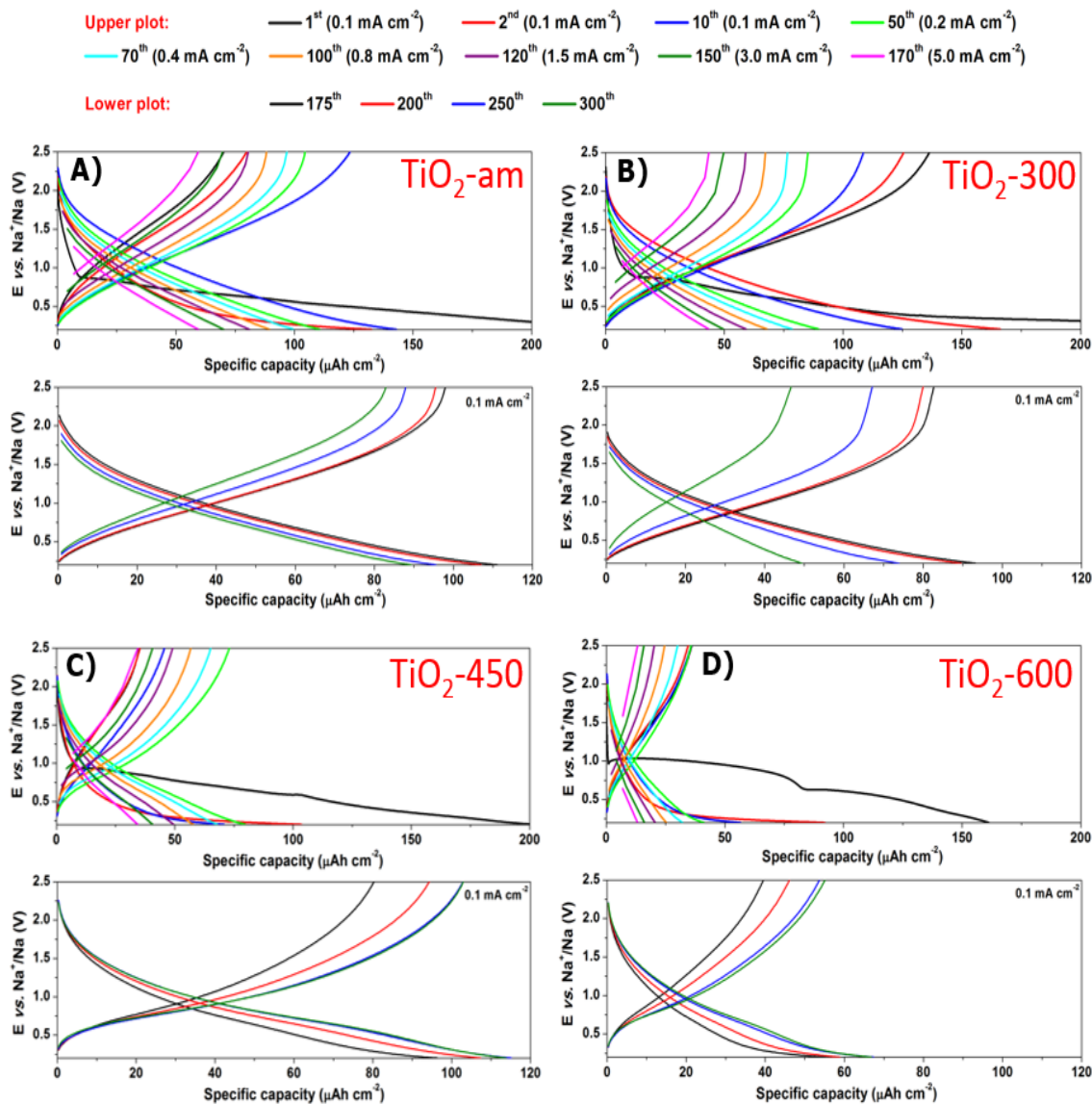
Figura 6. Comportamento elettrochimico a temperatura ambiente dei differenti tappetini di nanotubi in fase di studio: TiO 2 -am (A), TiO 2 -300 (B), TiO 2 -450 (C) e TiO 2 -600 (D). In particolare, sono mostrati profili di potenziale di scarica/carica a corrente costante in funzione della capacità specifica tra i cicli 1 e 170 a densità di corrente da 0,1 a 5 mA cm -2 (grafici superiori nelle figure da A a D) e tra i cicli 170 e 300 a densità di corrente fissa a 0,1 mA cm -2 (grafici in basso nelle figure da A a D).
