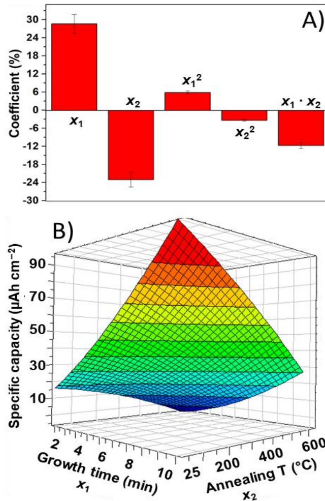
Figura 7. A) Diagramma dei coefficienti per il D-optimal DoE; B) Superficie di risposta in cui sono visibili gli effetti dei due parametri sperimentali sulla capacità all'85° ciclo di celle al sodio su scala da laboratorio assemblate con diversi tappetini di NT di TiO 2 .
