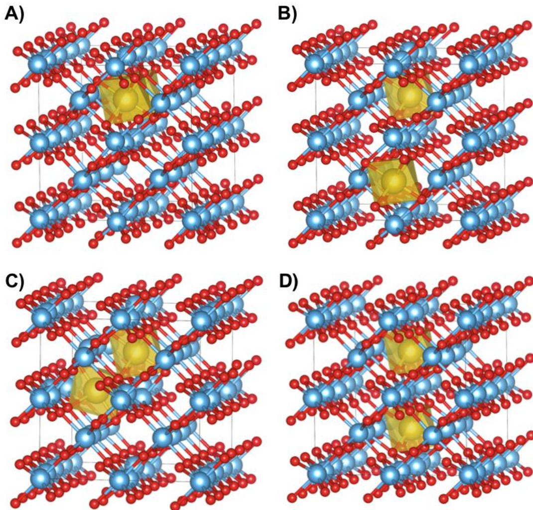
Figura 10. Modelli strutturali per un secondo catione Na^+ collocato in differenti configurazioni: A) adiacente lungo lo stesso canale in direzione [001]; B) nella posizione più lontana all'interno della supercella di 96 atomi; C) nel sito adiacente in un canale parallelo in direzione [001]; D) in un canale [001] parallelo collegato da un gruppo TiO_6 : il Ti centrale di tale gruppo va fortemente fuori posizione dopo il rilassamento strutturale. Ti in azzurro, O in rosso, Na^+ in giallo.
