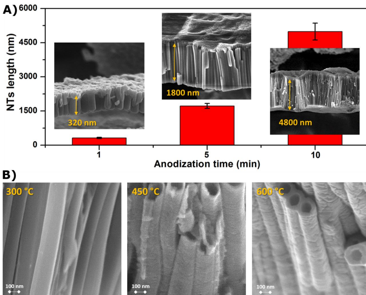
Figura 4. A) Grafico della lunghezza dei nanotubi in funzione del tempo di anodizzazione con relative immagini FESEM raffiguranti differenti lunghezze dei NT. B) Immagini FESEM a elevato ingrandimento dei nanotubi ricotti a differenti temperature (300, 450, 600 °C) per 1 h in atmosfera ambiente.
