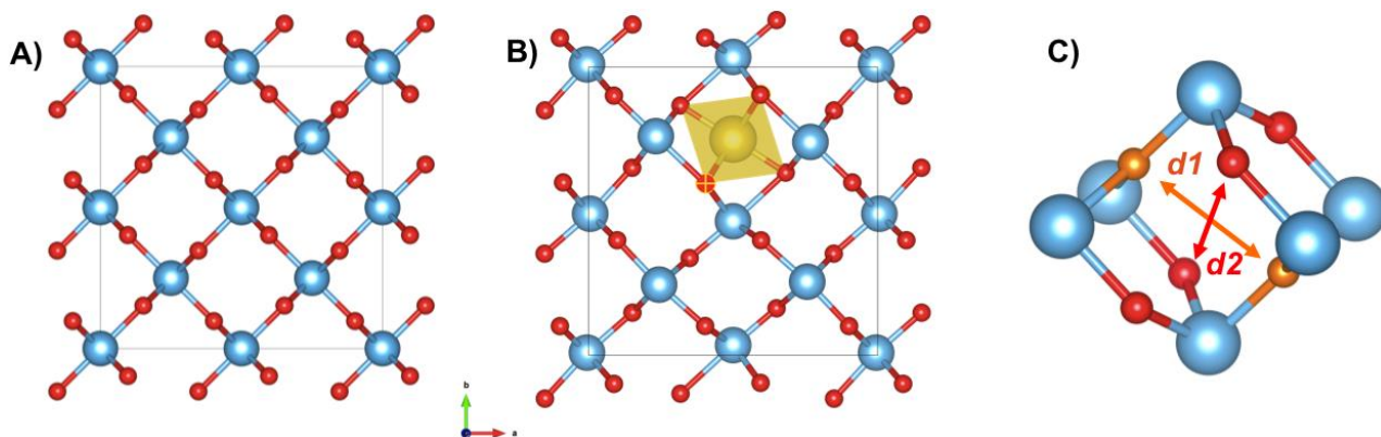
Figura 9. A) Modello strutturale in assenza di sforzi di una supercella 2x2x4 di 96 atomi di rutilo, visto lungo la direzione [001], Ti in azzurro, O in rosso. B) Struttura a minima energia per l'inserzione del catione Na + (in giallo) dentro il rutilo. C) Particolare su di una "gabbia" ospite Ti 6 O 6 per ioni Na + dove è mostrata la coordinazione dei 6 atomi di ossigeno. La misura di questa gabbia è determinata dai due atomi di ossigeno più vicini ( d1 in arancione), mentre altre due coppie equivalenti di O-O ( d2 in rosso) si trovano a distanza maggiore: d1 va da 3,36 Å nel rutilo puro a 4,01 Å in presenza di sodio (Na 0,03 TiO 2 ), d2 va da 4,49 Å a 4,41 Å.
