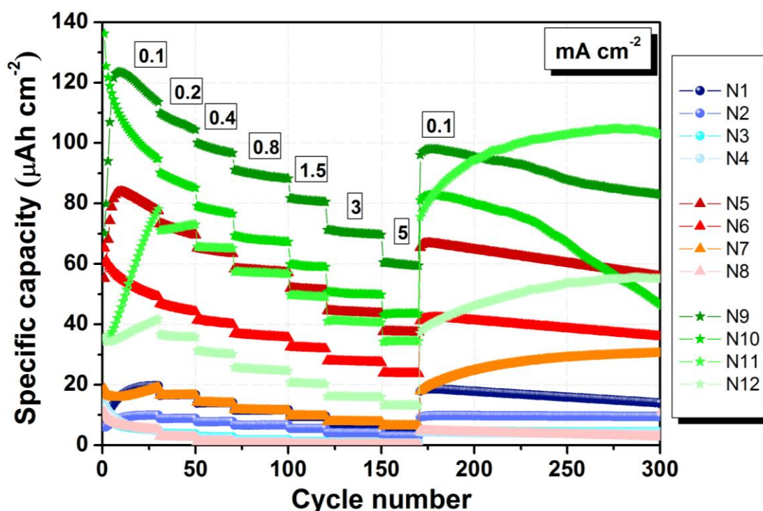
Figura 5. Capacità specifica in scarica in funzione del numero di cicli a differenti densità di corrente (da 0,1 a 5 mA cm -2 ) per celle al sodio assemblate con tappetini di NT TiO 2 (riferirsi alla Tabella 1 per le caratteristiche dei vari elettrodi).
