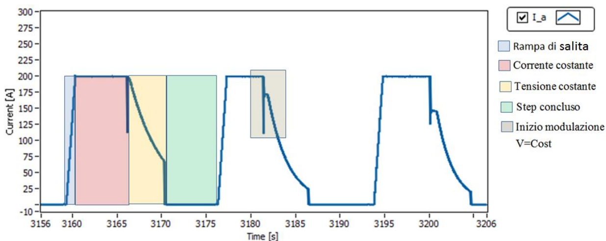
Figura 11. Andamento della corrente di linea nella prova a I_{max}=200\text{ A}
