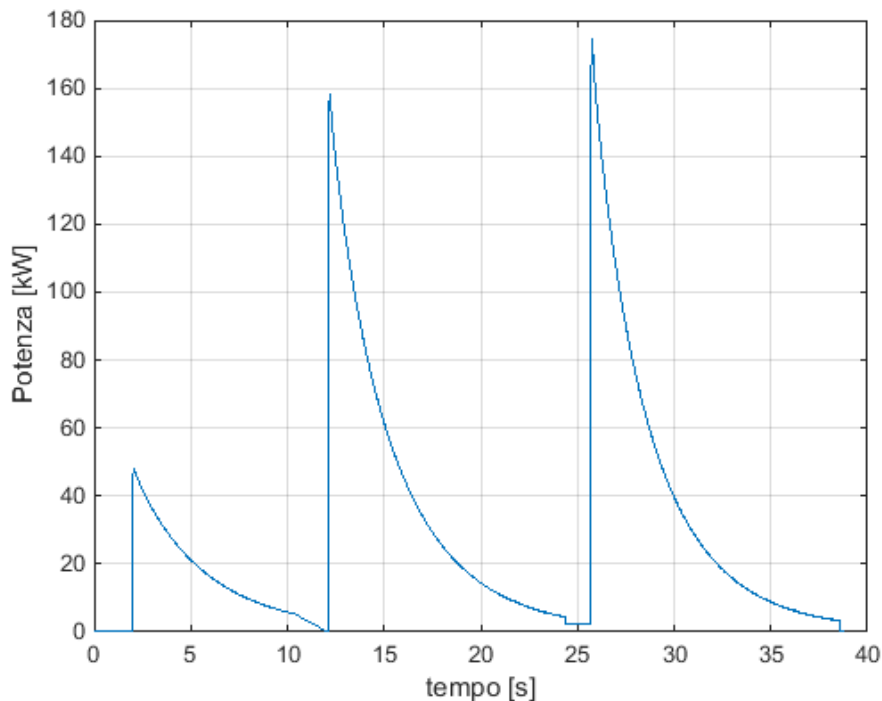
Figura 7 Potenza assorbita dagli SC di bordo nella ricarica a V_b=190\text{ V}
