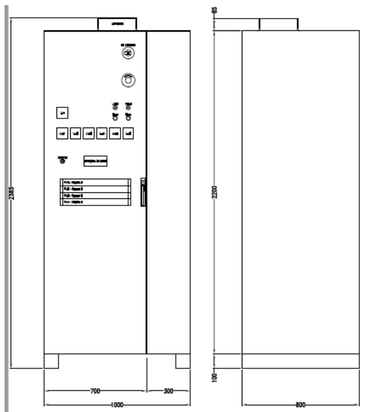
Figura 6. Dimensioni dell'armadio
