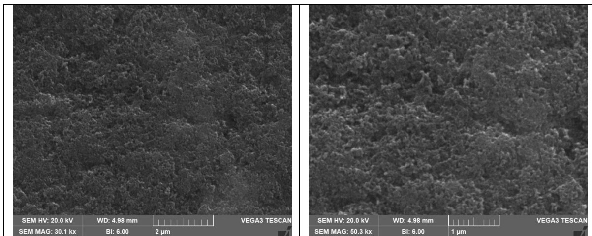
Figura 5 immagini SEM elettrodo composito
