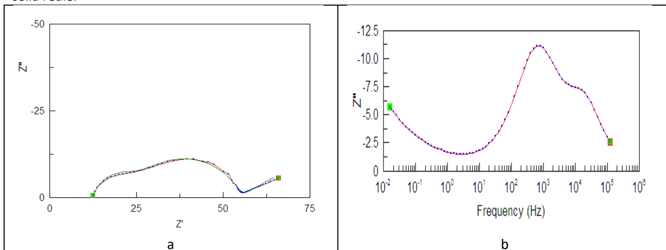
Figura 16 spettro d'impedenza batteria allo stato solido. Diagramma di Nyquist (a) diagramma di Bode (b)
