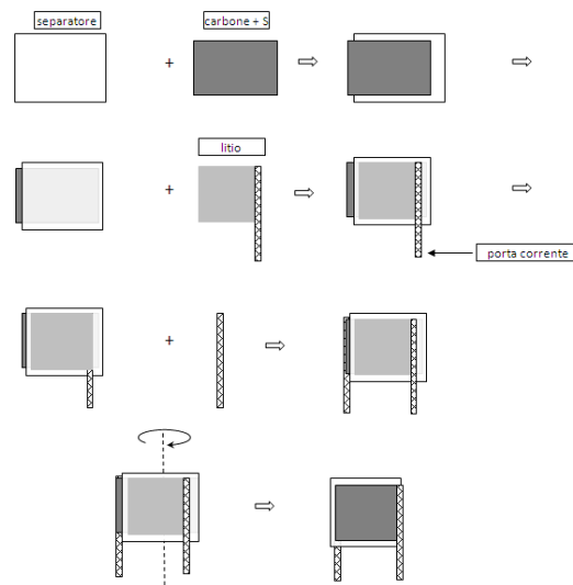
Figura 4 configurazione monopolare di una batteria
