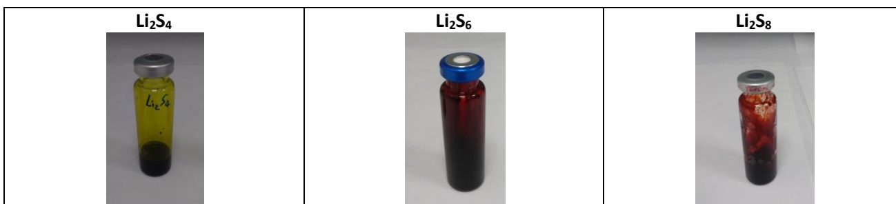
Figura 1 Soluzioni di polisolfuri in TEGDME
