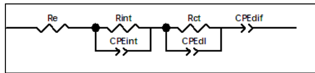
Figura 17 circuito equivalente
