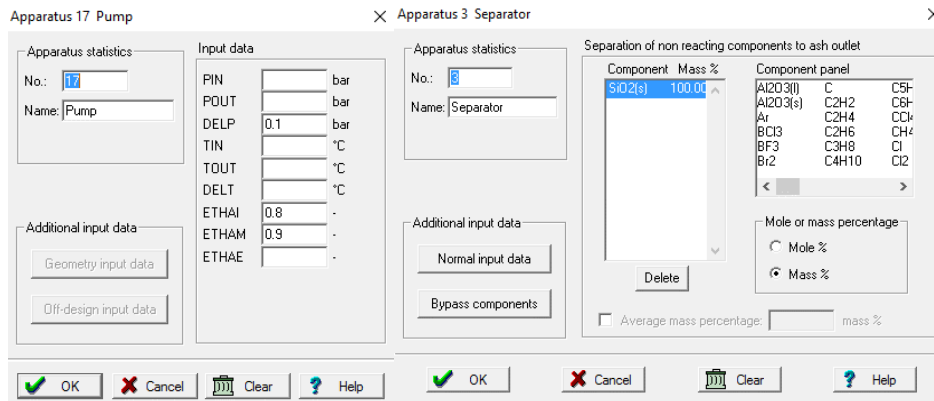
Fig.9 – Condizioni di lavoro modellate in Cycle Tempo del ciclone FIL.001 e delle pompe e ventilatori
