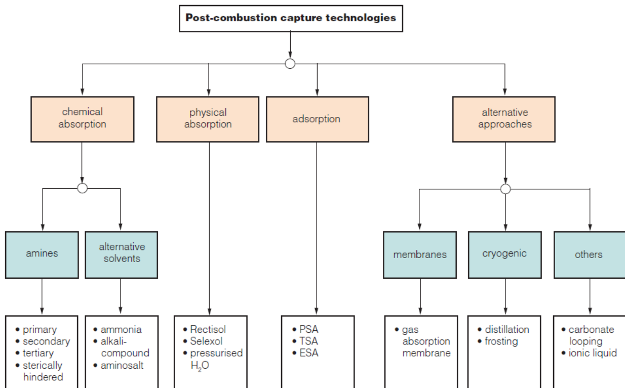
Figura 5. Alternative tecnologie per la separazione in post-combustione [2]
