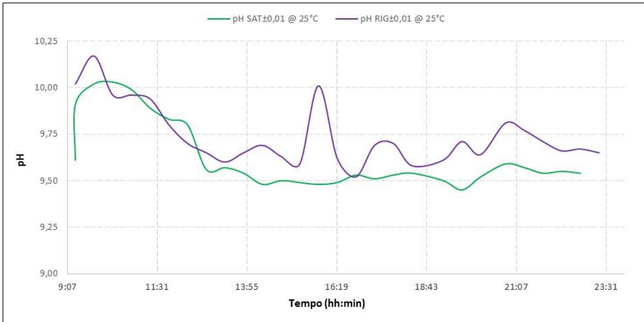
Figura 43. Andamento del pH durante il test per l'ammina esausta e per l'ammina rigenerata (14/07/2016)
