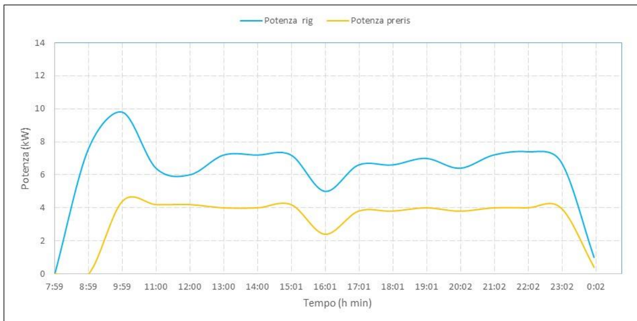
Figura 38. Consumi elettrici dell'unità di rigenerazione e del sistema di preriscaldamento delle ammine (Test del 14/07/2016)
