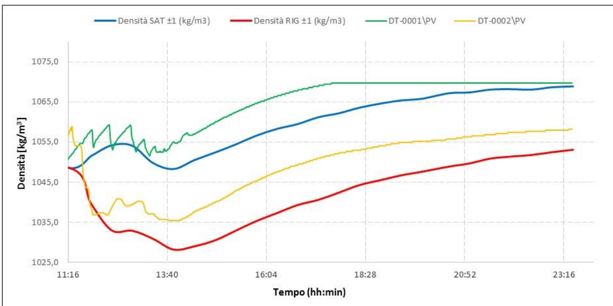
Figura 33. Confronto fra valori di densità misurati dai densimetri in linea e dal densimetro da laboratorio (Test del 05/05/2016)
