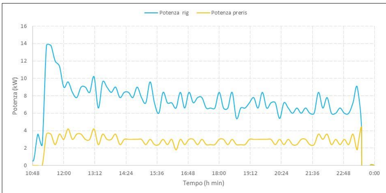
Figura 30. Consumi elettrici dell'unità di rigenerazione e del sistema di pre-riscaldamento delle ammine (Test del 05/05/2016)
