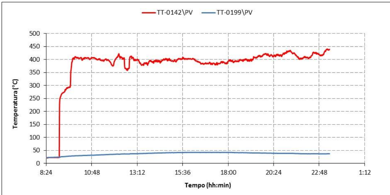
Figura 54. Temperature dei fumi in ingresso e in uscita dallo scambiatore gas/acqua (01/09/2016)
