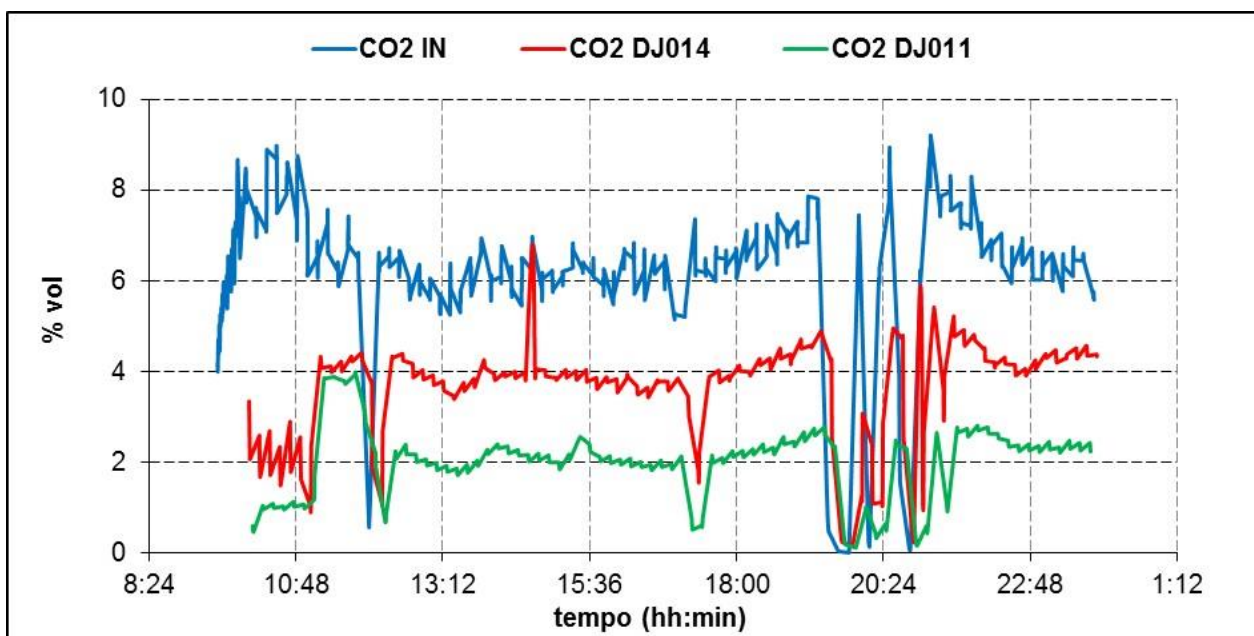
Figura 37. Sezione di cattura: concentrazione di CO 2 (Test del 14/07/2016)
