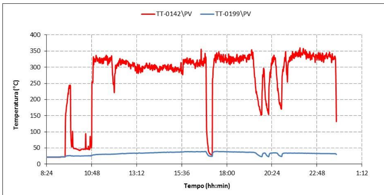
Figura 45. Temperature dei fumi in ingresso e in uscita dallo scambiatore gas/acqua (14/07/2016)
