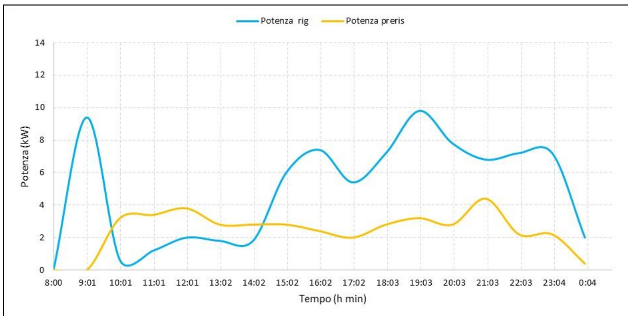
Figura 22. Consumi elettrici dell'unità di rigenerazione e del sistema di pre-riscaldamento delle ammine (Test del 21/04/2016)
