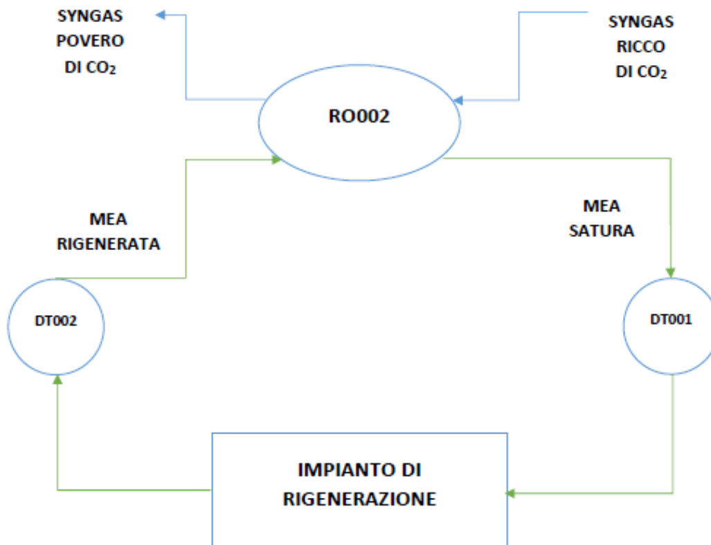
Figura 9. Circuito assorbimento/rigenerazione del 24 Marzo 2016
