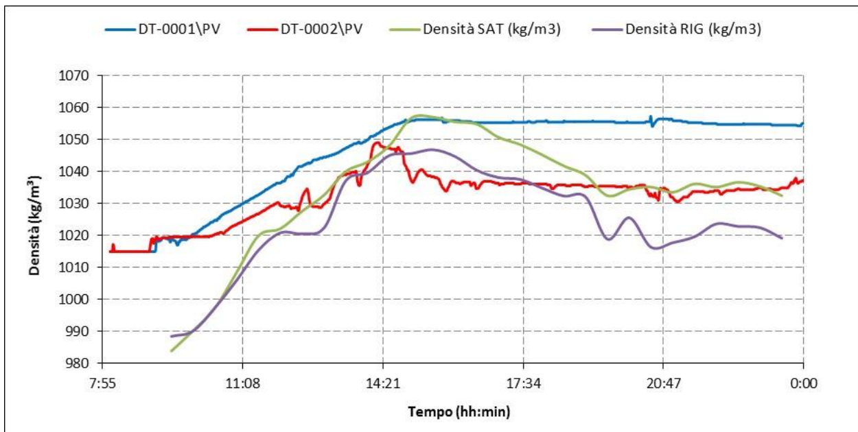
Figura 17. Confronto fra valori di densità misurati dai densimetri in linea e dal densimetro da laboratorio (Test del 24/03/2016)
