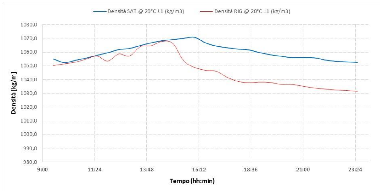
Figura 23. Andamento della densità rilevate con DENSITY METER DMA35 durante il test per l'ammina esausta e per l'ammina rigenerata (Test del 21/04/2016)
