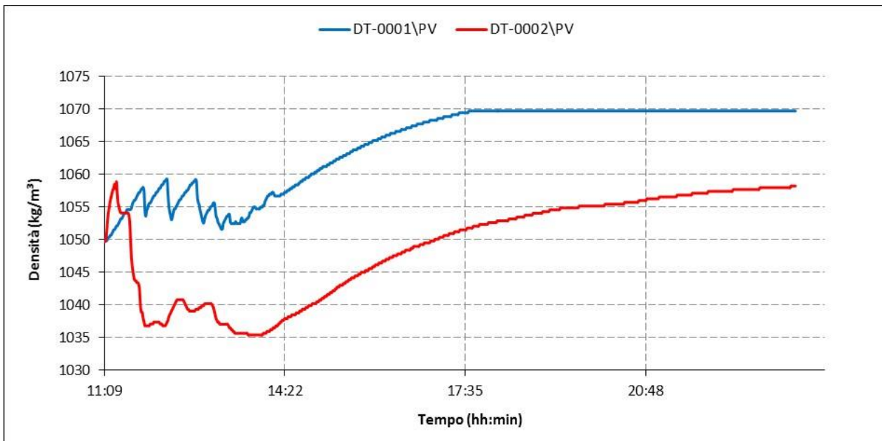
Figura 32. Andamento delle densità durante il test per l'ammina esausta e per l'ammina rigenerata rilevata mediante DT001 e DT002 (Test del 05/05/2016)
