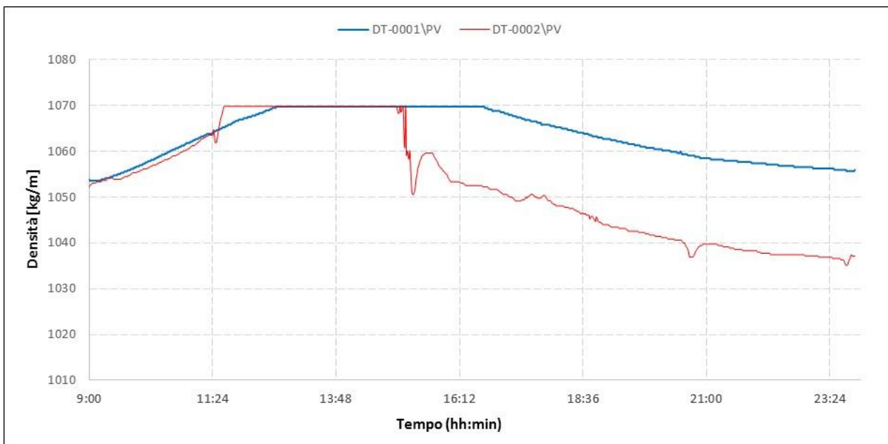
Figura 24. Andamento della densità durante il test per l'ammina esausta e per l'ammina rigenerata rilevata mediante DT001 e DT002 (Test del 21/04/2016)
