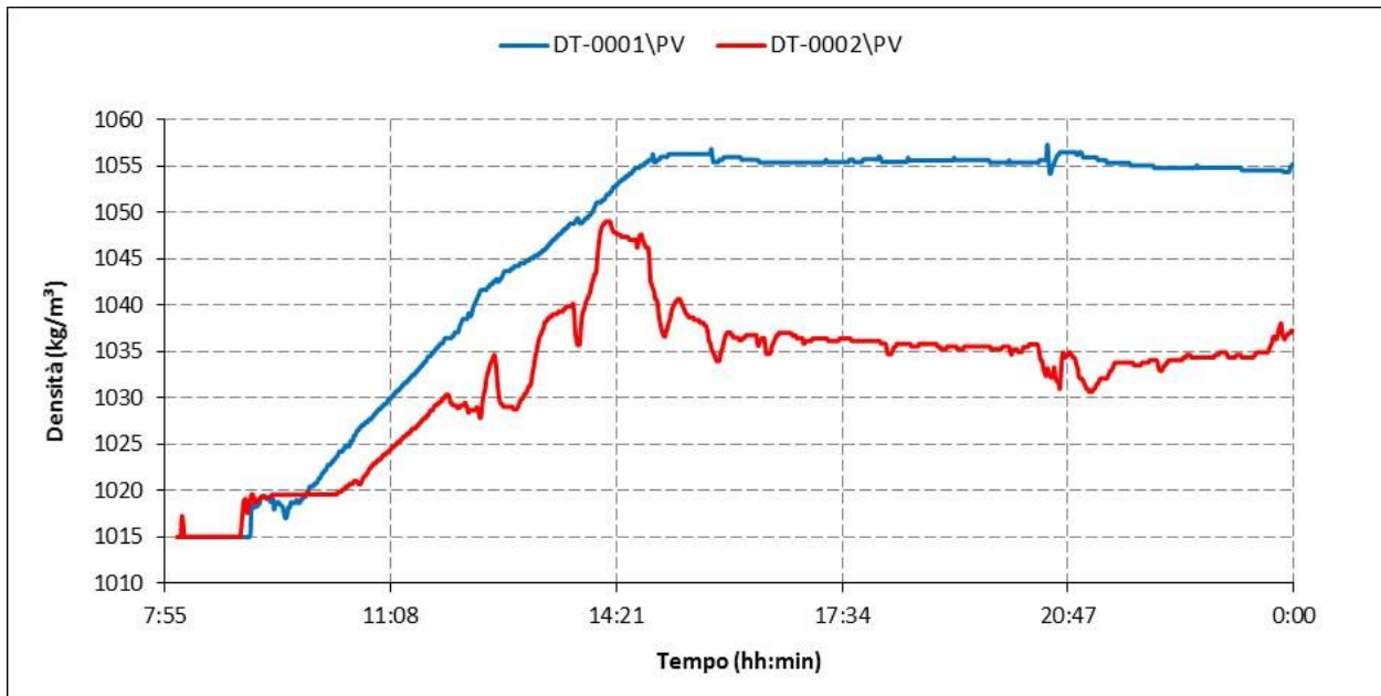
Figura 16. Andamento della densità durante il test per l'ammina esausta e per l'ammina rigenerata rilevata mediante DT001 e DT002 (Test del 24/03/2016)
