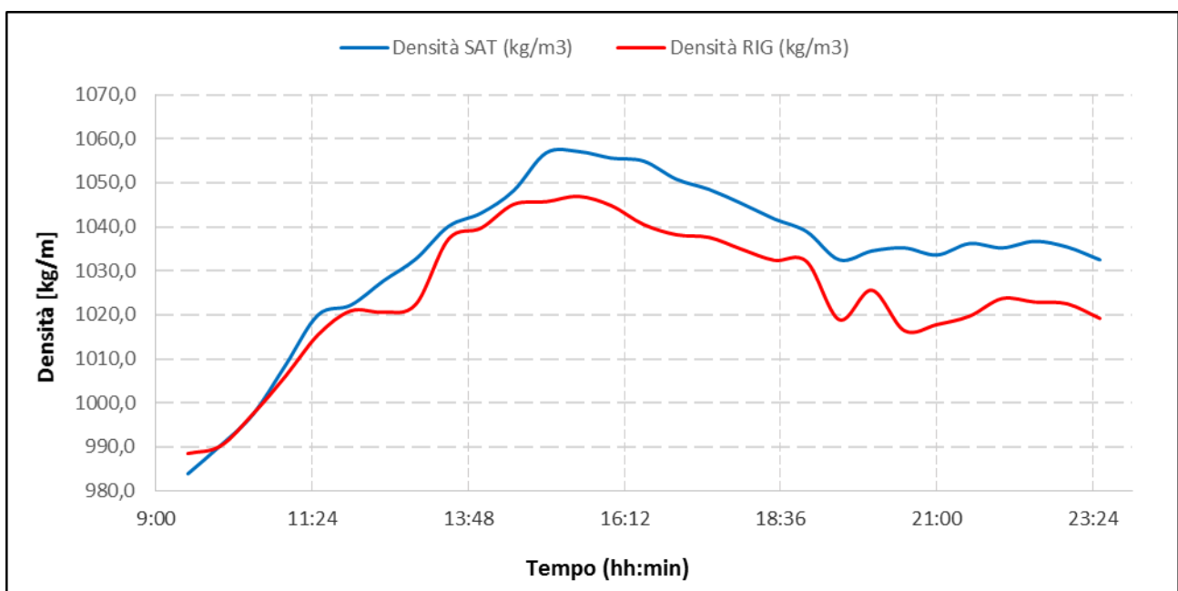
Figura 15. Andamento della densità rilevate con DENSITY METER DMA35 durante il test per l'ammina esausta e per l'ammina rigenerata (Test del 24/03/2016)
