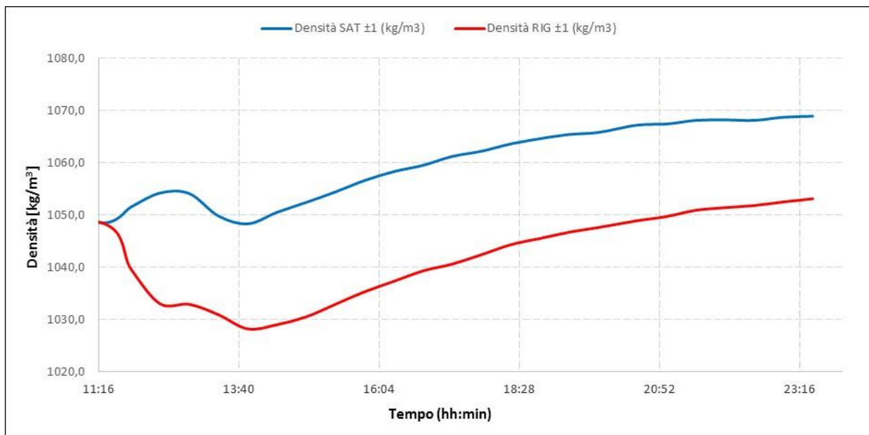
Figura 31. Andamento delle densità, rilevate con DENSITY METER DMA35, durante il test per l'ammina esausta e per l'ammina rigenerata (Test del 05/05/2016)
