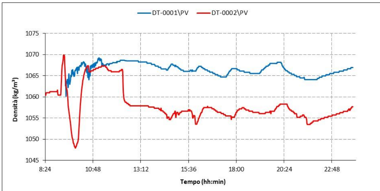
Figura 40. Andamento delle densità durante il test per l'ammina esausta e per l'ammina rigenerata rilevata mediante DT001 e DT002 (Test del 14/07/2016)
