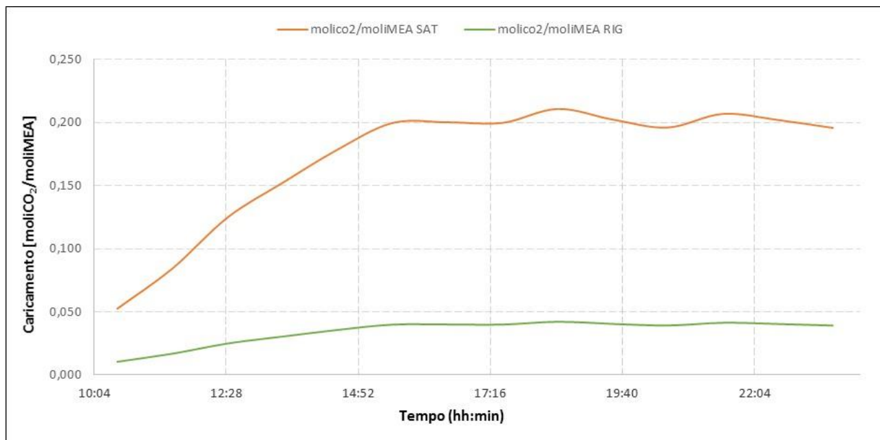
Figura 20. Andamento del caricamento durante il test per l'ammina esausta e per l'ammina rigenerata (Test del 24/03/2016)
