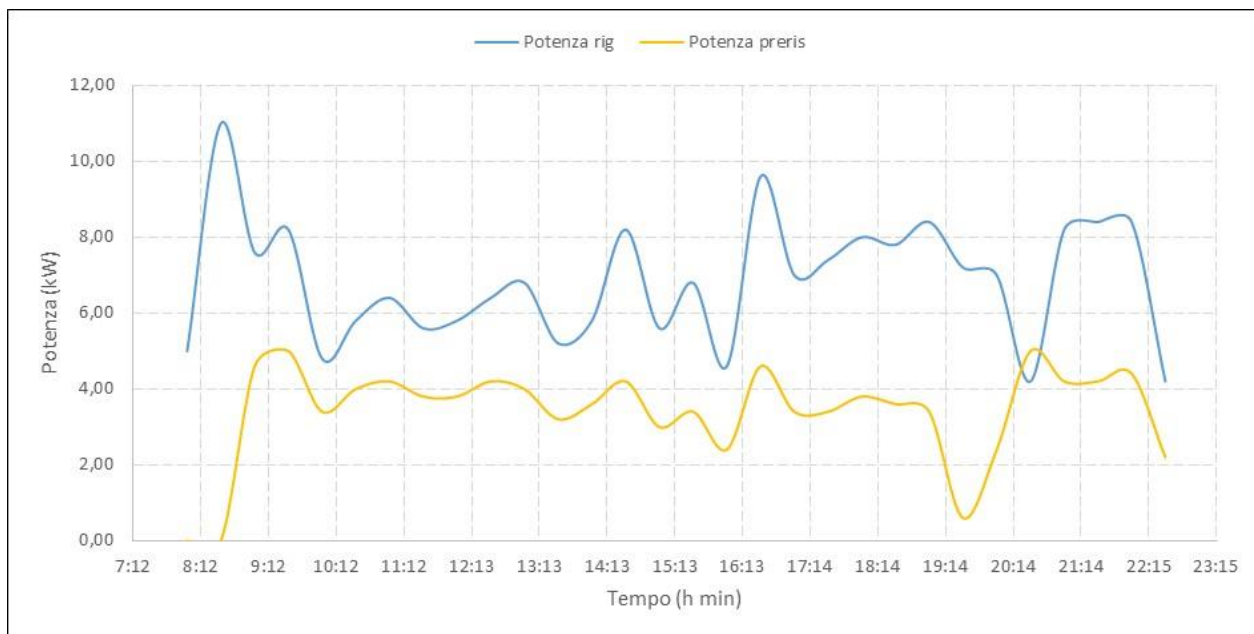
Figura 47. Consumi elettrici dell'unità di rigenerazione e del sistema di preriscaldamento delle ammine (Test del 01/09/2016)
