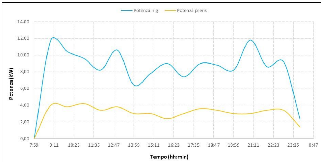
Figura 14. Consumi elettrici dell'unità di rigenerazione e del sistema di pre-riscaldamento delle ammine (Test del 24/03/2016)
