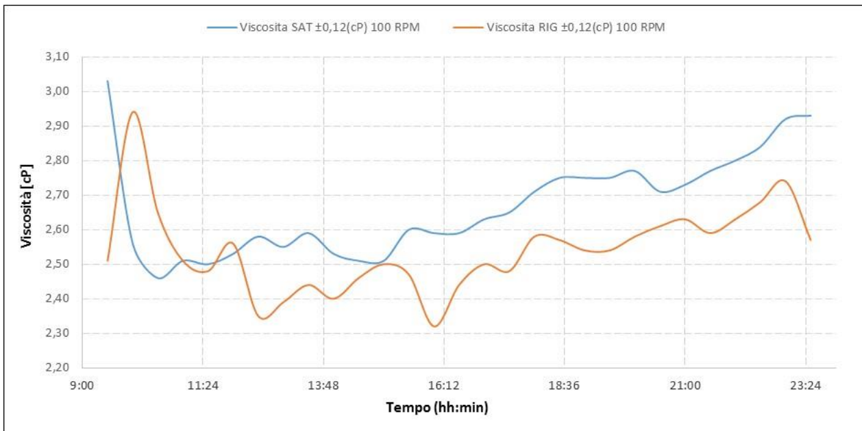
Figura 18. Andamento della viscosità (100 RPM) durante il test per l'ammina esausta e per l'ammina rigenerata (Test del 24/03/2016)
