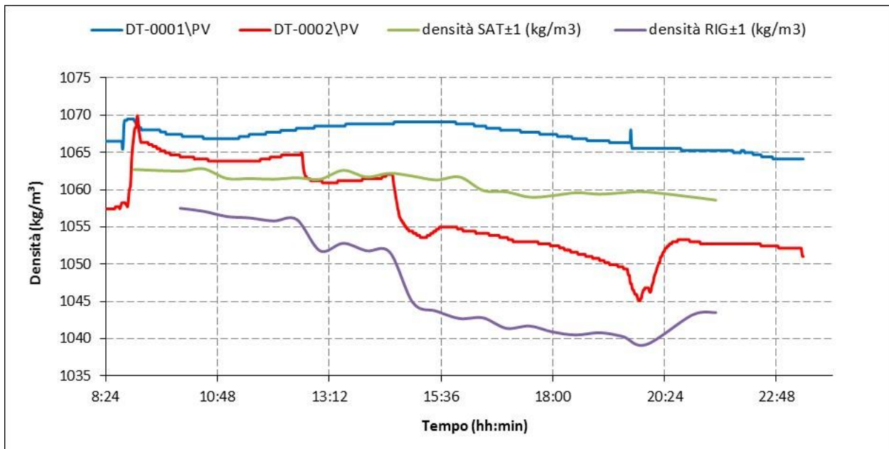
Figura 50. Confronto fra valori di densità misurati dai densimetri in linea e dal densimetro da laboratorio (Test del 01/09/2016)
