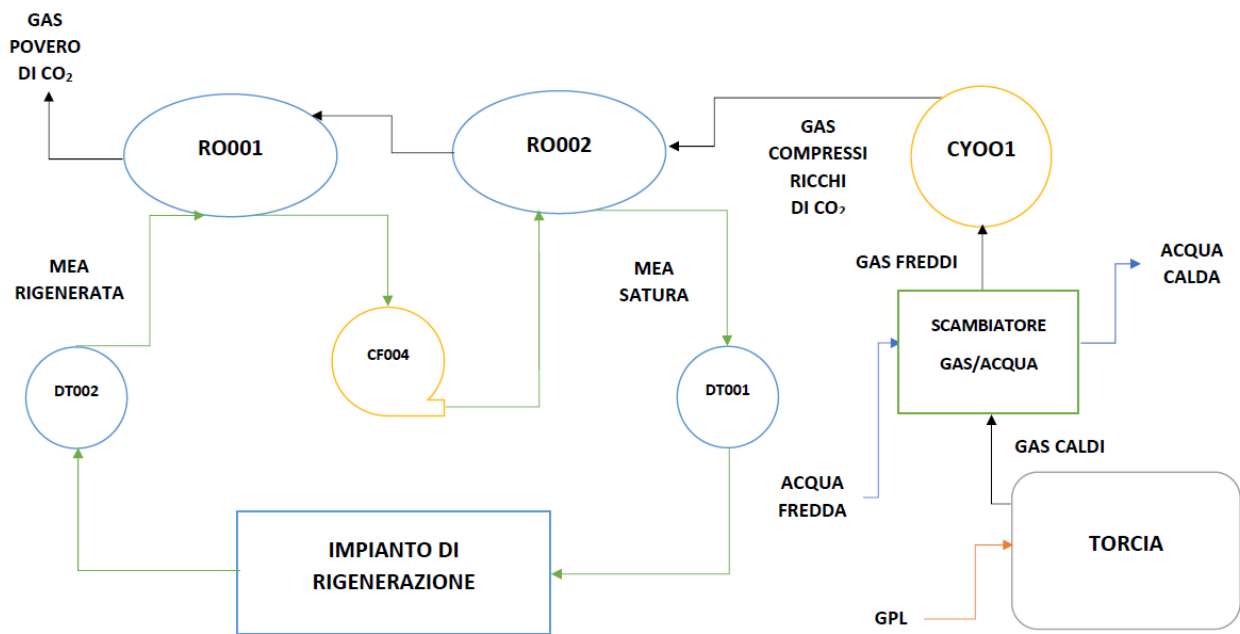
Figura 11. Circuito di adduzione gas da torcia e assorbimento/rigenerazione (test del 14/07/2016)
