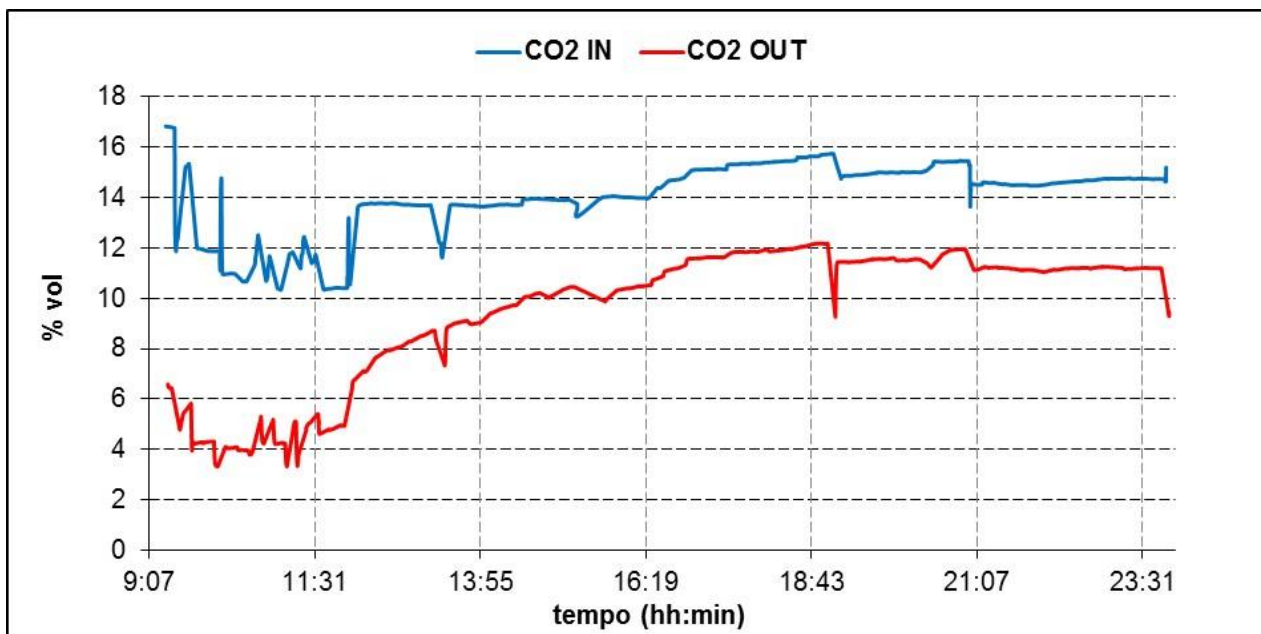
Figura 13. Sezione di cattura: concentrazione di CO 2 (Test del 24/03/2016)
