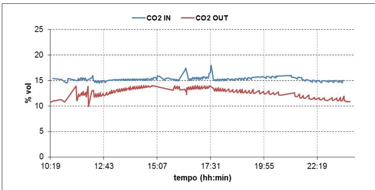
Figura 21. Sezione di cattura: concentrazione di CO 2 (Test del 21/04/2016)
