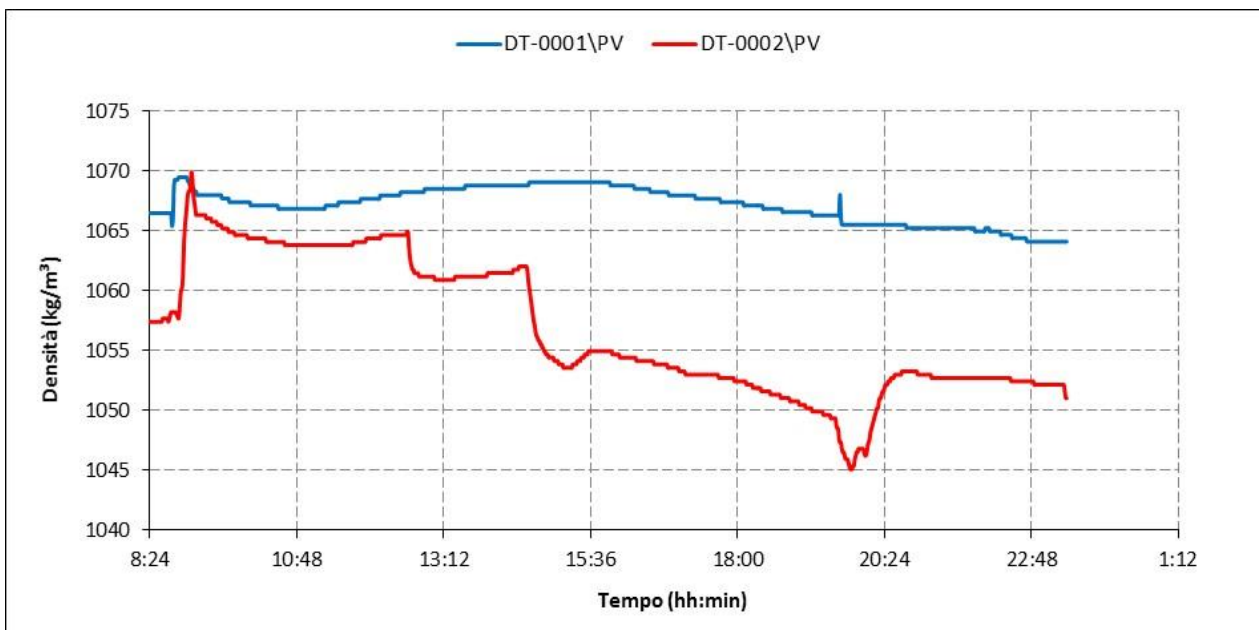
Figura 49. Andamento delle densità durante il test per l'ammina esausta e per l'ammina rigenerata rilevata mediante DT001 e DT002 (Test del 01/09/2016)
