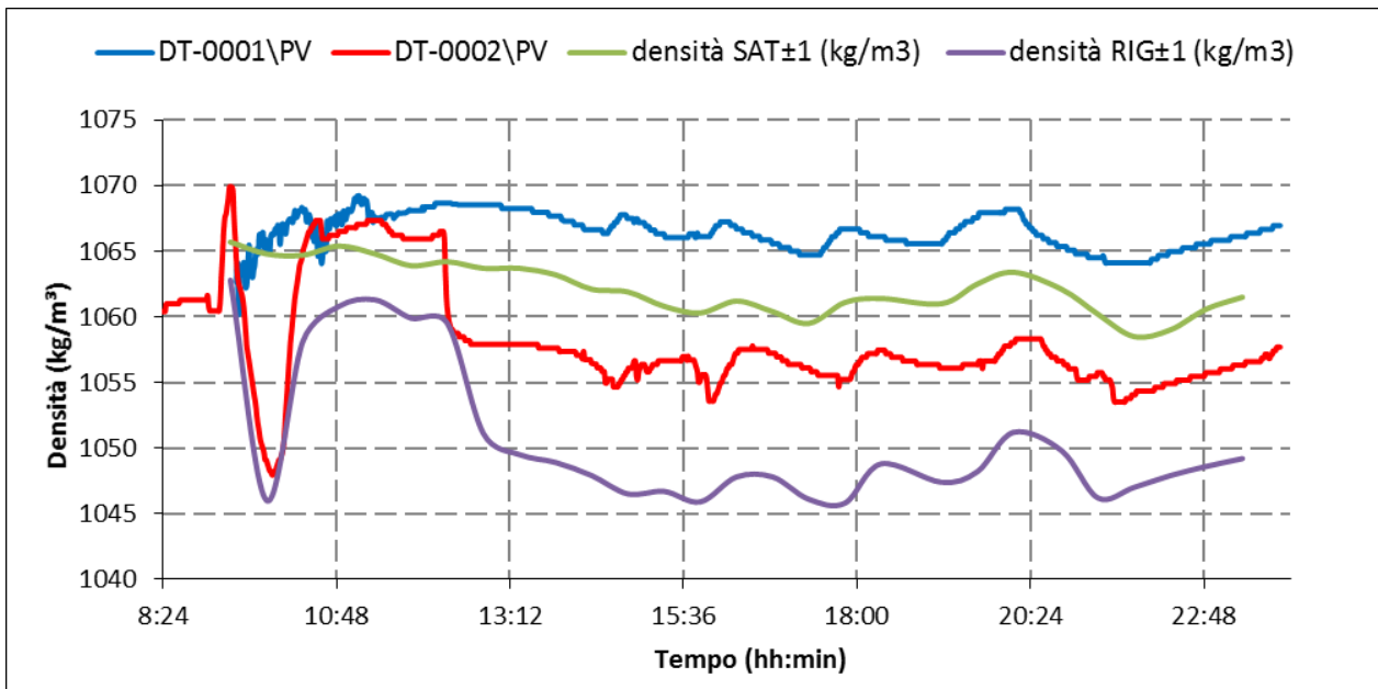
Figura 41. Confronto fra valori di densità misurati dai densimetri in linea e dal densimetro da laboratorio (Test del 14/07/2016)
