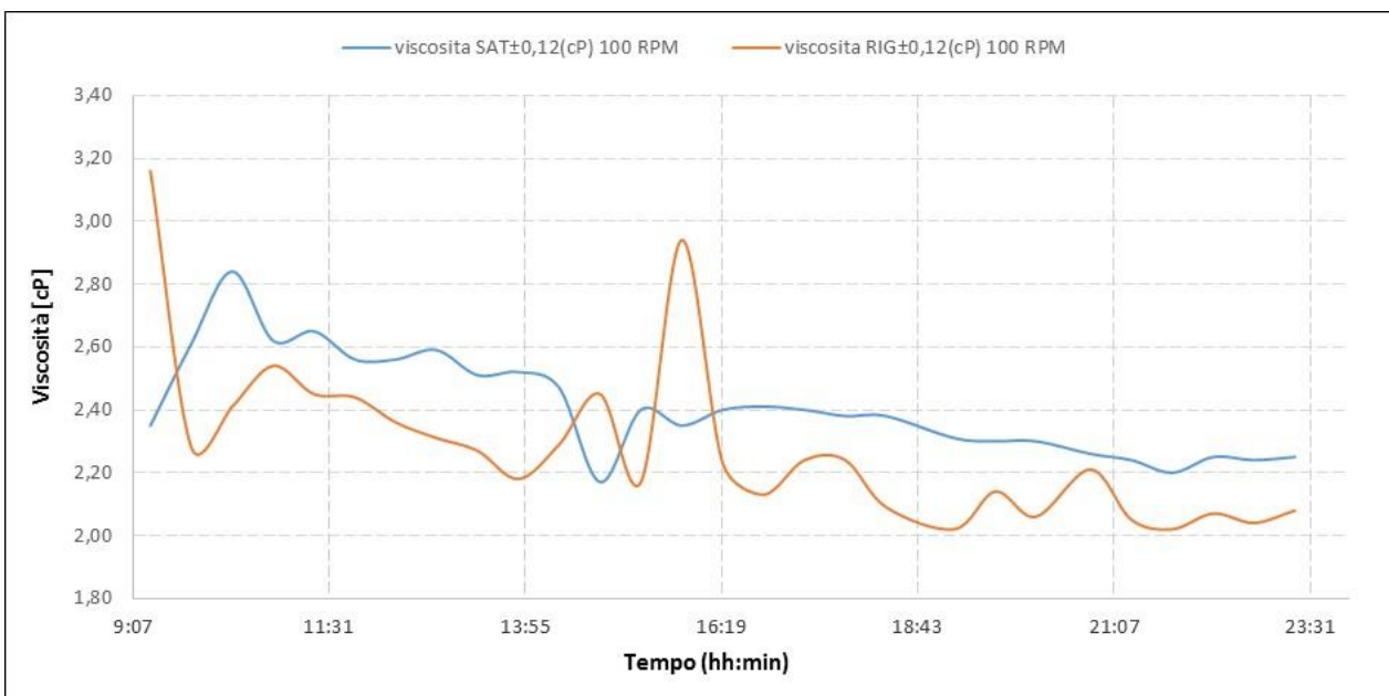
Figura 42. Andamento della viscosità (100 RPM) durante il test per l'ammina esausta e per l'ammina rigenerata (Test del 14/07/2016)
