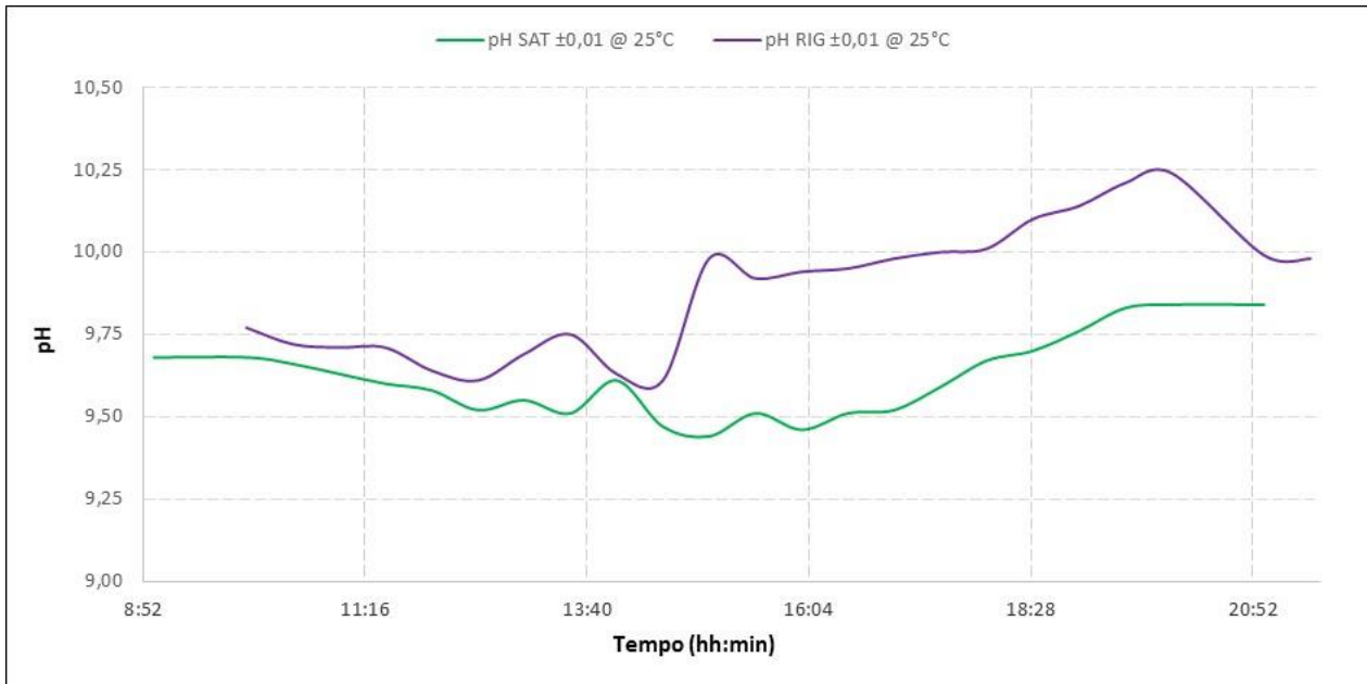
Figura 52. Andamento del pH durante il test per l'ammina esausta e per l'ammina rigenerata (01/09/2016)
