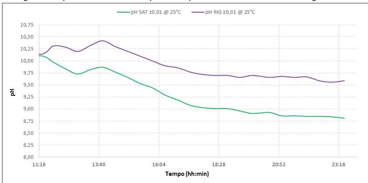
Figura 35. Andamento del pH durante il test per l'ammina esausta e per l'ammina rigenerata (Test del 05/05/2016)
