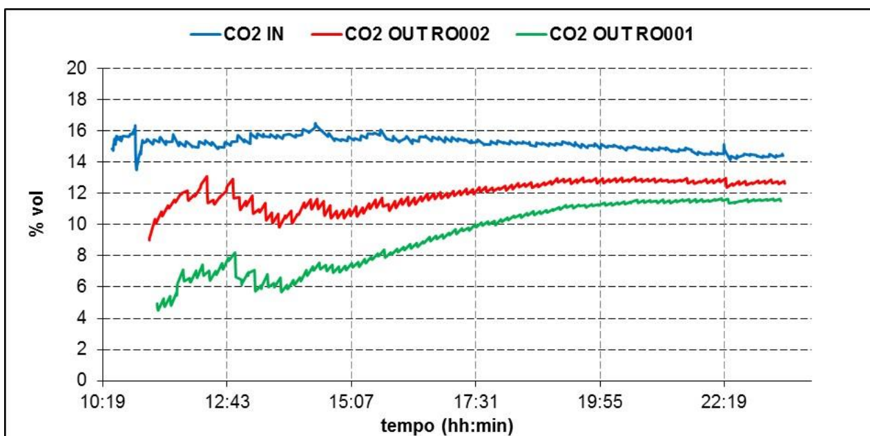
Figura 29. Sezione di cattura: concentrazione di CO 2 (Test del 05/05/2016)
