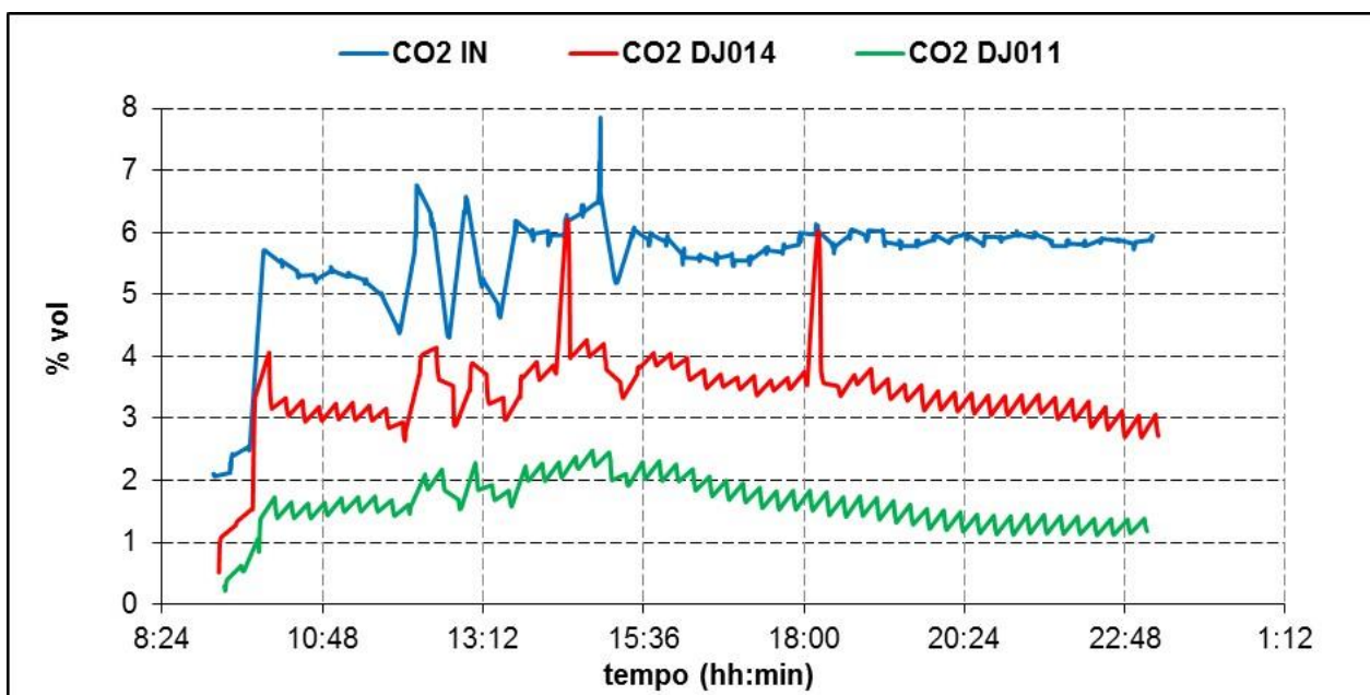
Figura 46. Sezione di cattura: concentrazione di CO 2 (Test del 01/09/2016)
