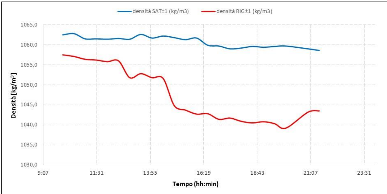
Figura 48. Andamento delle densità, rilevate con DENSITY METER DMA35, durante il test per l'ammina esausta e per l'ammina rigenerata (Test del 01/09/2016)
