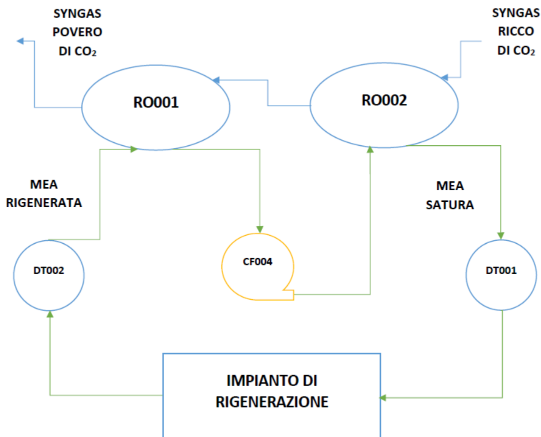
Figura 10. Circuito di assorbimento/rigenerazione utilizzato nei test del 21/04/2016 e 05/05/2016
