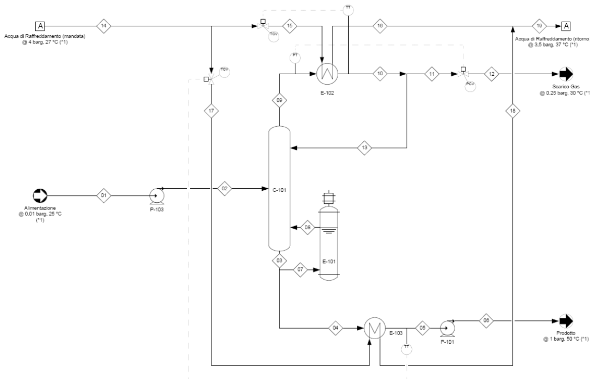
Figura 8. Schema semplificato del sistema di rigenerazione delle ammine
