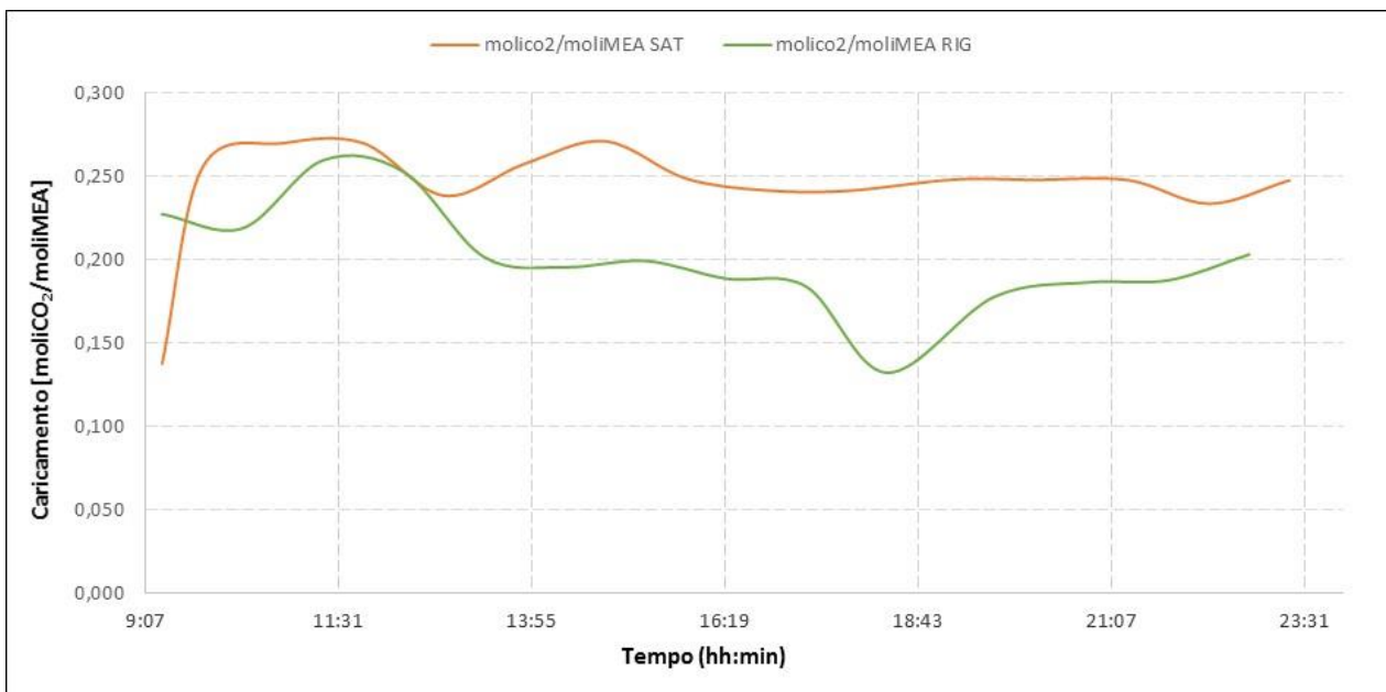
Figura 44. Andamento del caricamento durante il test per l'ammina esausta e per l'ammina rigenerata (14/07/2016)
