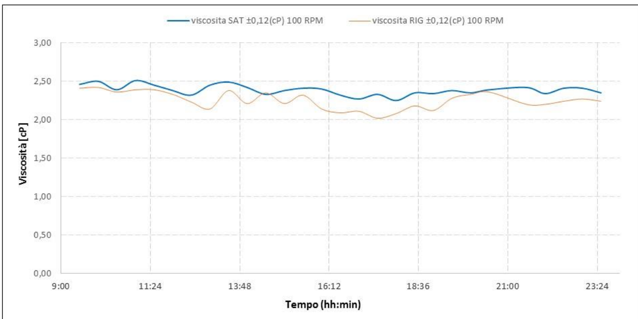
Figura 26. Andamento della viscosità (100 RPM) durante il test per l'ammina esausta e per l'ammina rigenerata (Test del 21/04/2016)
