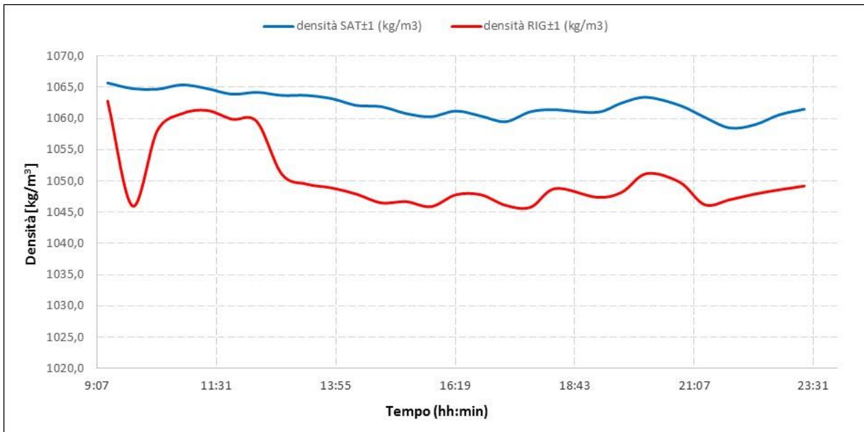
Figura 39. Andamento delle densità, rilevate con DENSITY METER DMA35, durante il test per l'ammina esausta e per l'ammina rigenerata (Test del 14/07/2016)
