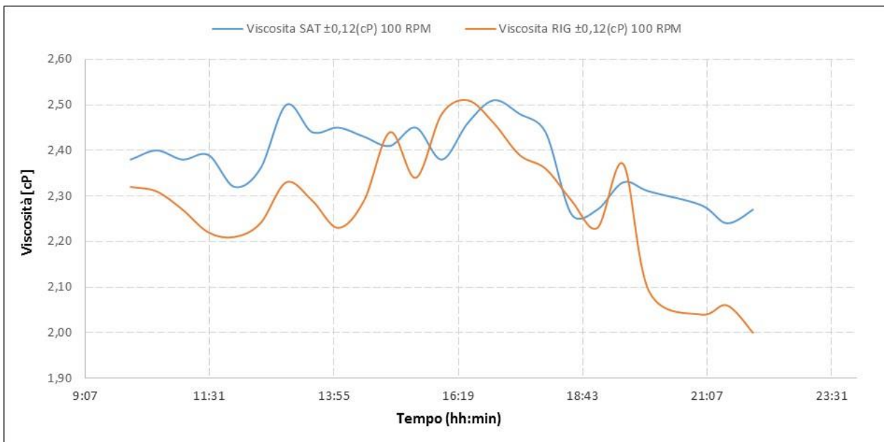
Figura 51. Andamento della viscosità (100 RPM) durante il test per l'ammina esausta e per l'ammina rigenerata (Test del 01/09/2016)
