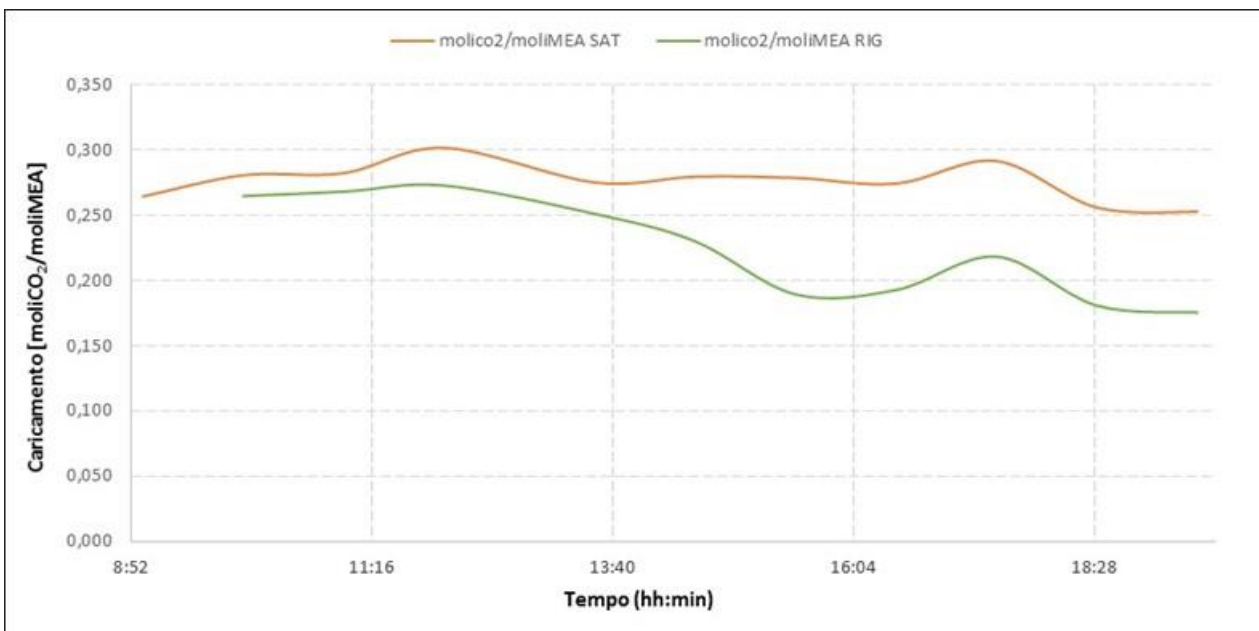
Figura 53. Andamento del caricamento durante il test per l'ammina esausta e per l'ammina rigenerata (01/09/2016)
