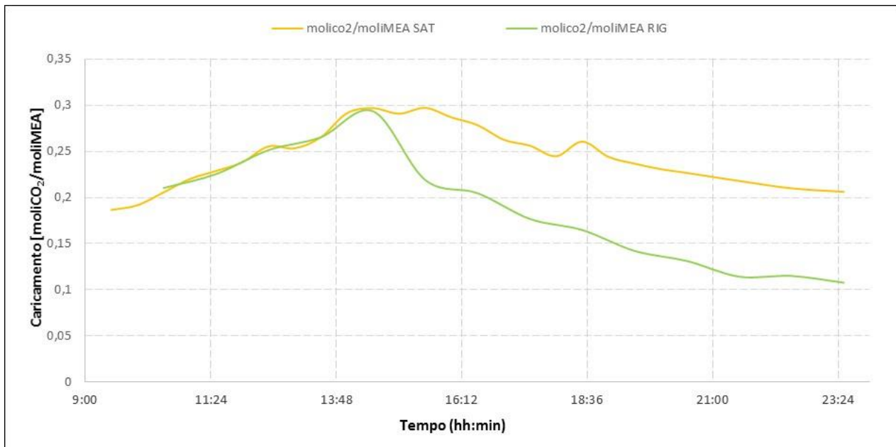
Figura 28. Andamento del caricamento durante il test per l'ammina esausta e per l'ammina rigenerata (Test del 21/04/2016)
