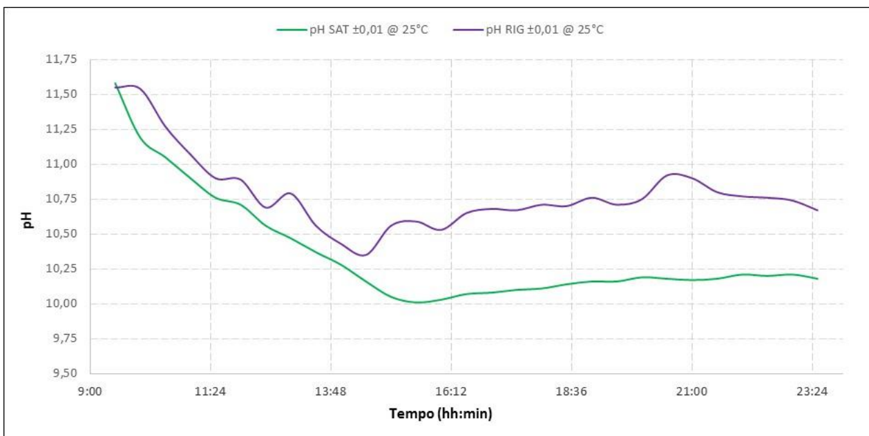
Figura 19. Andamento del pH durante il test per l'ammina esausta e per l'ammina rigenerata (Test del 24/03/2016)
