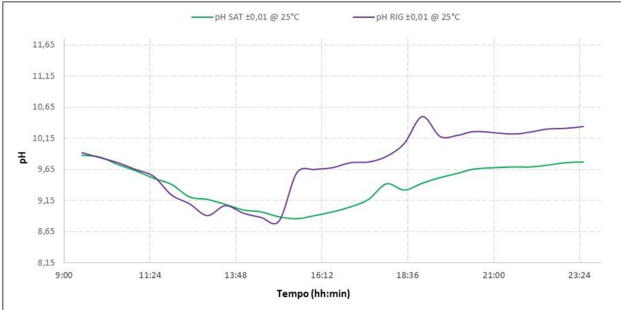
Figura 27. Andamento del pH durante il test per l'ammina esausta e per l'ammina rigenerata (Test del 21/04/2016)
