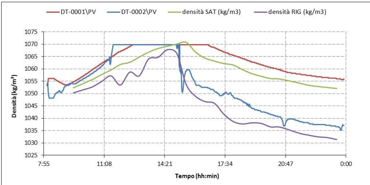
Figura 25. Confronto fra valori di densità misurati dai densimetri in linea e dal densimetro da laboratorio (Test del 21/04/2016)
