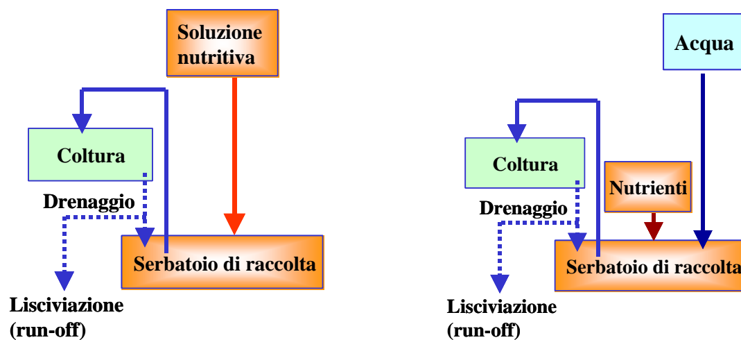
Figura 19 - Differenti sistemi di reintegro dei nutrienti nelle soluzioni riciccolanti dei sistemi a ciclo chiuso. A destra: opzione a conducibilità costante; a sinistra: opzione con concentrazione dei nutrienti costante.
