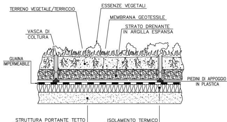
Figura 2 - Sistema di coltivazione su substrato
