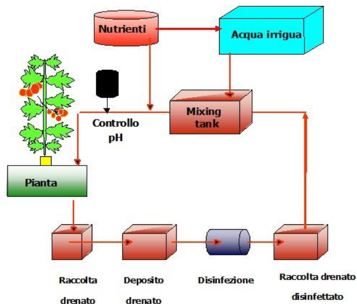
Figura 18 - Lay-out di un sistema idroponico avanzato
