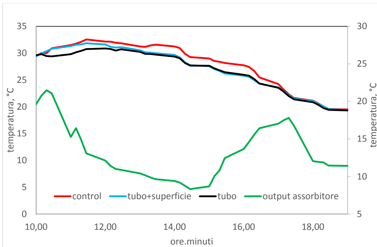
Figura 36: Temperature dell'aria in prossimità delle piante per zona non raffreddata (control), zona raffreddata con tubo posto in posizione centrale (tubo), zona raffreddata con tubo più superficie metallica (tubo+superficie), temperatura dell'acqua raffreddata in uscita dall'assorbitore (output assorbitore - asse dx).
