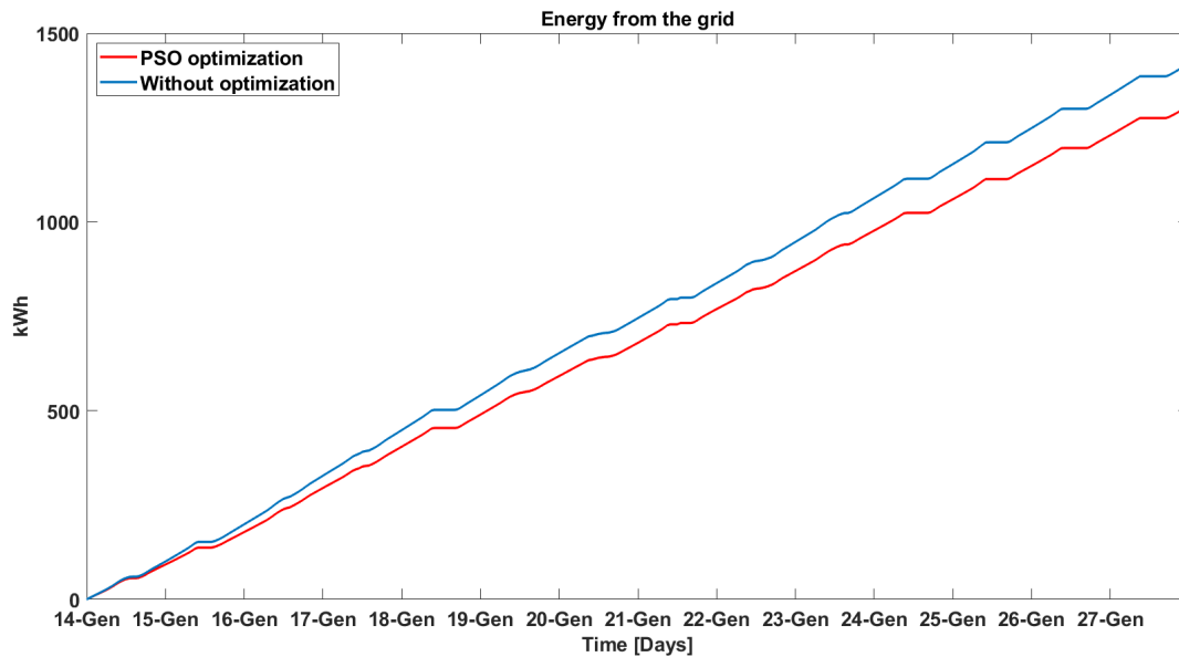
Figura 2-3 Energia prelevata dalla rete (energia elettrica consumata meno energia PV) nel periodo 14/01-27/01
