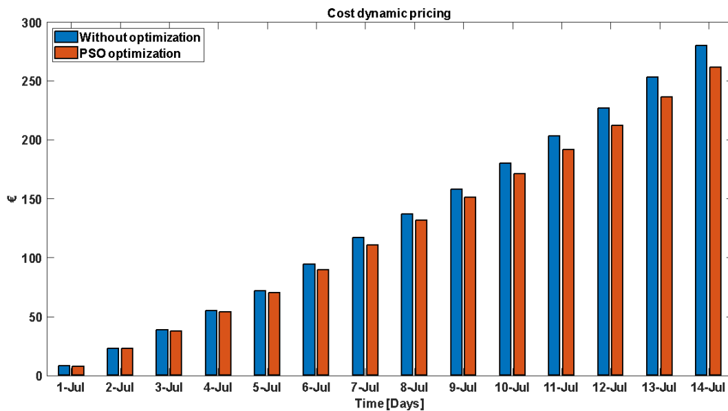
Figura 2-14 Media giornaliera del dynamic pricing con PV nel periodo 01/07-14/07
