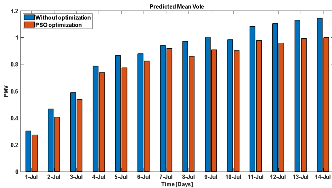
Figura 2-22 Media giornaliera del Predicted Mean Vote (PMV) nel periodo 01/07-14/07
