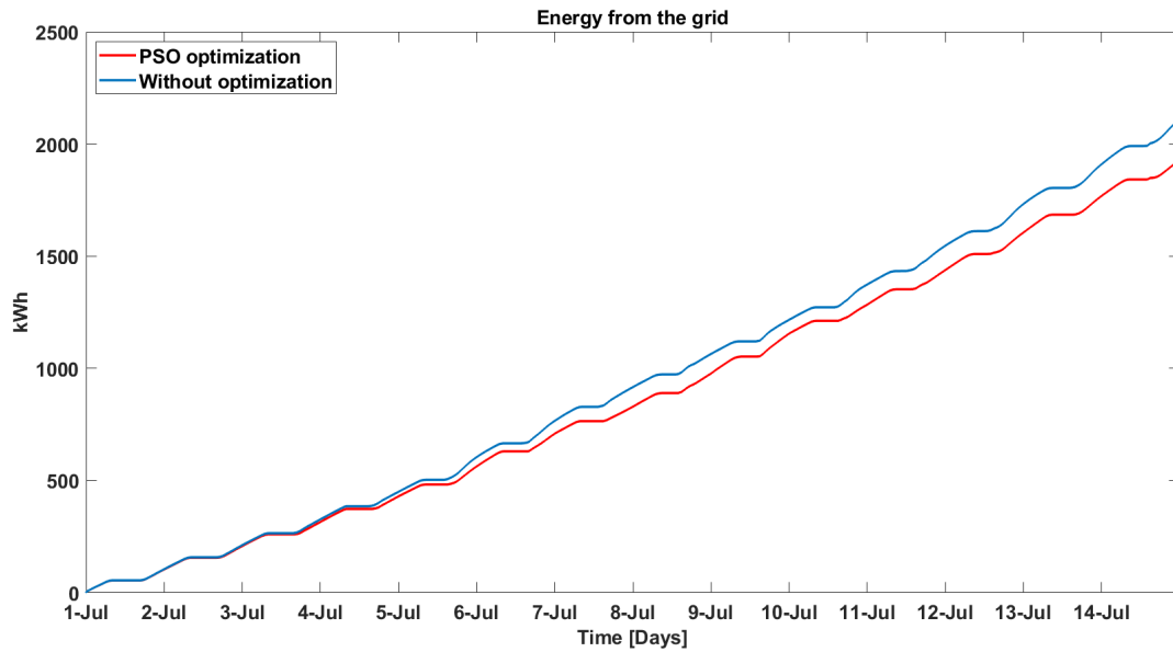
Figura 2-5 Energia prelevata dalla rete (energia elettrica consumata meno energia PV) nel periodo 01/07-14/07
