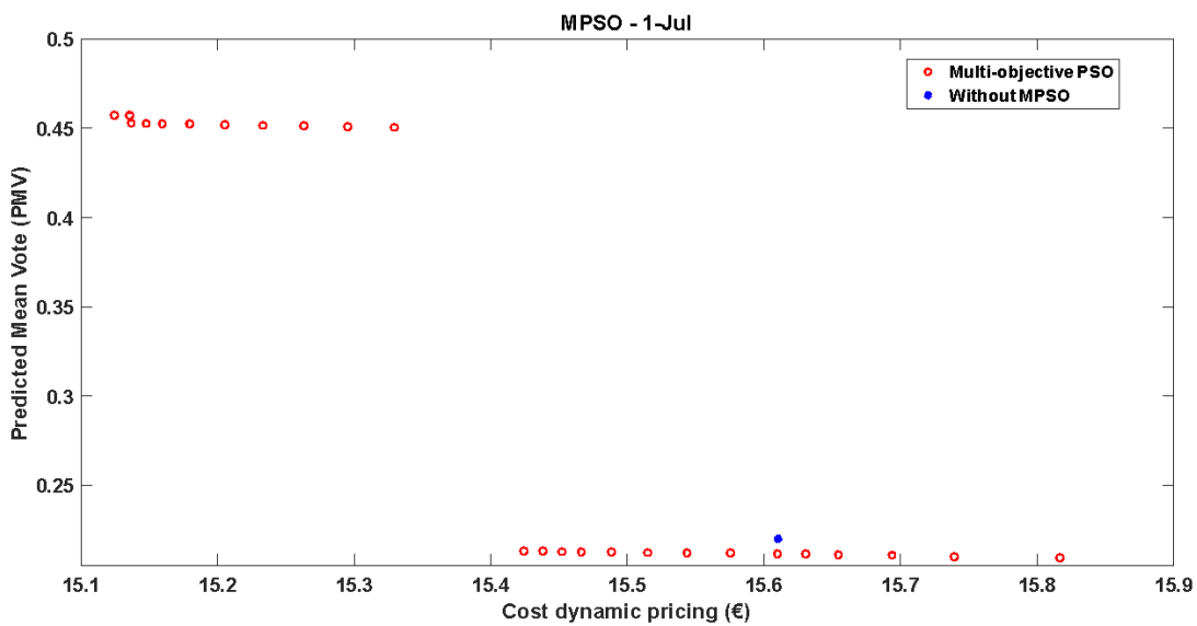
Figura 2-26 Punti non dominanti (in rosso) dell'algorithm MPSO considerando il PMV e la spesa energetica in termini di dynamic pricing, nella giornata 01/07
