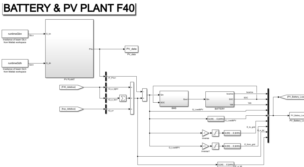
Figura 2-2 Schema a blocchi del sottosistema Batteria e Fotovoltaico
