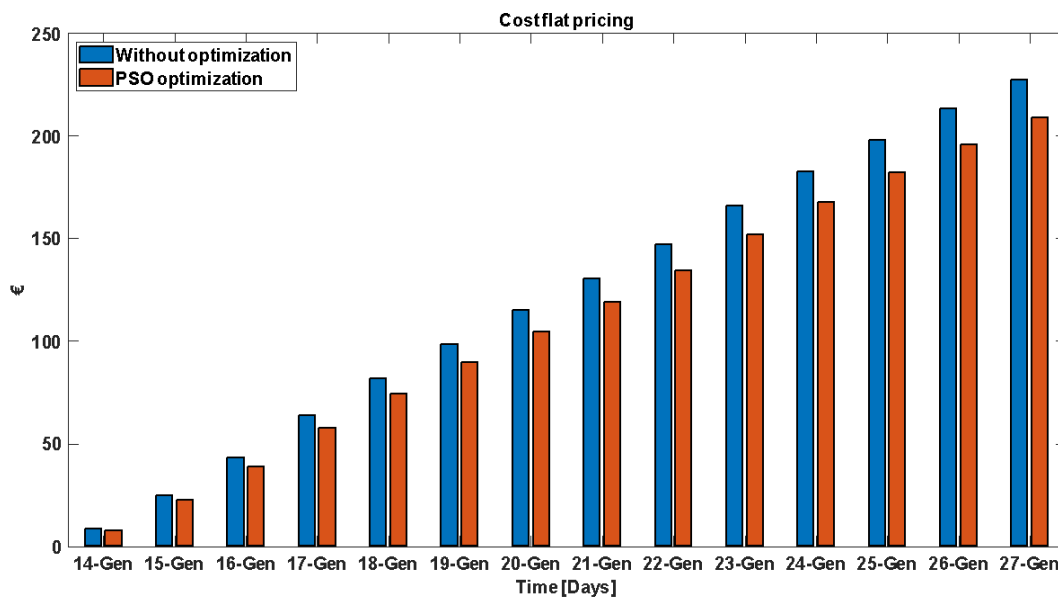
Figura 2-8 Media giornaliera del flat pricing con PV nel periodo 14/01-27/01
