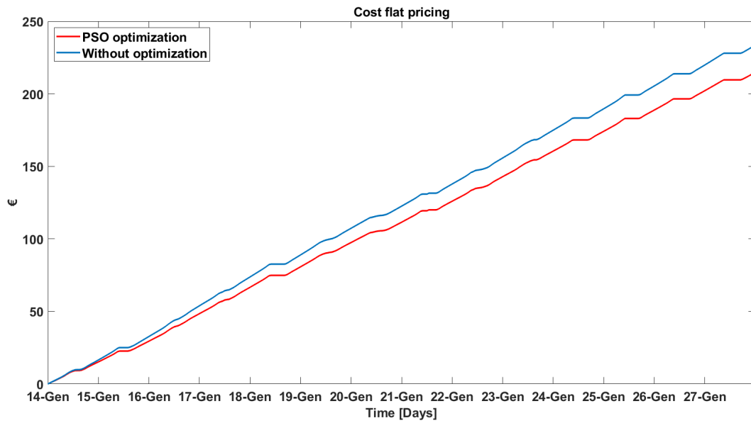
Figura 2-7 Flat pricing con PV nel periodo 14/01-27/01
