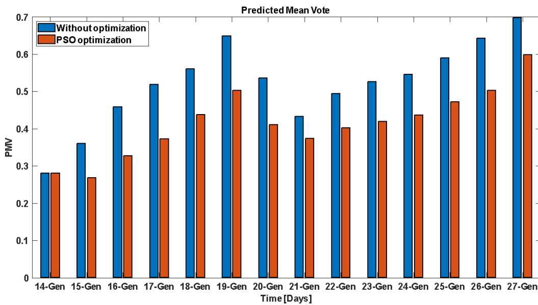
Figura 2-20 Media giornaliera del Predicted Mean Vote (PMV) nel periodo 14/01-27/01
