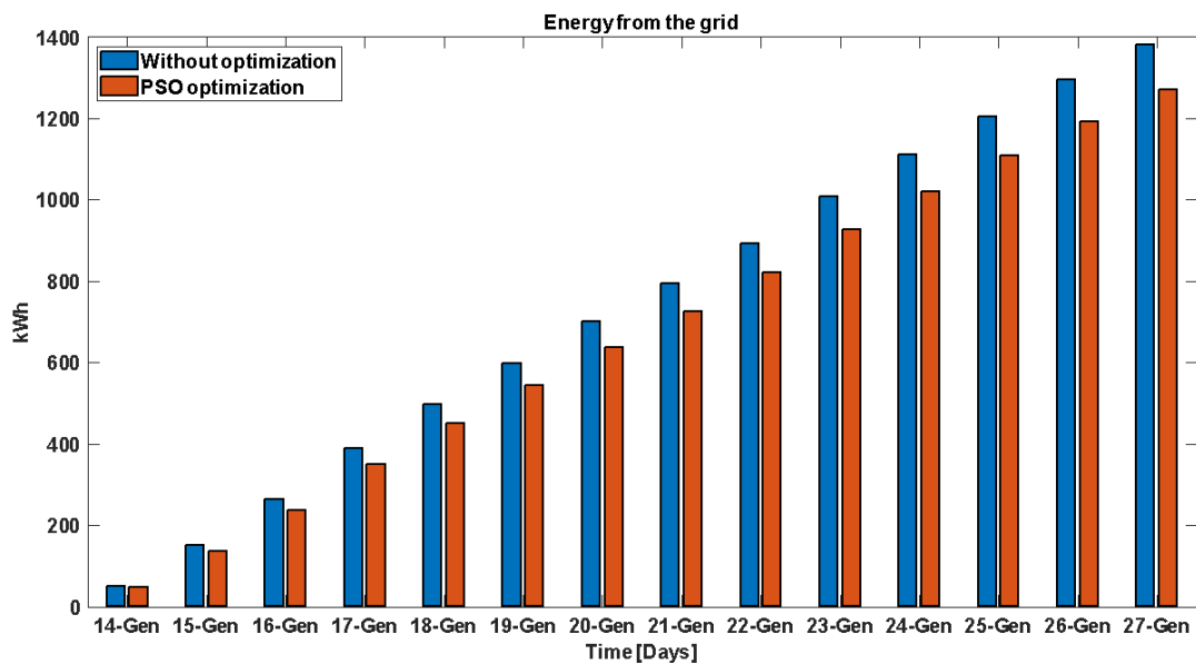
Figura 2-4 Media giornaliera dell'energia prelevata dalla rete (energia elettrica consumata meno energia PV) nel periodo 14/01-27/01
