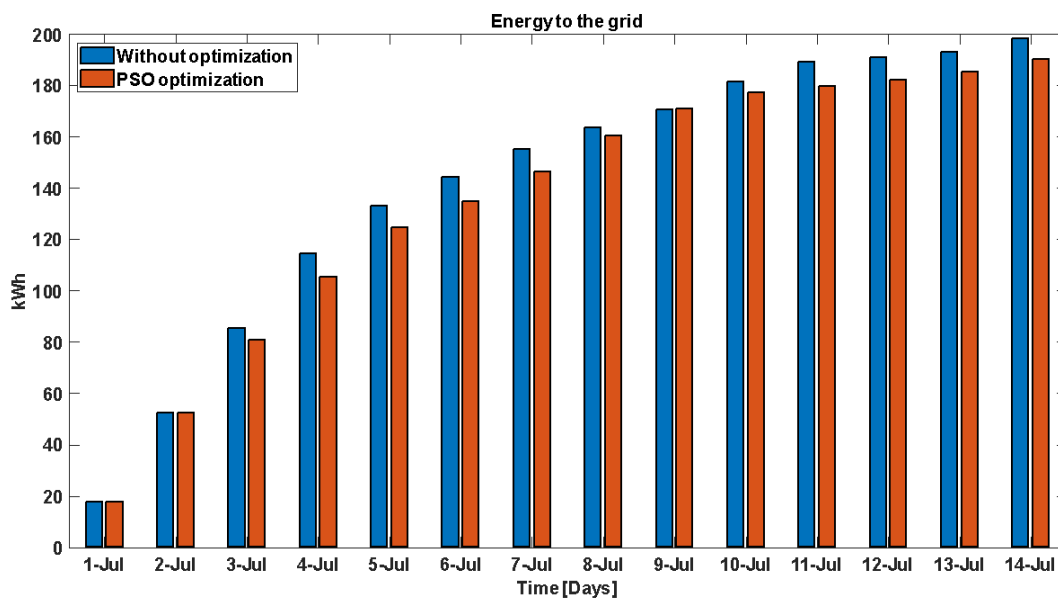
Figura 2-18 Media giornaliera dell'energia in eccesso reimmessa in rete considerando il PV nel periodo 01/07-14/01
