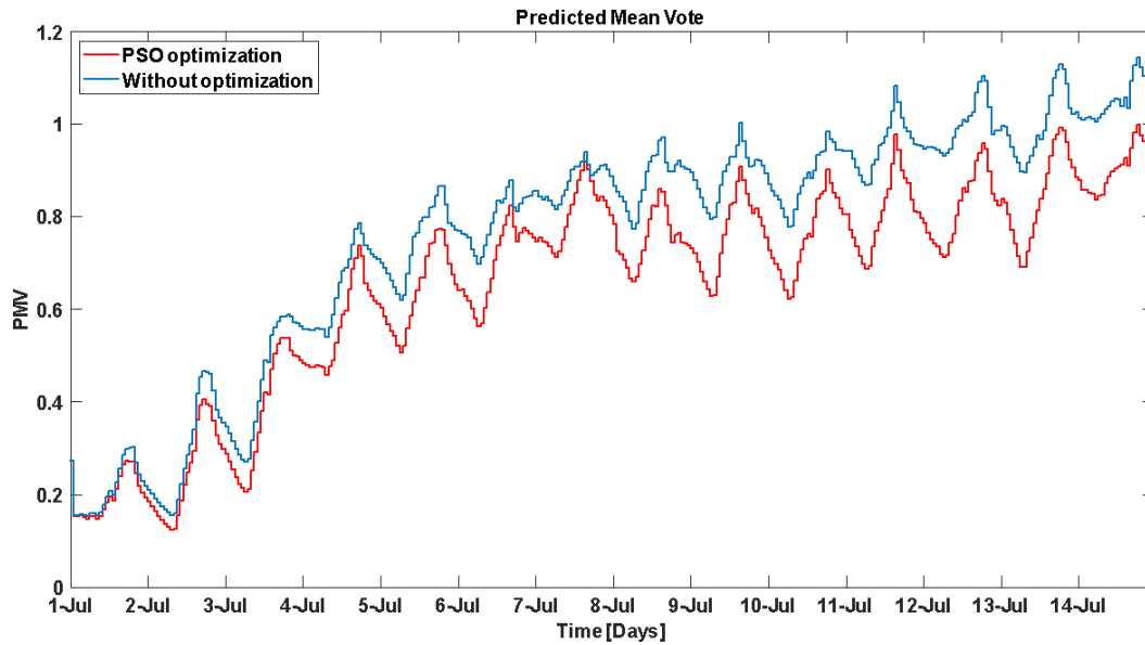
Figura 2-21 Predicted Mean Vote (PMV) nel periodo 01/07-01/07
