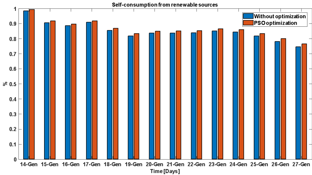
Figura 2-23 Percentuale di autoconsumo da fonti rinnovabili (PV) nel periodo 14/01-27/01
