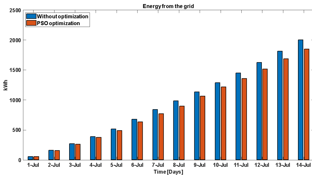
Figura 2-6 Media giornaliera dell'energia prelevata dalla rete (energia elettrica consumata meno energia PV) nel periodo 01/07-14/07
