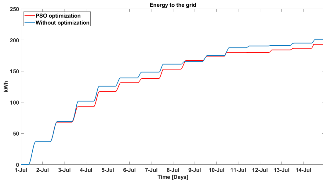
Figura 2-17 Energia in eccesso reimmessa in rete considerando il PV nel periodo 01/07-14/07
