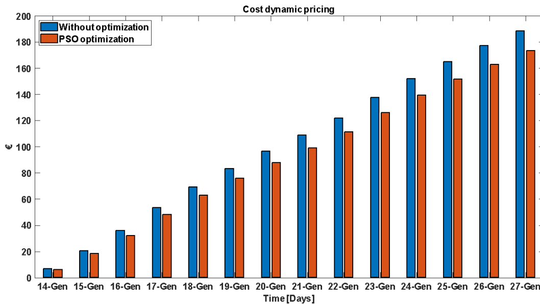
Figura 2-12 Media giornaliera del dynamic pricing con PV nel periodo 14/01-27/01
