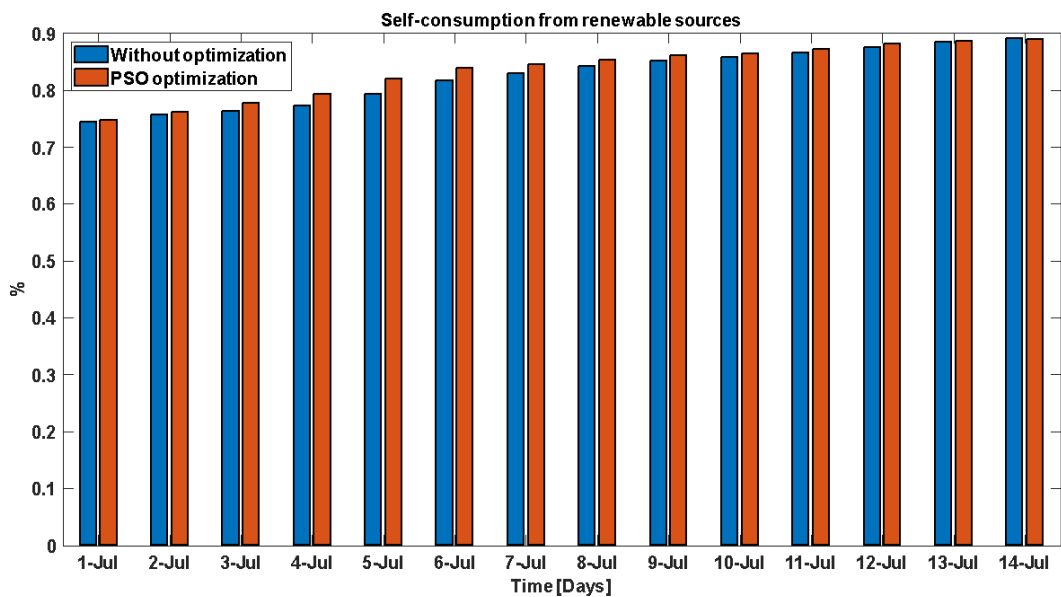
Figura 2-24 Percentuale di autoconsumo da fonti rinnovabili (PV) nel periodo 01/07-14/07
