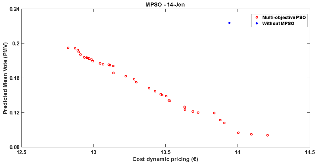
Figura 2-25 Punti non dominanti (in rosso) dell'algorithm MPSO considerando il PMV e la spesa energetica in termini di dynamic pricing, nella giornata 14/01
