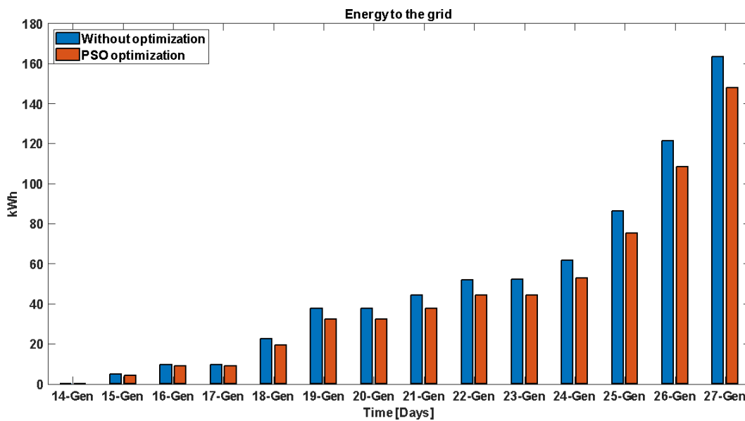
Figura 2-16 Media giornaliera dell'energia in eccesso reimessa in rete considerando il PV nel periodo 14/01-27/01
