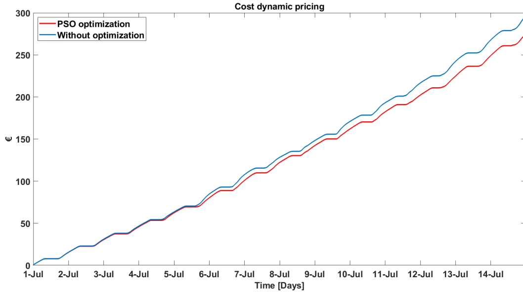
Figura 2-13 Dynamic pricing con PV nel periodo 01/07-14/07
