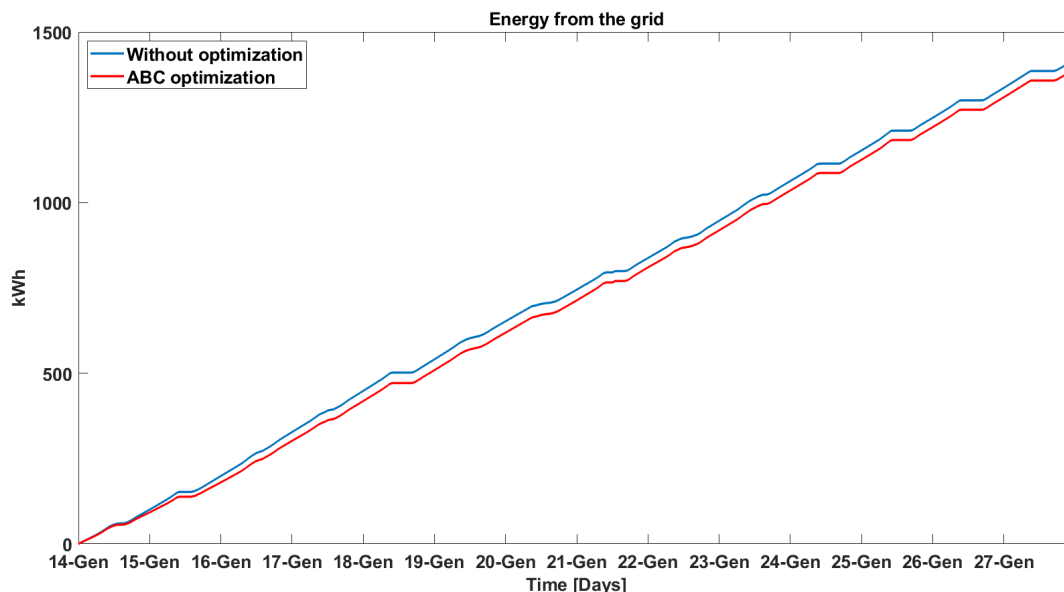
Figura 2-27 Ottimizzazione dell’energia prelevata dalla rete (energia elettrica consumata meno energia PV) nel periodo 14/01-27/01 utilizzando l’algoritmo ABC
