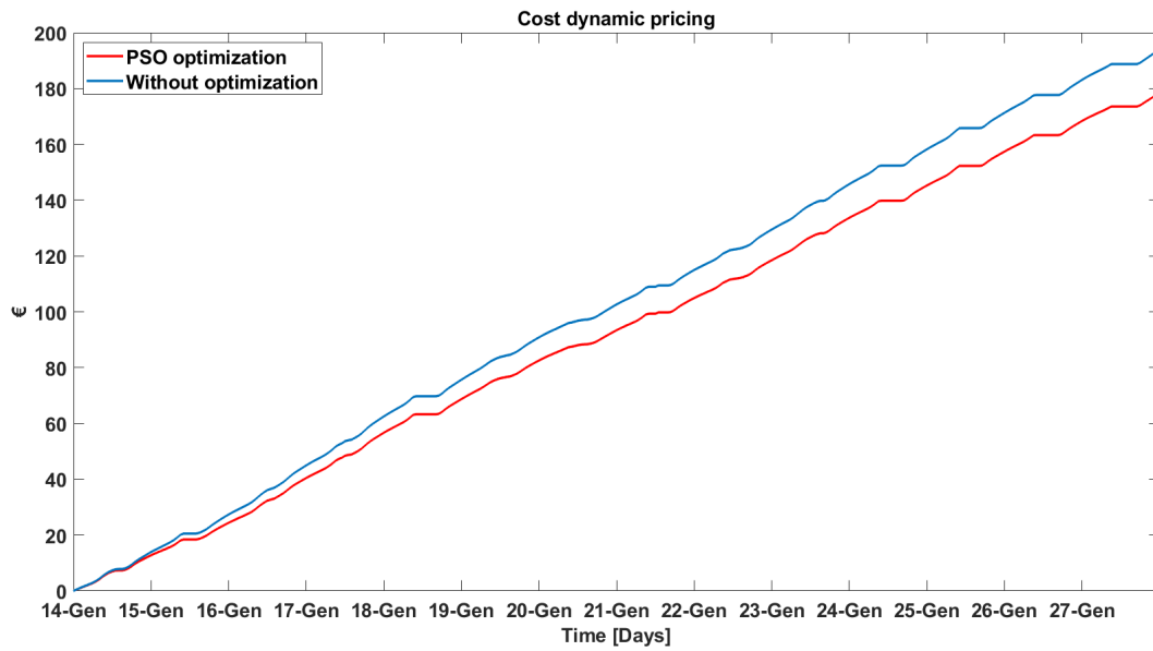
Figura 2-11 Dynamic pricing con PV nel periodo 14/01-27/01
