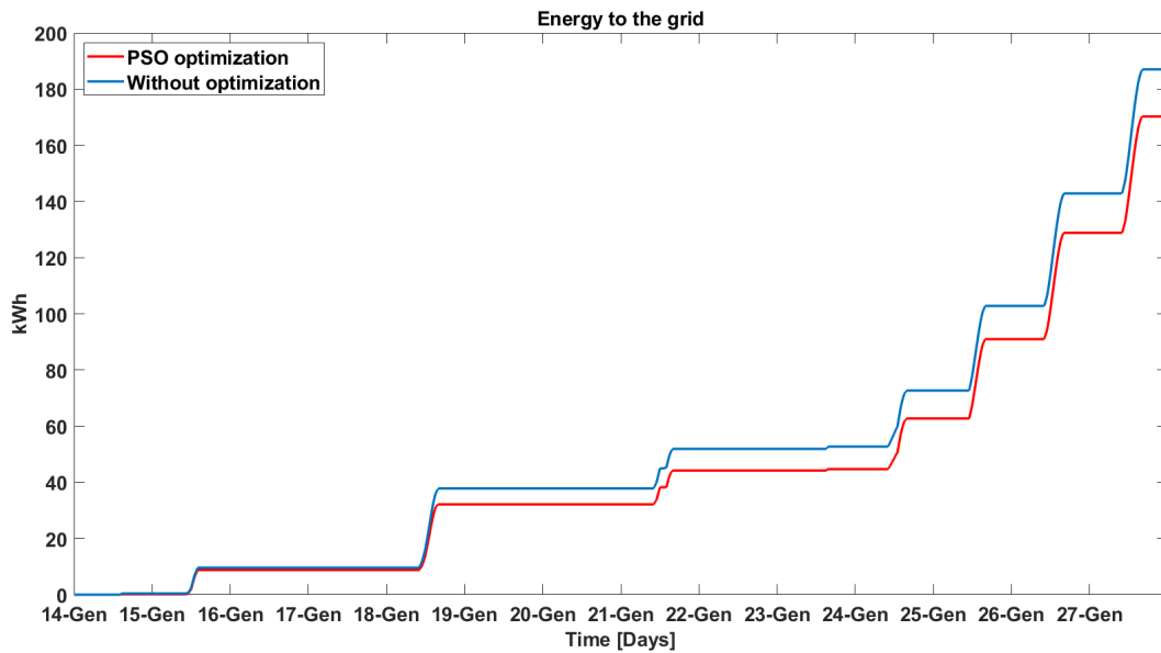
Figura 2-15 Energia in eccesso reimessa in rete considerando il PV nel periodo 14/01-27/01
