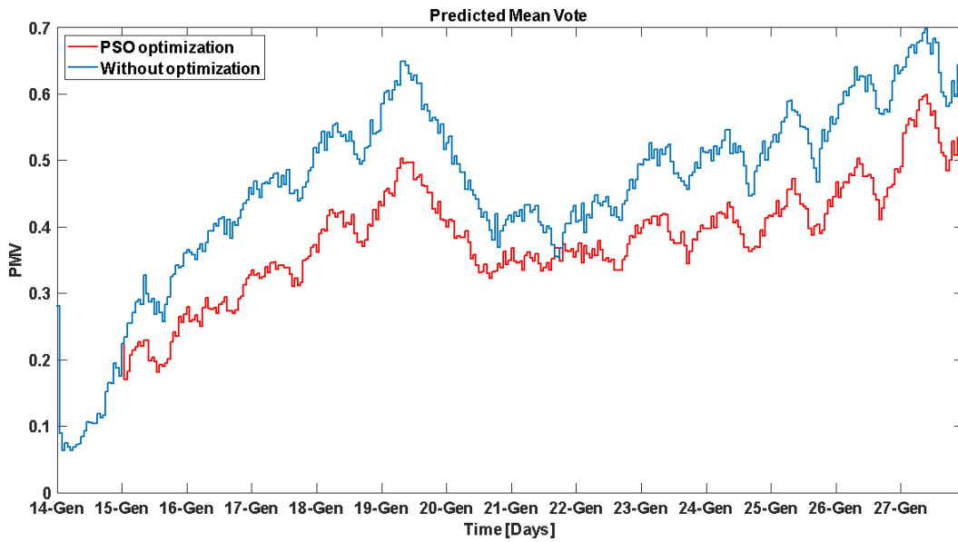
Figura 2-19 Predicted Mean Vote (PMV) nel periodo 14/01-27/01
