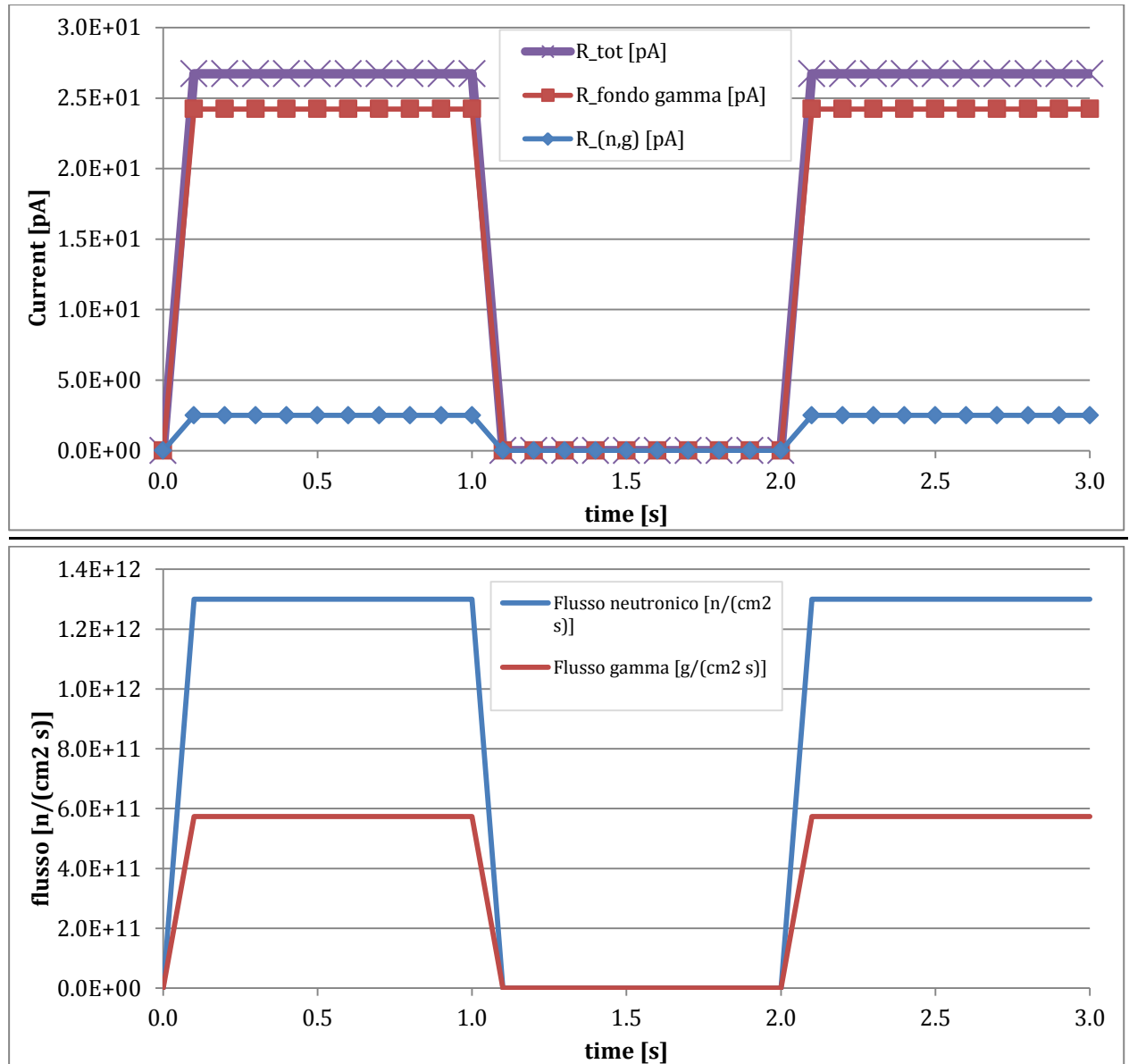
Figura 12 - Risposta dinamica del SPND alimentato con 190 Pt (platino in composizione isotopica naturale) all'interno del canale diametrale di TAPIRO al variare del flusso neutronico (e variazione del conseguente flusso gamma), nel caso di sonda "vergine".
