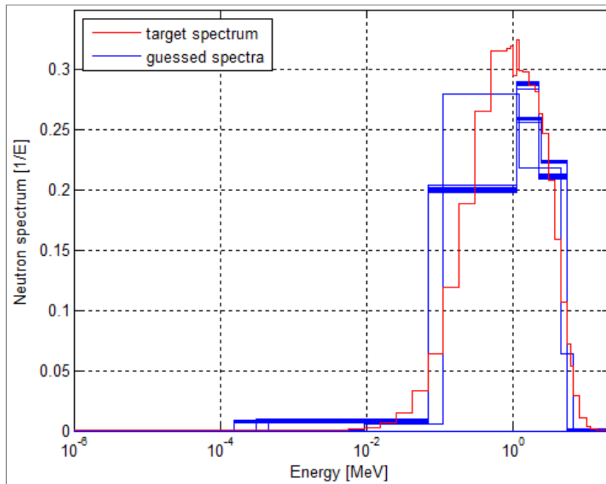
Figura 20 - Risultati dell'algorithm di unfolding realizzato in Matlab, a partire dalle correnti misurate dai 7 SPND in Tabella 18.
