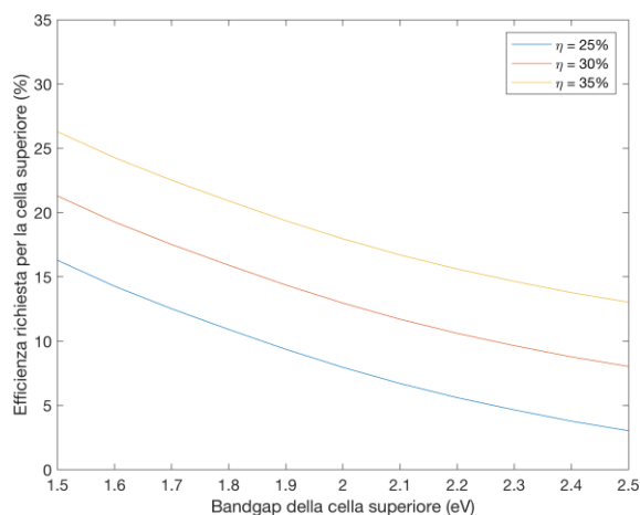
Figura 5: Efficienza richiesta per la cella frontale in funzione del bandgap della cella frontale per tre valori fissati di efficienza totale: η = 25% (curva blu), η = 30% (curva rossa) e η = 35% (curva gialla).
