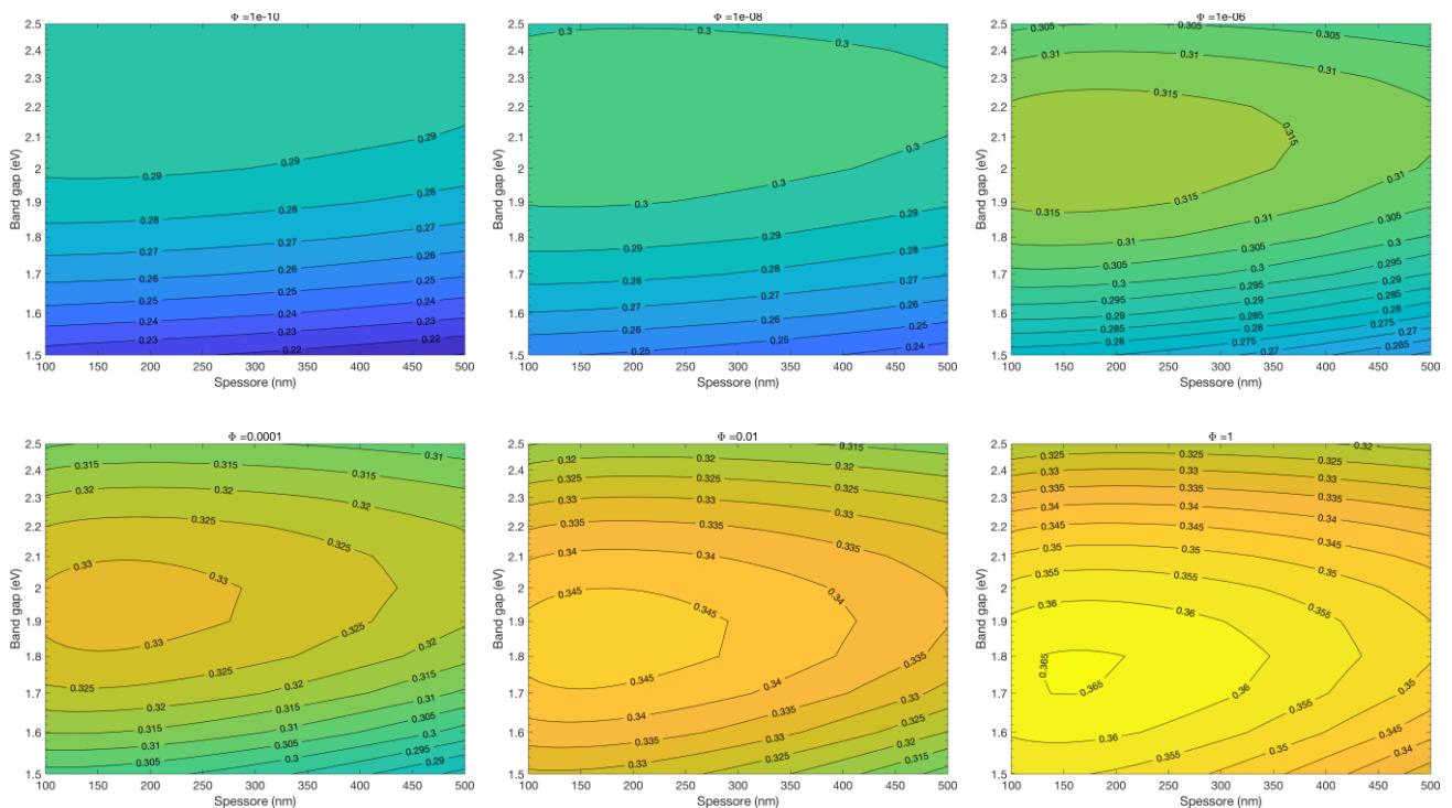
Figura 7: Spessore della cella frontale ottimo in caso di light trapping
