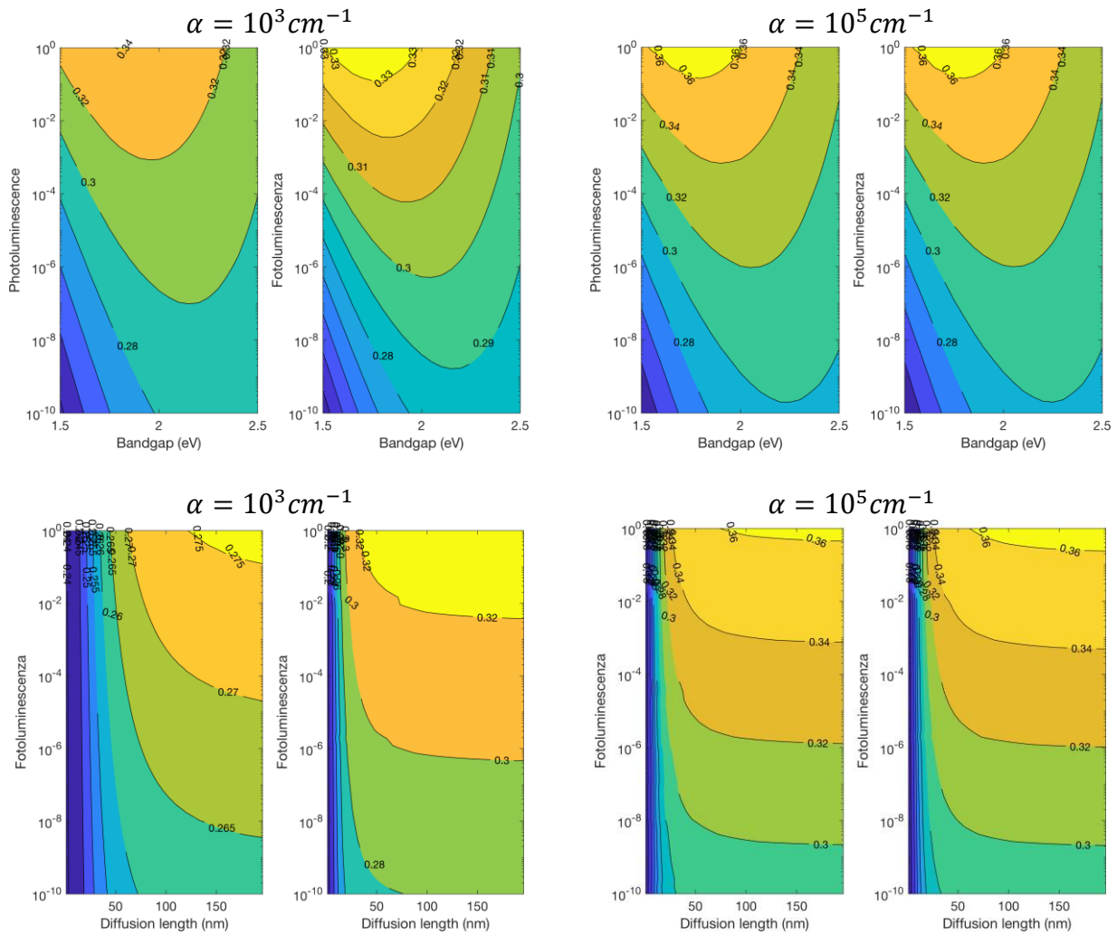
Figura 11: Efficienza totale al variare della fotoluminescenza e del bandgap (prima riga) e della lunghezza di diffusione (seconda riga) per valori di \alpha_0 = 10^3 \text{ cm}^{-1} (prima colonna) e \alpha_0 = 10^5 \text{ cm}^{-1} (seconda colonna)
