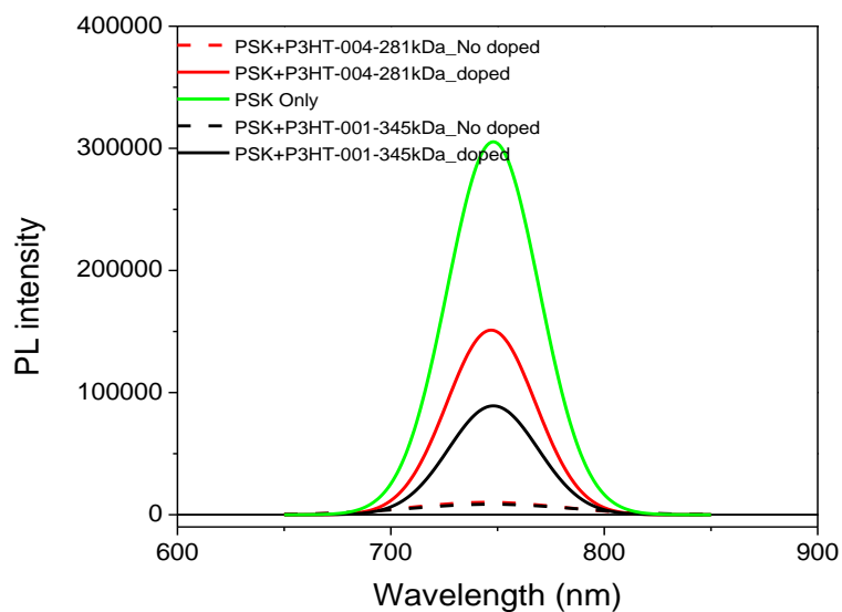
Figura 2.1.2.7: fotoluminescenza di HTM+PSK su mp-TiO 2 con strati di P3HT004-281 kDa e P3HT001-345 kDa e della sola perovskite
