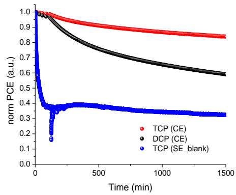
Figura 2.2.8: a) Stabilità in condizioni di light soaking di celle TCP, DCP e TCP 1step di riferimento; b) stabilità in condizioni di shelf life di celle di larga area TCP e DCP.
