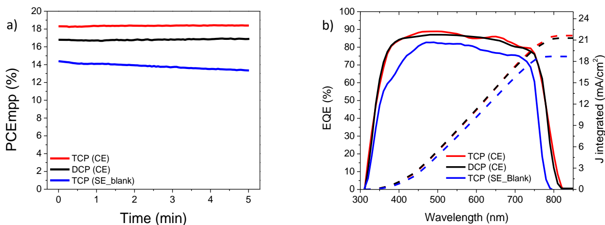
Figura 2.2.6: a) Efficienza di fotocorrente dei dispositivi al MPP sotto illuminazione AM1.5G. b) Curve EQE dei dispositivi realizzati.
