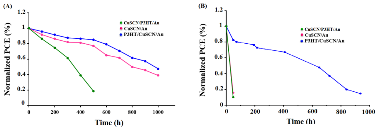
Figura 2.1.2.13: Misure di stabilità di dispositivi non incapsulati basati sulla struttura SnO 2 /perovskite/HTM/Au, con CuSCN, P3HT/CuSCN, CuSCN/P3HT come HTL. (A) condizioni ambientali ( shelf life ); (B) stress termico a 85 °C.
