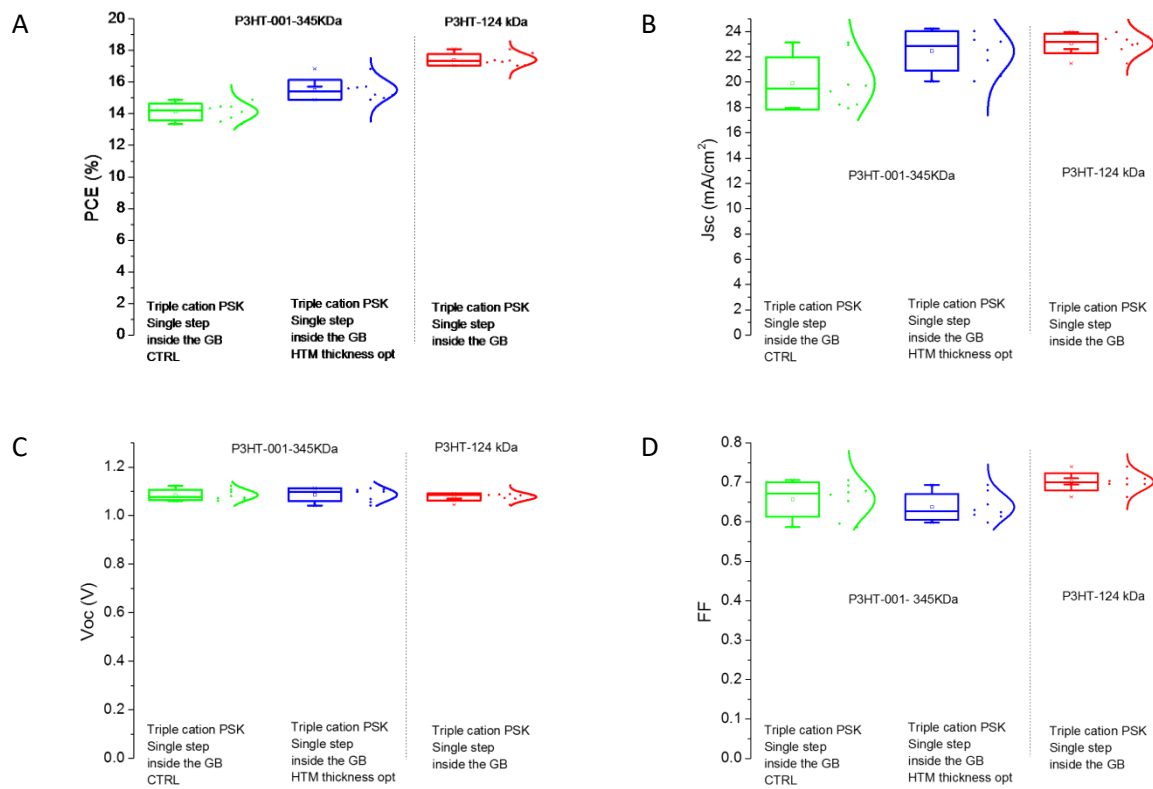
Figura 2.1.2.5: Prestazioni fotovoltaiche statistiche delle PSC fabbricate con perovskite a triplo catione utilizzando diversi P3HT come strato HTM: P3HT001-345 kDa (drogato) e con ottimizzazione dello spessore e P3HT-124 kDa (drogato).
