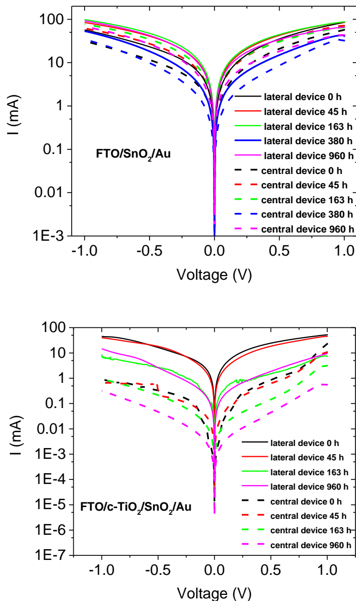
Figura 2.1.1.6: Caratteristiche a diodo per monitorare l'aumento della resistività del materiale ETL. Le diverse colorazioni indicano le curve registrate in funzione del tempo ad 85°C e 30% di RH.
