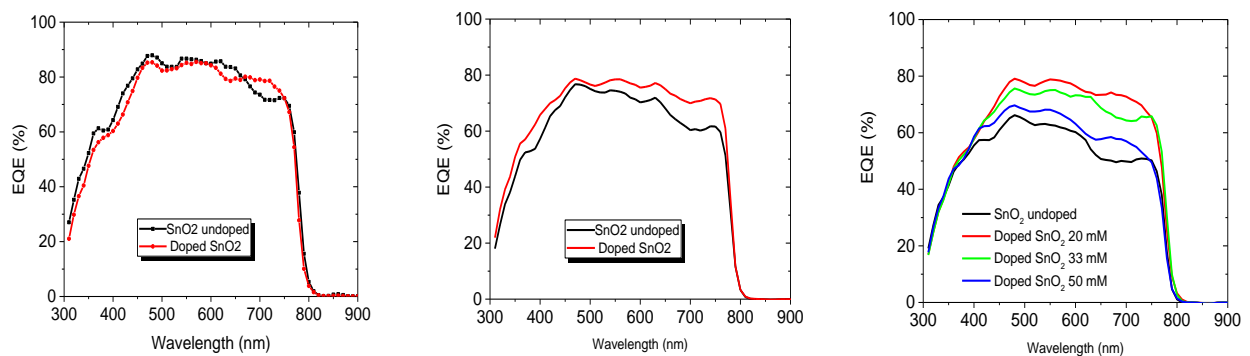
Figura 2.1.1.10: EQE della cella di riferimento (in nero) e della cella drogata con Cesio (rosso) presi appena depositate (sinistra), dopo 1600 ore (centro) e dopo 2800 ore (destra)
