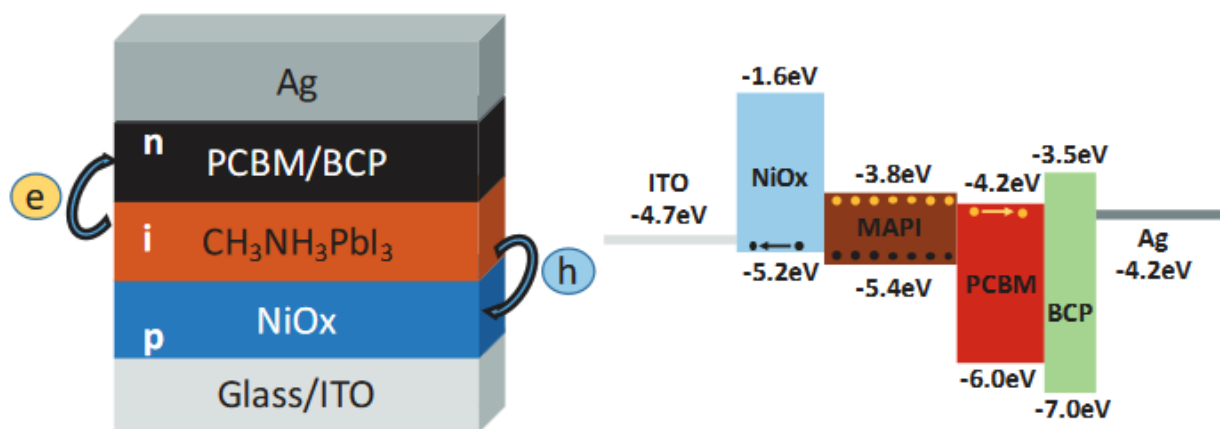
Figura 2.1.2.14: Struttura del dispositivo a perovskite con architettura invertita e schema energetico riportante i livelli energetici dei materiali costituenti il dispositivo.
