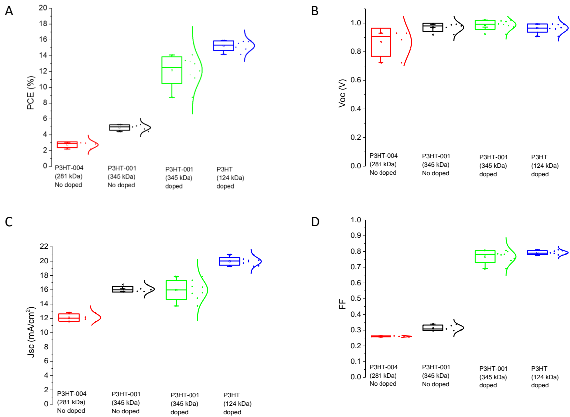
Figura 2.1.2.4: Prestazioni fotovoltaiche statistiche delle PSC fabbricate con perovskite a triplo catione utilizzando diversi P3HT come strato HTM: P3HT004-281 kDa (non drogato), P3HT001-345 kDa (drogato e non drogato) e P3HT-124 kDa (drogato).
