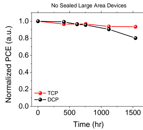
Figura 2.2.8: a) Stabilità in condizioni di light soaking di celle TCP, DCP e TCP 1step di riferimento; b) stabilità in condizioni di shelf life di celle di larga area TCP e DCP.
