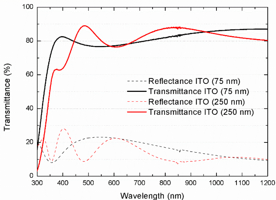
Figura 2.2.4: Trasmittanza (curve solide) e riflettanza (curve tratteggiate) di strati di ITO spessi 75 nm (linee nere) e 250 nm (linee rosse).
