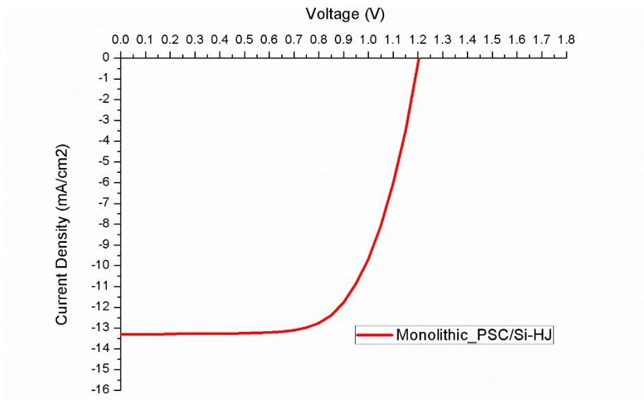
Figura 2.3.3: Curva J-V del dispositivo tandem silicio/perovskite monolitico.
