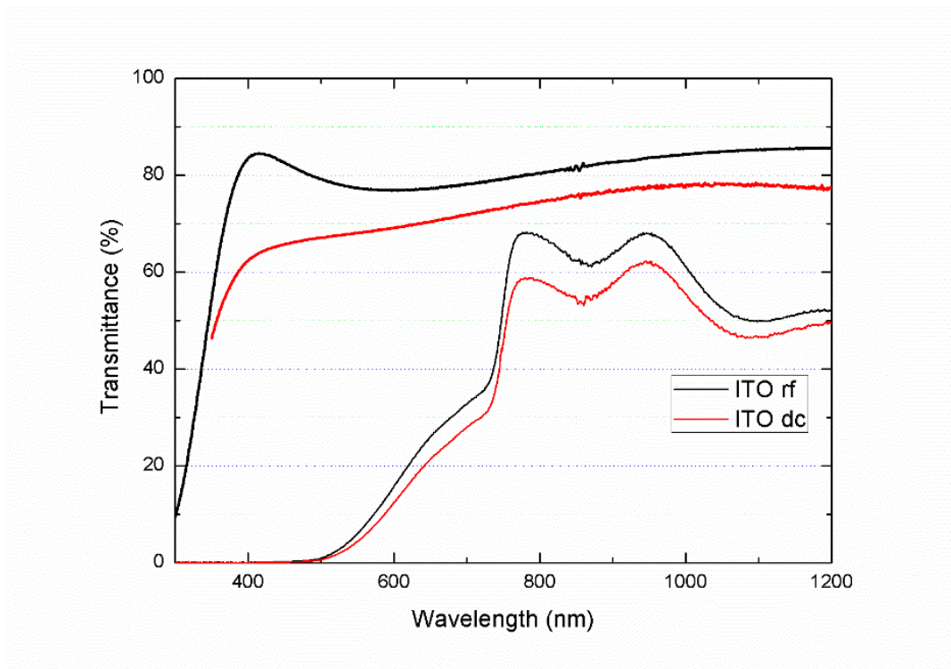
Figura 2.2.2: Trasmittanza da 300 nm a 1200 nm degli strati di ITO depositati mediante sputtering con sorgente DC (curva rossa) e RF (curva nera). Sono presenti anche le curve corrispondenti alla trasmittanza di due PSC semitrasparenti con contatto posteriore di ITO depositato per sputtering DC (curva rossa) e RF (curva nera).
