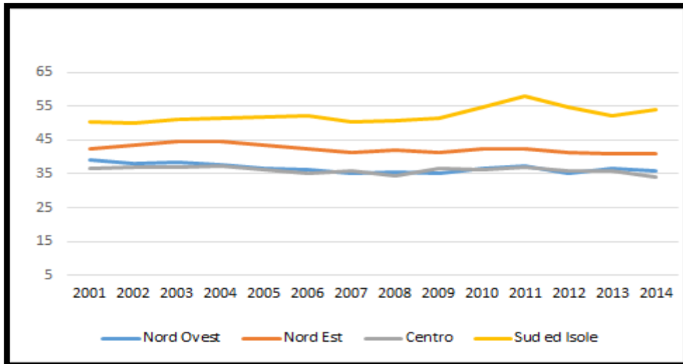
Figura 3. Dinamica dell'intensità energetica nel comparto industria in senso stretto e costruzioni (elaborazioni su dati ISTAT)
