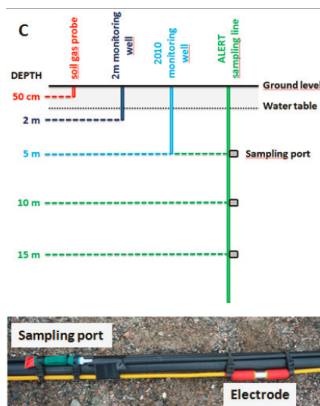
Figura 14. Sito CO2FieldLab: (a) le operazioni di perforazione; (B) vista del sito, mostrando serbatoio CO2 a destra, la testa di pozzo a fianco del serbatoio all'interno del recinto, e una varietà di edifici di controllo / operazioni - notare che il foro immerge 45° e inietta alla profondità di 20 m a metà strada tra il serbatoio e la cabina portatile blu; (C) il layout di pozzi per tutta l'area (a sinistra) e il dettaglio della zona di iniezione (a destra); (D) distribuzione della profondità di diversi pozzi di campionamento delle acque sotterranee; (E) West Bay sistema a più livelli (Gal et al, 2013;.. Barrio et al, 2013; Jones et al 2014).
