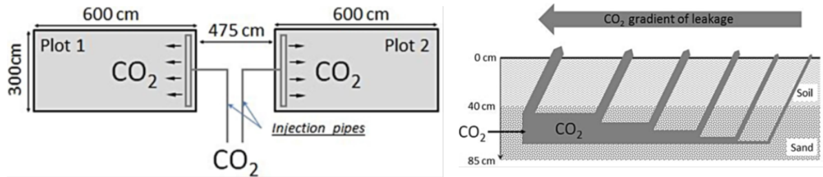
Figure 5. Schema del sito di iniezione di Grimsrud Farm (a) pianta; (b) profilo che mostra il gradiente di perdita creato (Moni and Rasse, 2014).
