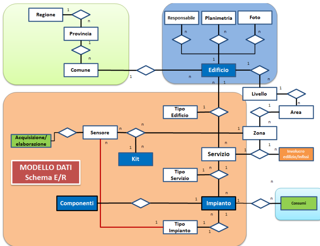
Figura 1: Schema concettuale E/R generale Sezione Edifici
