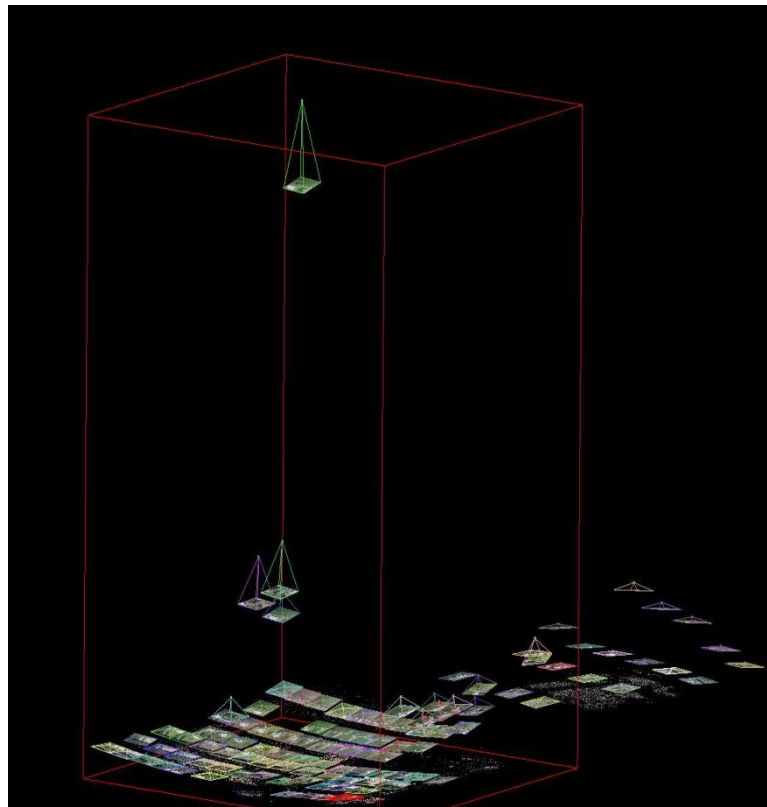
Figura 73: Triangolazione tramite VisualSFM
