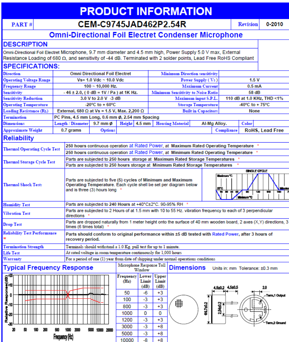
Figura 81: Datasheet microfono per modulo B13/A17
