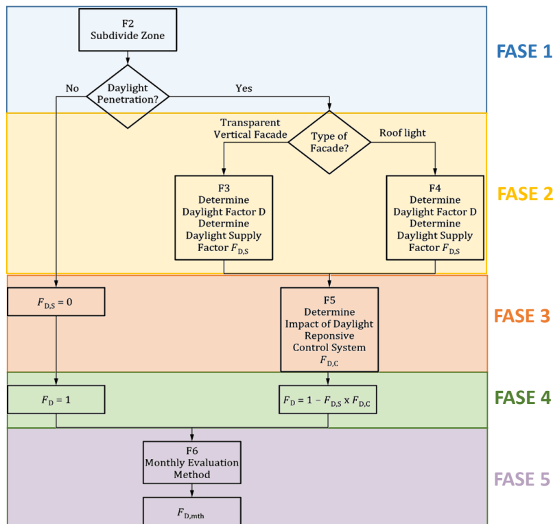
Figura 4. Flow-chart descrittivo della procedura di calcolo di F_D [2]
