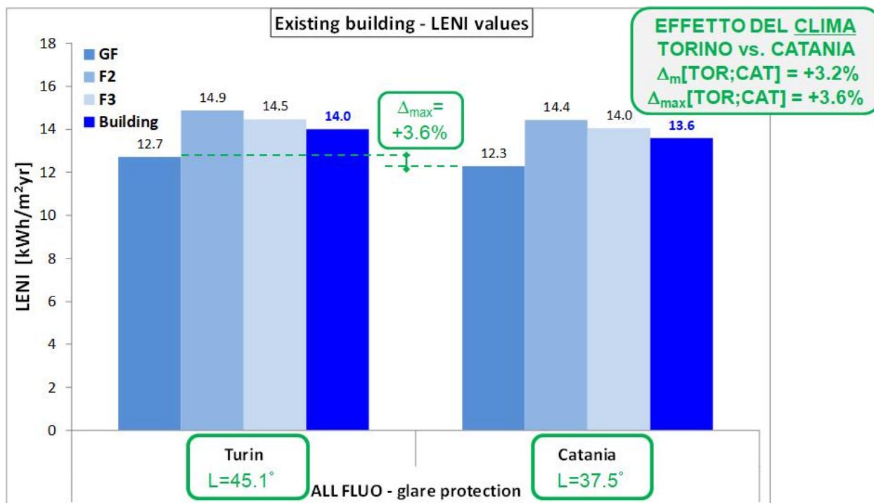
Figura 18 – Valori LENI ottenuti per gli edifici esistenti (scenario 1): influenza del clima.
