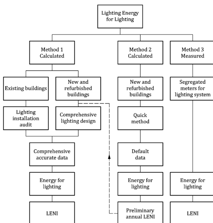
Figura 1. Flow-chart relativo alle possibili modalità di calcolo del LENI secondo la norma EN15193-1:2017 [2]
