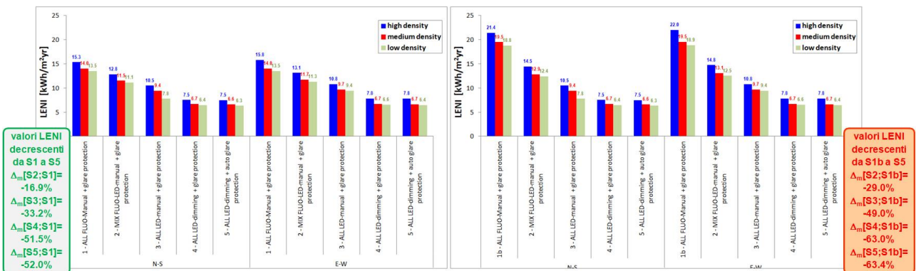
Figura 26 – Valori LENI ottenuti per i 4 interventi di retrofit, messi a confronto con lo scenario 1 o 1b.
