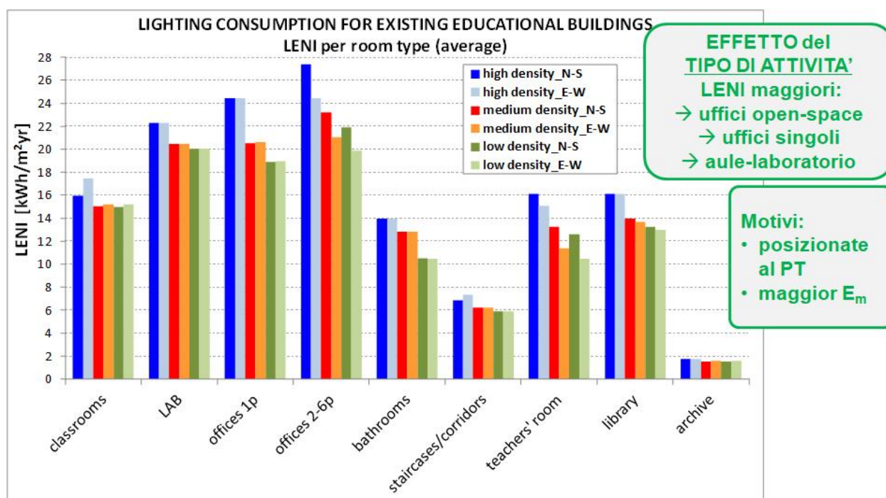
Figura 22 – Valori LENI ottenuti per gli edifici esistenti (scenario 1): influenza della destinazione d'uso prevista nei vari ambienti.
