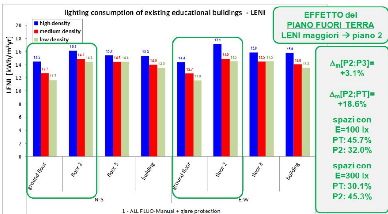
Figura 21 – Valori LENI ottenuti per gli edifici esistenti (scenario 1): influenza del piano fuori terra.
