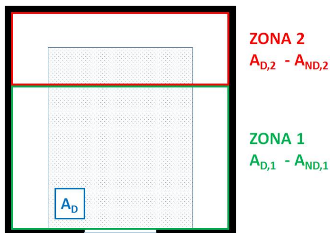
Figura 14: Ambiente suddiviso in 2 zone con diverse funzioni, e caratteristiche impiantistiche
