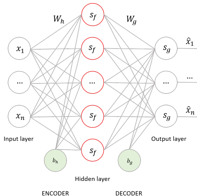
Figura 5: Architettura di un Auto-Encoder
