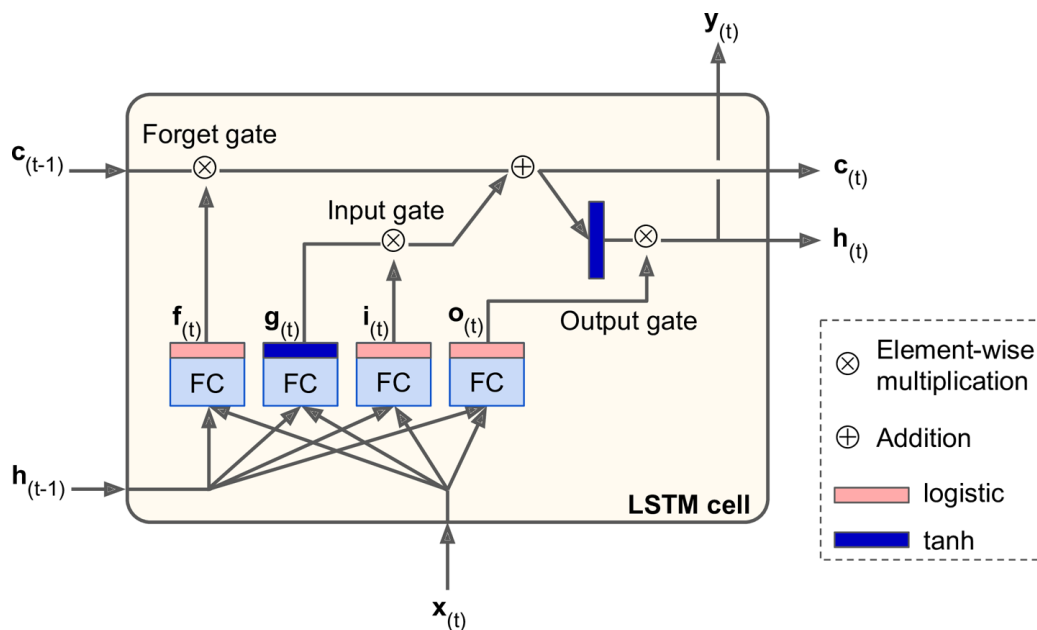
Figura 4: struttura della cella LSTM
