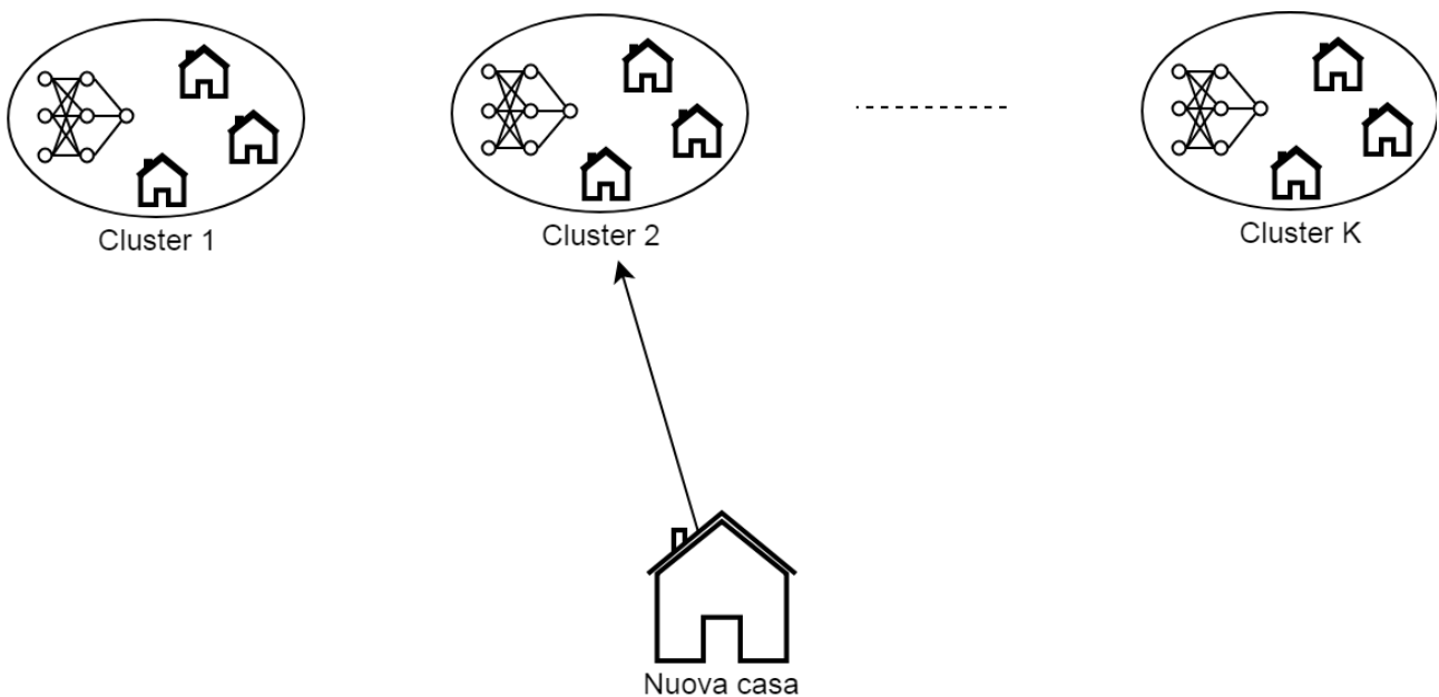
Figura 31: strategia di clustering per la disaggregazione del consumo elettrico
