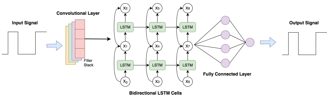
Figura 14: Rete realizzata con celle LSTM bidirezionali
