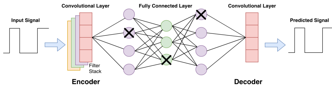
Figura 17: Rete realizzata con auto encoder
