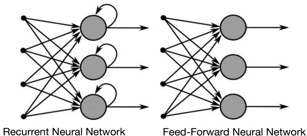
Figura 3: esempi di reti neurali ricorrenti e feed forward
