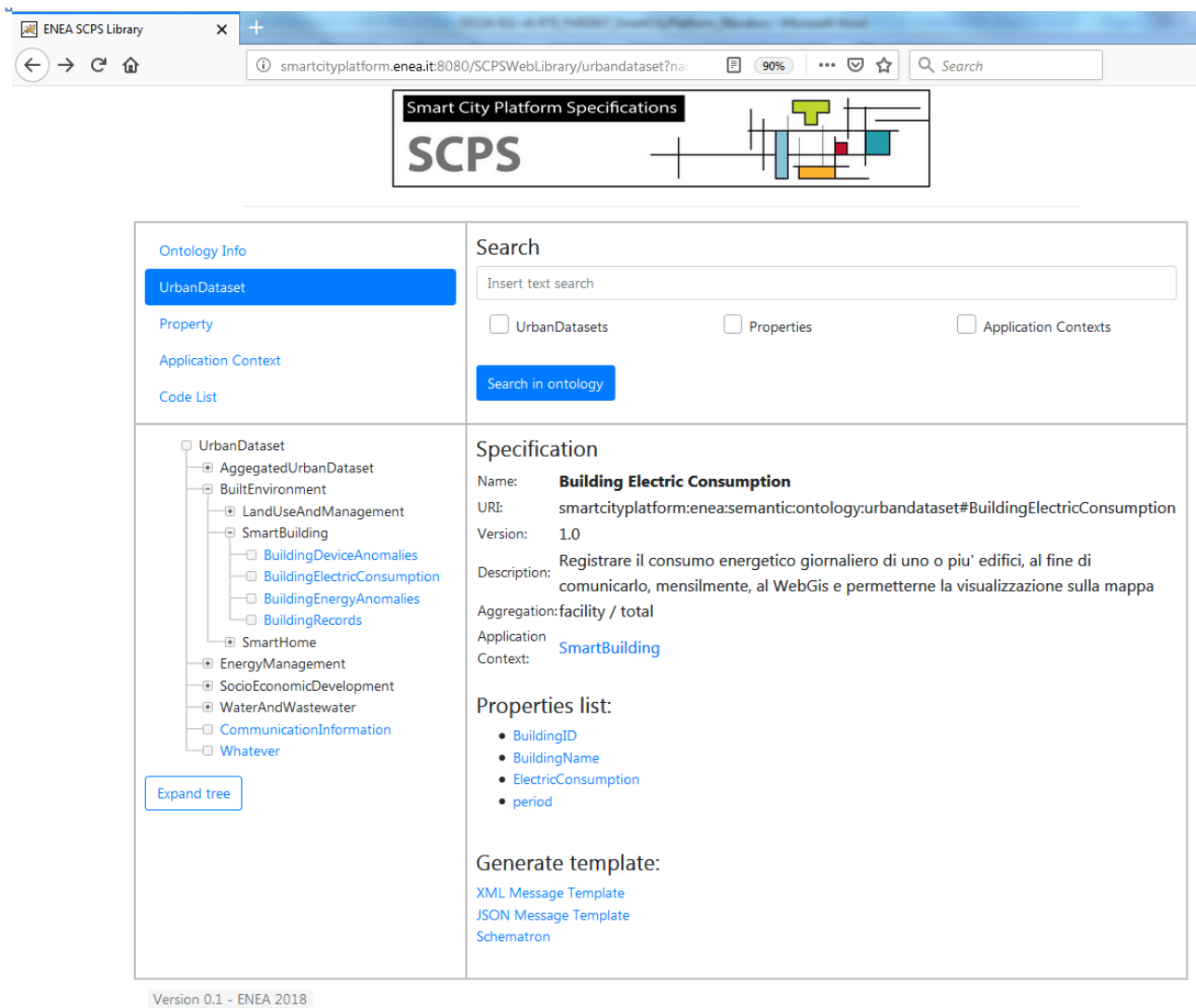
Figura 17 – Interfaccia di navigazione Ontologia
