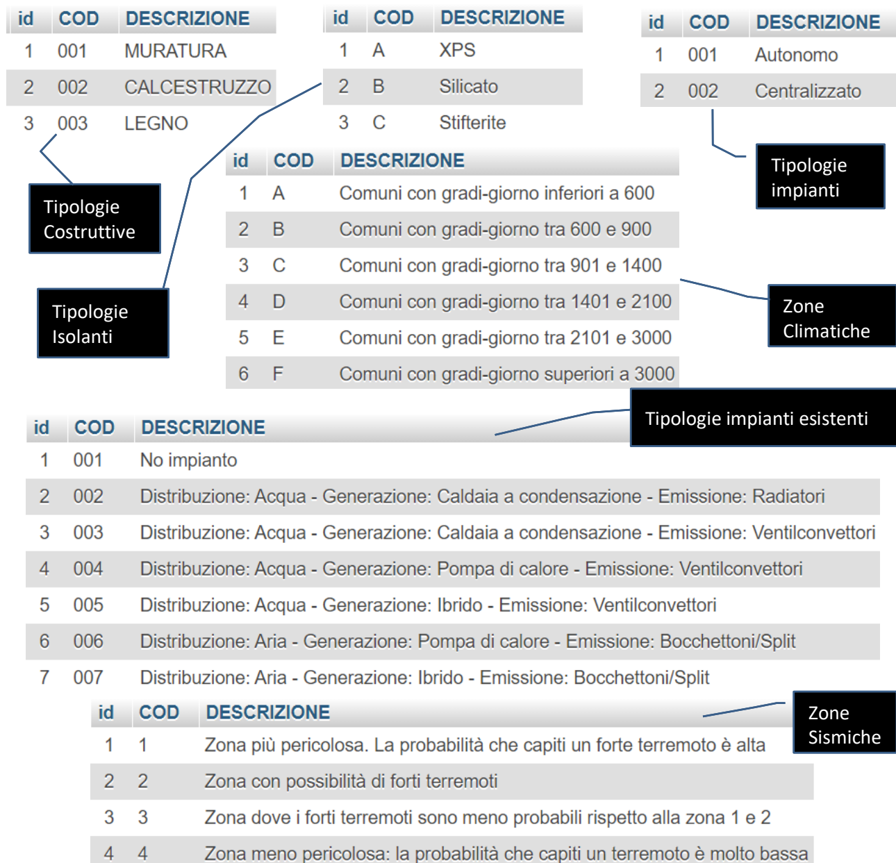
Figura 19: Contenuto delle tabelle tipologie costruttive, impianti, impianti esistenti, isolanti, zone sismiche e climatiche all'atto di rilascio del portale
