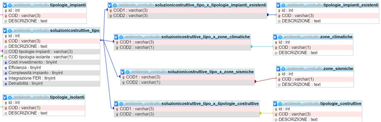
Figura 20: tabella soluzionicostruttive_tipo e relative tabelle per implementare la matrice dinamica delle scelte
