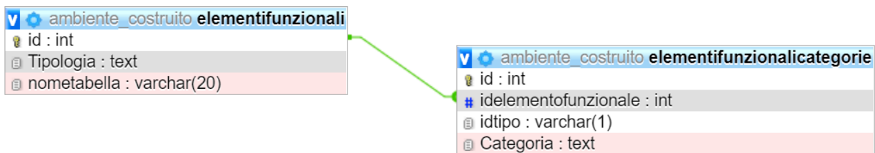
Figura 11: tabella elementifunzionali e sua relazione con la tabella elementifunzionali
