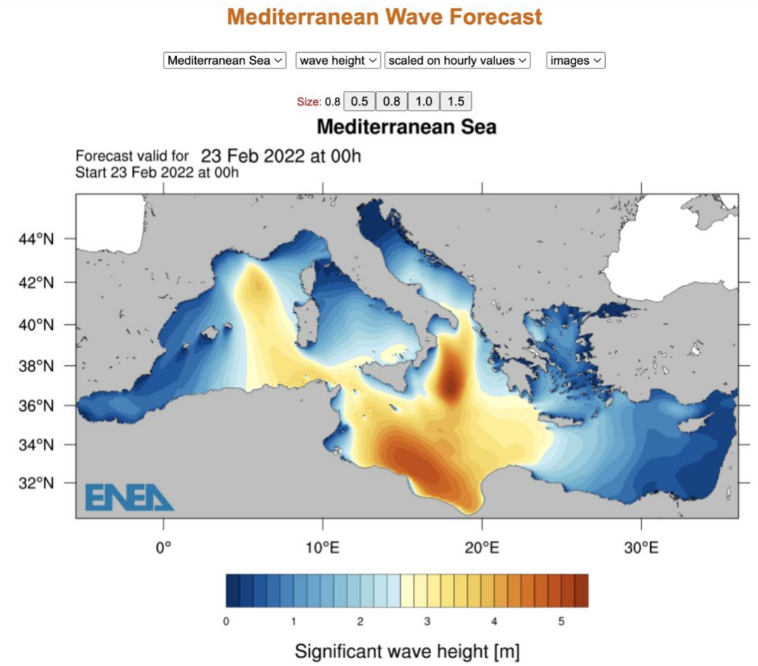
Figura 3A: immagine da https://climaweb.casaccia.enea.it/en/WW3MED/ relativa alla previsione dell'ampiezza significativa delle onde sull'intero bacino mediterraneo.
