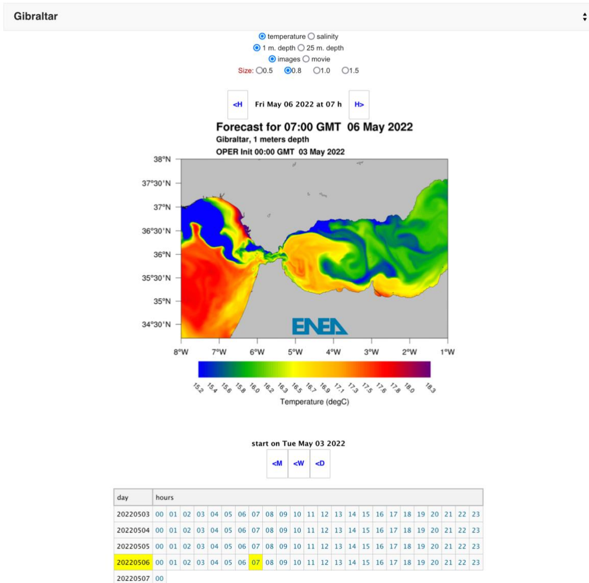
Figura 2: Immagine da http://climaweb.casaccia.enea.it/en/MITO relativa alla previsione della temperatura per l'area dello stretto di Gibilterra.
