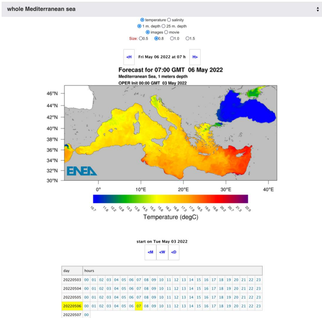
Figura 1: Immagine da http://climaweb.casaccia.enea.it/en/MITO relativa alla previsione della temperatura sull'intero dominio di calcolo
