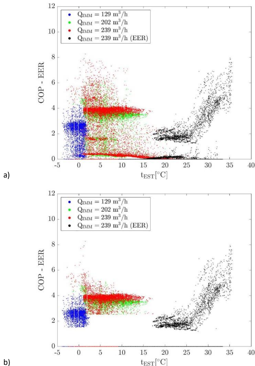
Figura 2-16 Andamenti del COP e dell'EER (valori con risoluzione 5 minuti) al variare della temperatura esterna: per tutti i punti operativi campionati (a) e senza i punti operativi di produzione di ACS filtrati secondo il criterio di soglia proposto (b)
