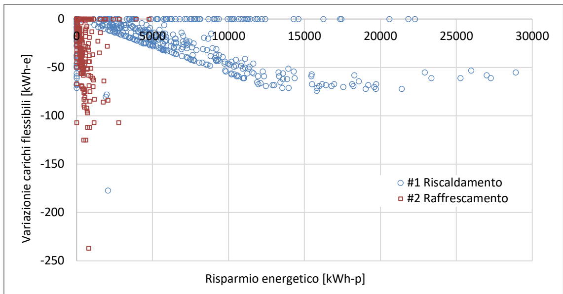
Figura 3.1 – Riscaldamento e raffrescamento.
