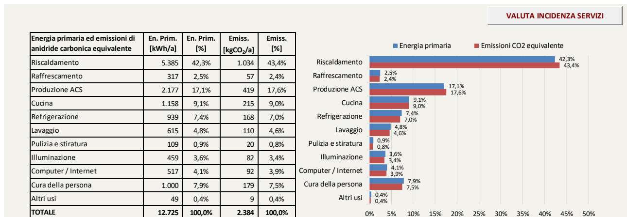
Figura 4.2 – Ripartizione consumi energia primaria ed emissioni. Nuova versione.
