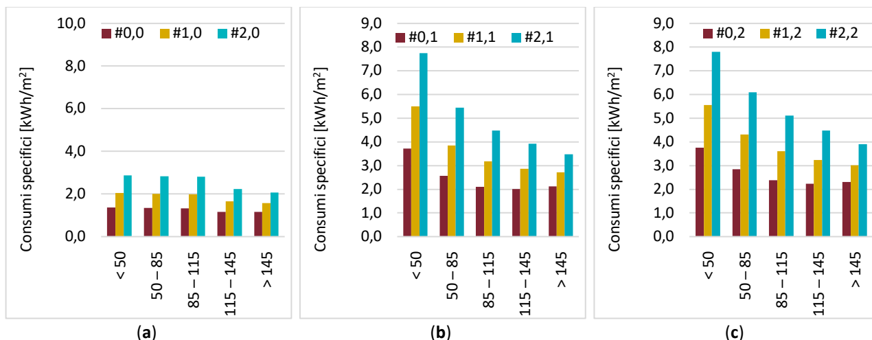
Figura 3.22 – Napoli: consumi specifici di energia primaria per raffrescamento (a) Dotazione esistente; (b) Dotazione esistente + 1 climatizzatore; (c) Dotazione esistente + 2 climatizzatori.
