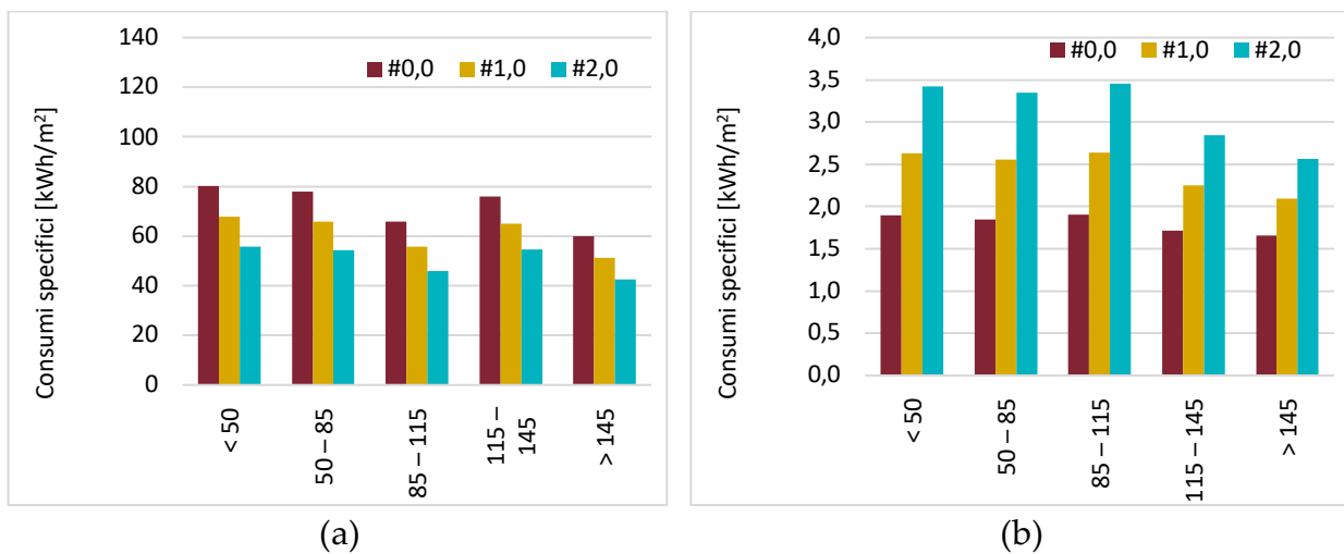
Figura 3.16 – Firenze: consumi specifici di energia primaria (a) Riscaldamento; (b) Raffrescamento.
