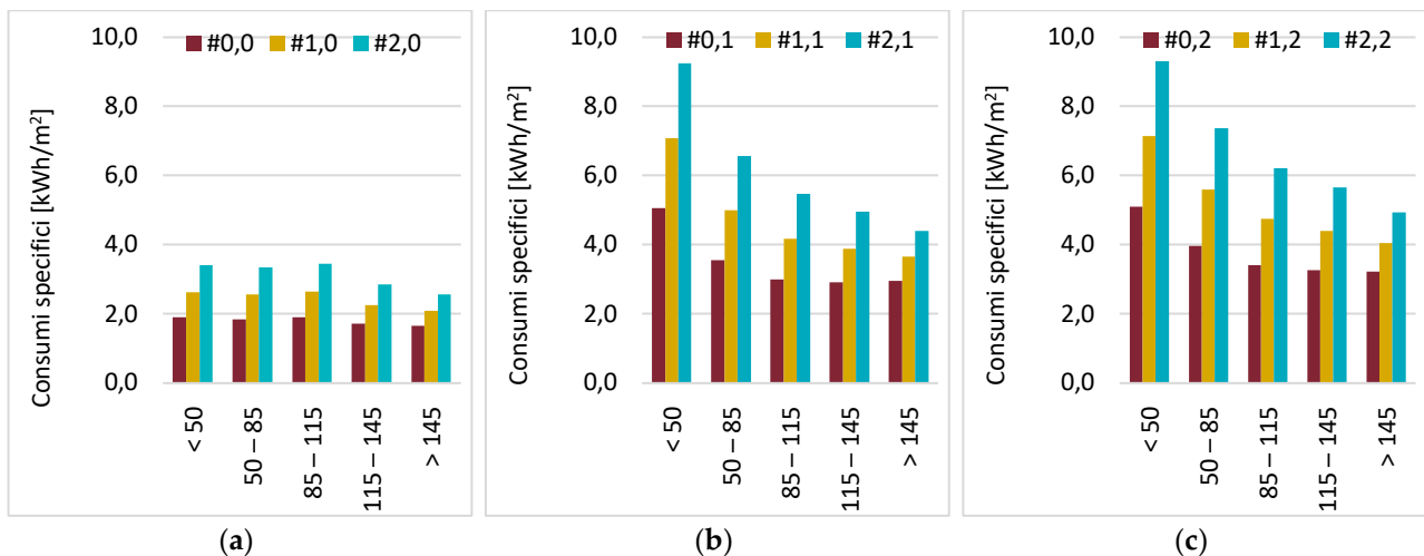
Figura 3.20 – Firenze: consumi specifici di energia primaria per raffrescamento (a) Dotazione esistente; (b) Dotazione esistente + 1 climatizzatore; (c) Dotazione esistente + 2 climatizzatori.
