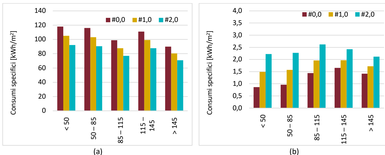
Figura 3.15 – Milano: consumi specifici di energia primaria (a) Riscaldamento; (b) Raffrescamento.
