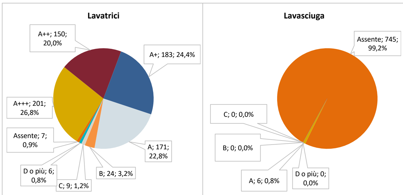
Figura 2.18 – Presenza e classe energetica di lavatrici e lavasciuga.
