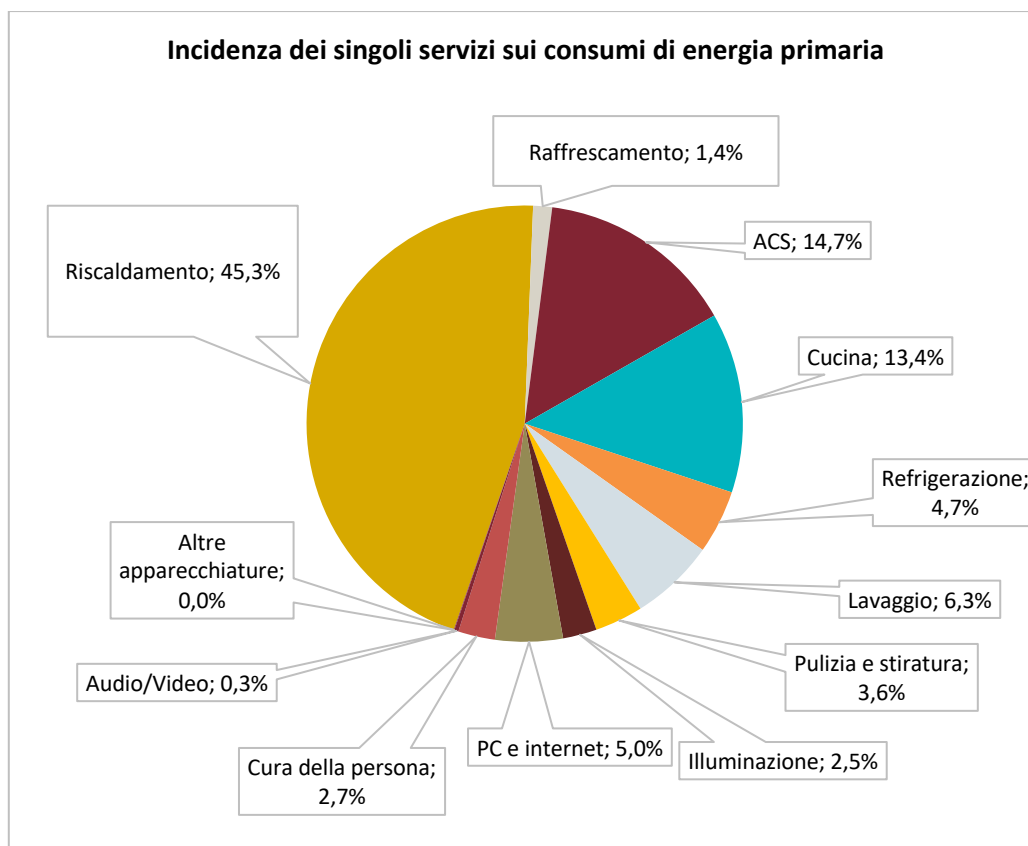
Figura 2.28 – Incidenza dei singoli servizi sui consumi di energia primaria.
