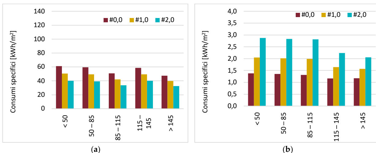
Figura 3.18 – Napoli: consumi specifici di energia primaria (a) Riscaldamento; (b) Raffrescamento.
