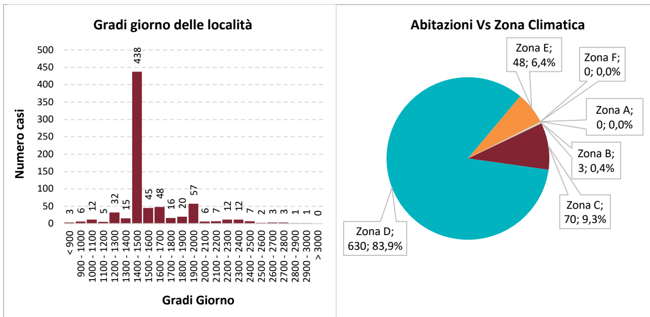
Figura 2.3 – Gradi giorno delle località e zona climatica per le abitazioni considerate.
