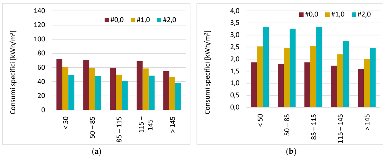
Figura 3.17 – Roma: consumi specifici di energia primaria (a) Riscaldamento; (b) Raffrescamento.
