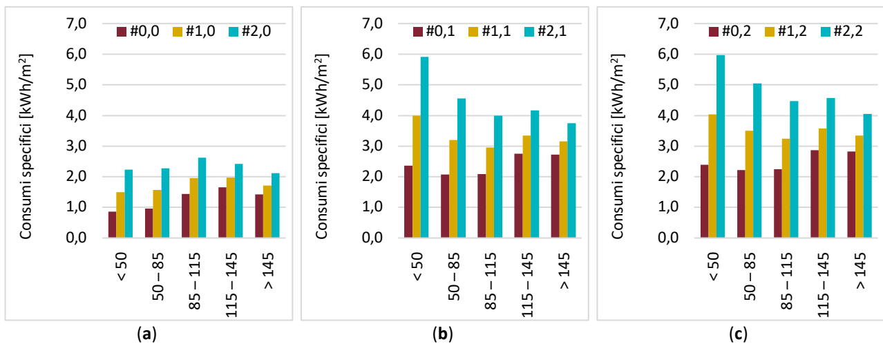
Figura 3.19 – Milano: consumi specifici di energia primaria per raffrescamento (a) Dotazione esistente; (b) Dotazione esistente + 1 climatizzatore; (c) Dotazione esistente + 2 climatizzatori.
