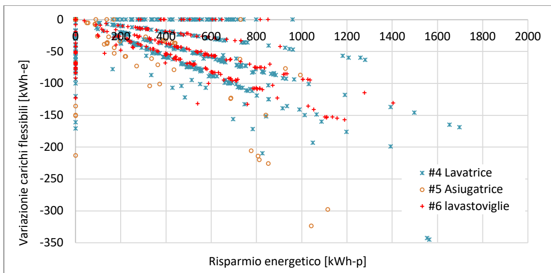
Figura 3.4 – Lavaggio (lavatrici, asciugatrici, lavastoviglie).
