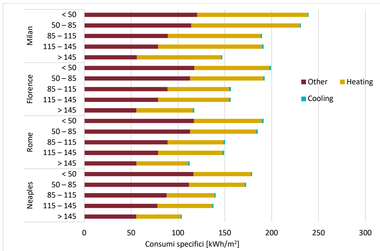
Figura 3.14 – Consumi specifici di energia primaria per riscaldamento, raffrescamento, altri usi.
