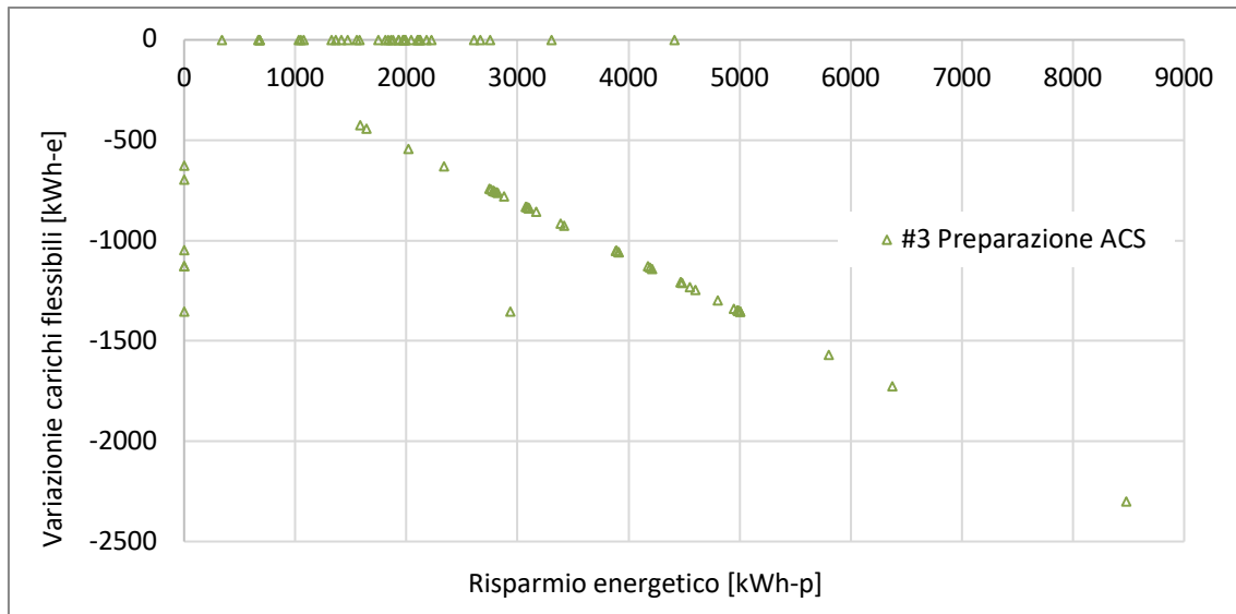
Figura 3.2 – Preparazione acqua calda sanitaria.
