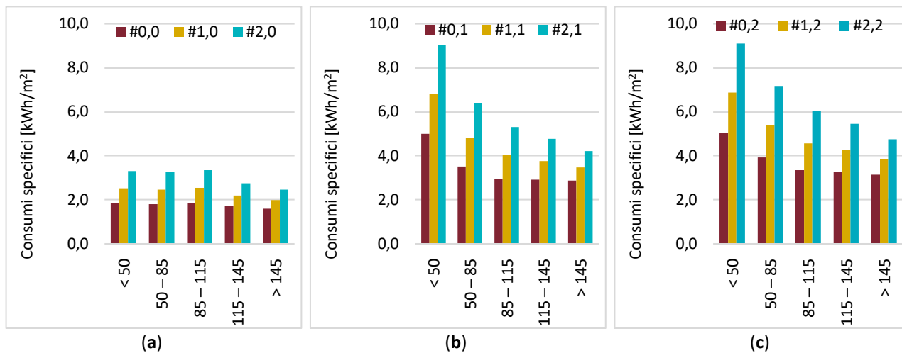
Figura 3.21 – Roma: consumi specifici di energia primaria per raffrescamento (a) Dotazione esistente; (b) Dotazione esistente + 1 climatizzatore; (c) Dotazione esistente + 2 climatizzatori.
