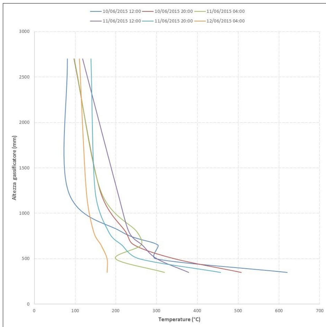
Figura 5.8. Profilo di temperatura all'interno del gassificatore durante le prove di gassificazione del 10-12/06/2015
