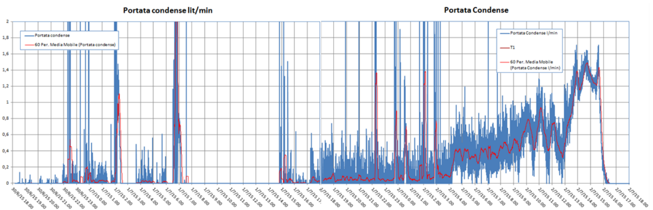
Figura 5.3. Esempio della misura della portata delle condense di ritorno al waterjacket a valle dell'aeroterme
