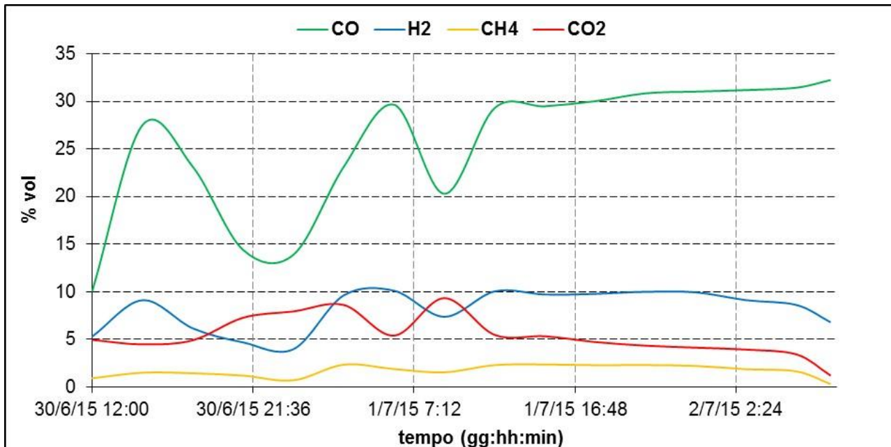
Figura 5.13. Andamento nel tempo della composizione del syngas grezzo DJ002P del 30/06 – 02/07/2015
