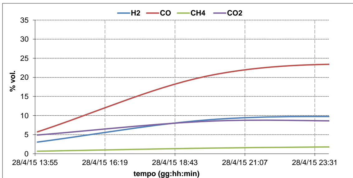
Figura 5.7. Andamento nel tempo della composizione del syngas grezzo DJ002P del 28-30/04/2015
