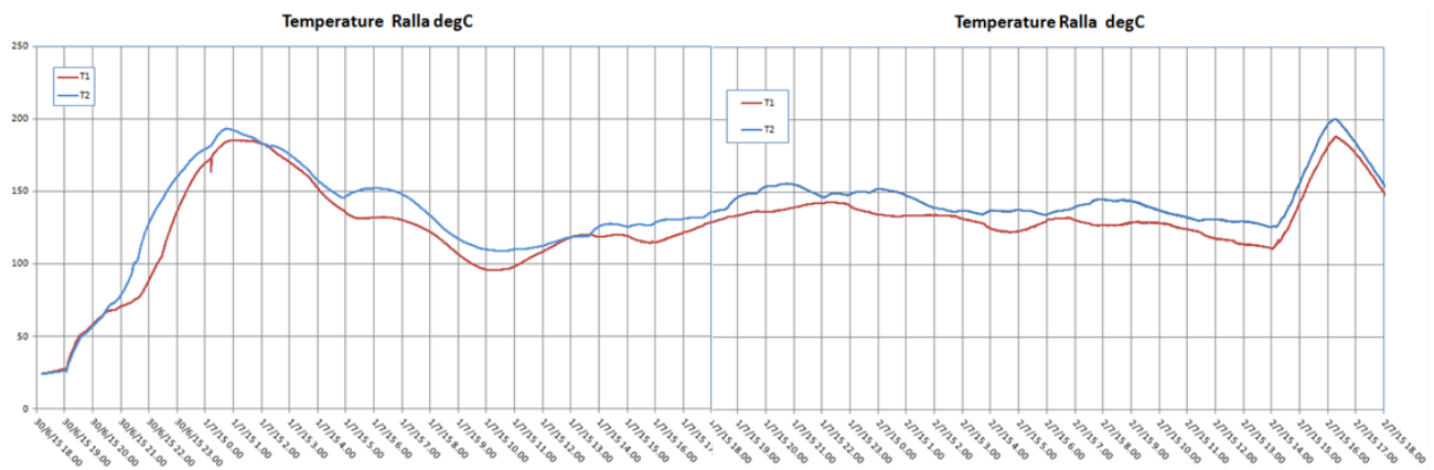
Figura 5.4. Esempio della misura della temperatura in prossimità della ralla di sostegno della griglia rotante
