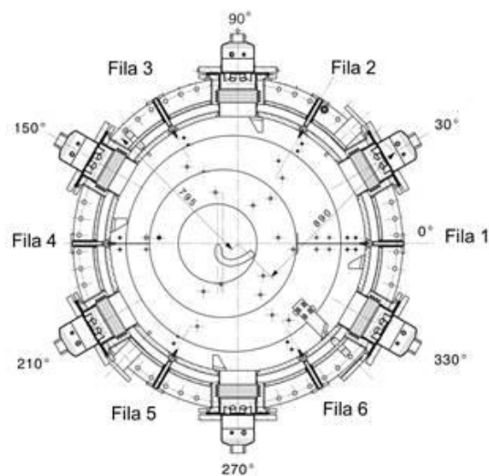
Figura 2.3. Sezione del gassificatore: posizione degli irradiator di accensione
