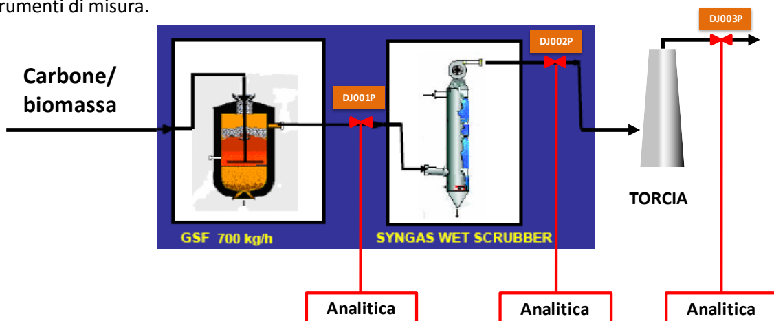
Figura 2.8. Campionamento del syngas: punti DJ001 (gassificatore), DJ002 (scrubber) e DJ003 (torcia)
