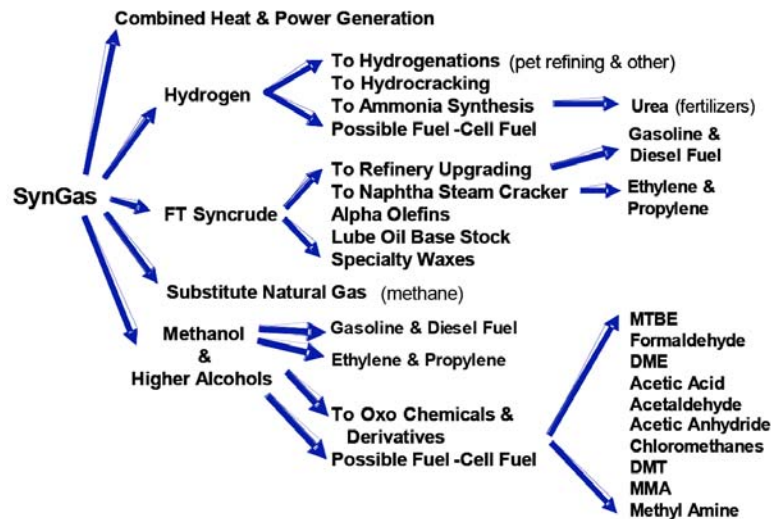
Figura 1: Principali prodotti ottenibili dal gas di sintesi
