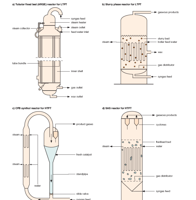
Fig. 6: principali tipologie di reattori FT usati dalla Sasol (da Collot, 2004)
