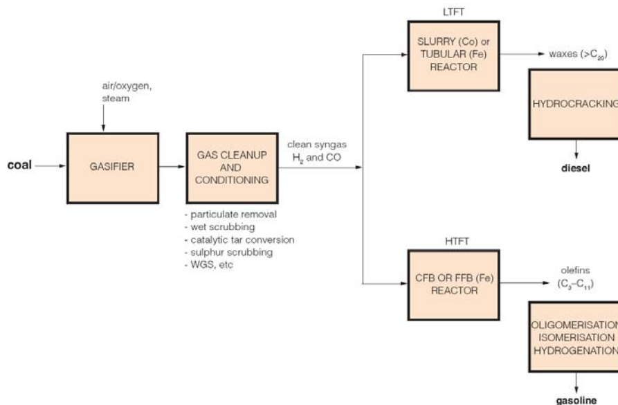
Figura 5 - Schema del processo FT
