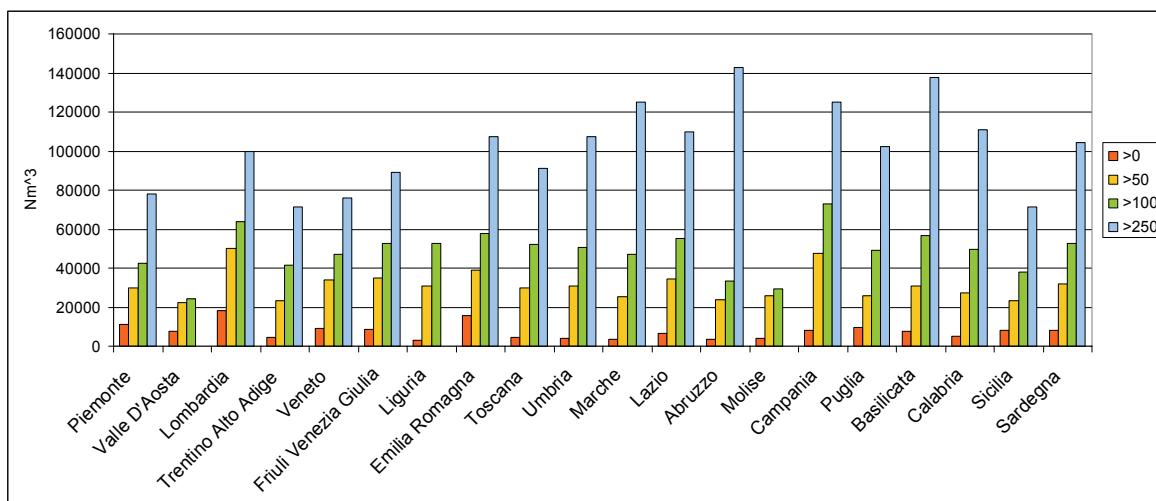
Figura 2.19– Potenziale lordo medio aziendale al variare della soglia aziendale
