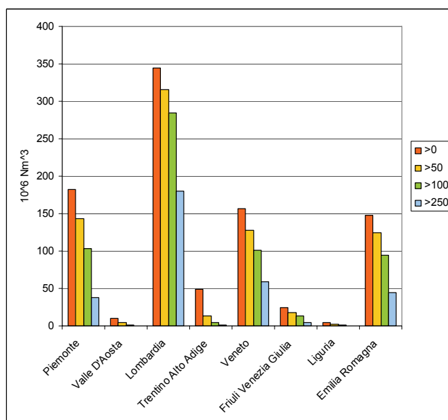
Figura 2.15 – Potenziale lordo per le Regioni del Nord al variare della soglia aziendale
