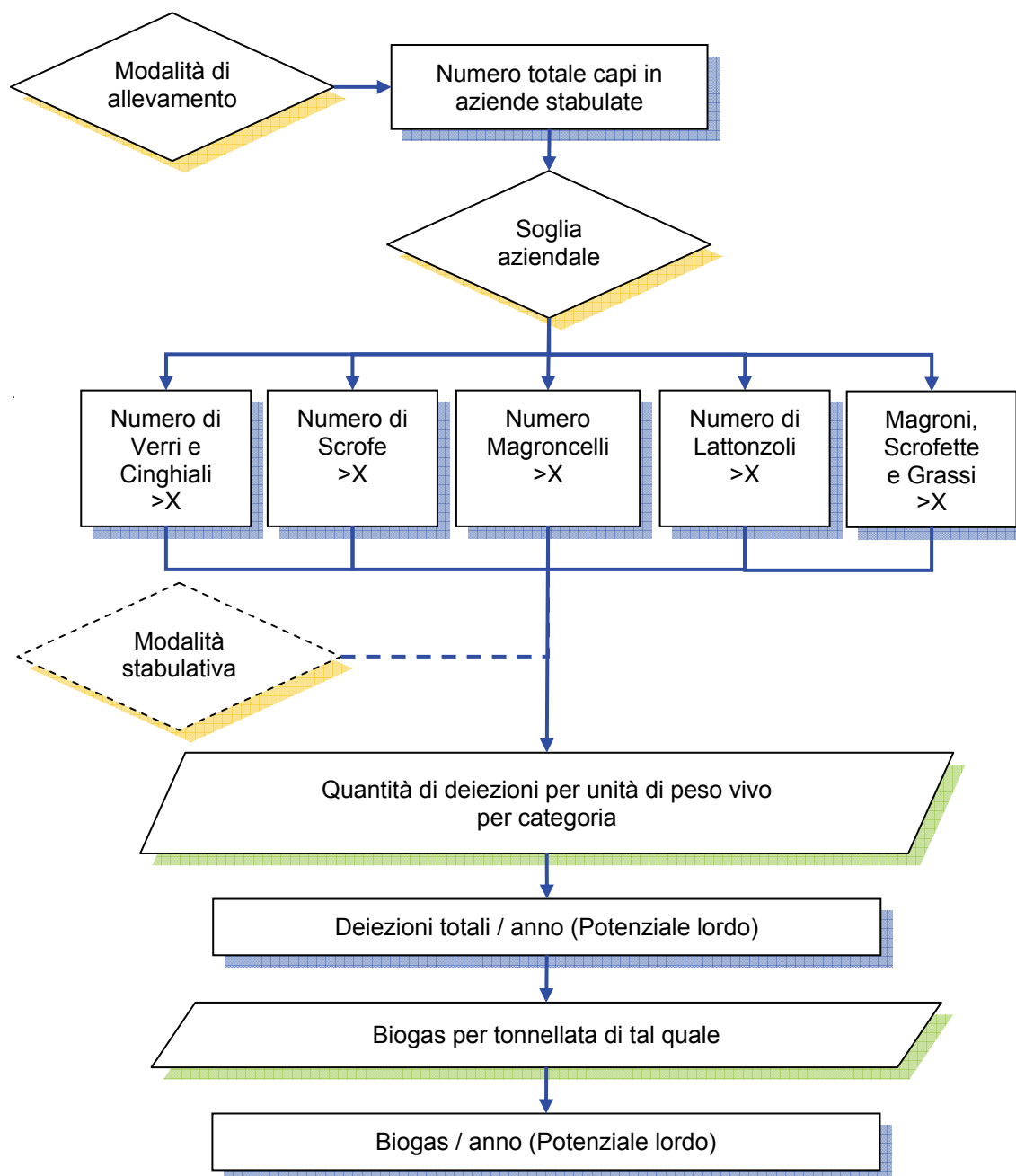
Figura 3.10 - Schema di flusso per la stima del potenziale (lordo) da reflui suini valorizzabile energeticamente
