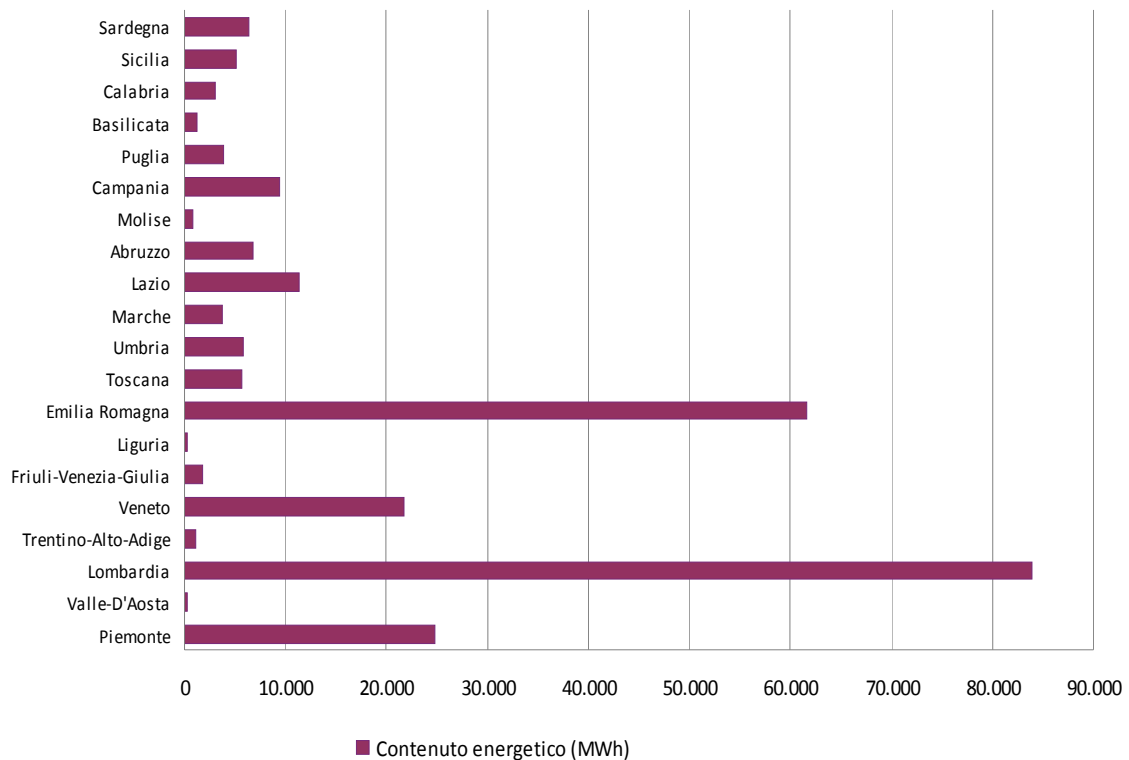
Figura 4.15 – Stima del contenuto energetico per regione del biogas producibile da scarti di macellazione
