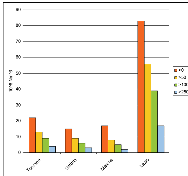
Figura 2.16 – Potenziale lordo per le Regioni del Centro al variare della soglia aziendale
