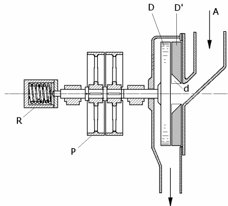
Figura 7. Macchine di macinazione per flessione/taglio: mulino a dischi
