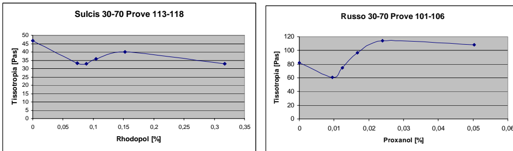
Figura 24. Tissotropia della miscela in funzione del dosaggio separato degli additivi
