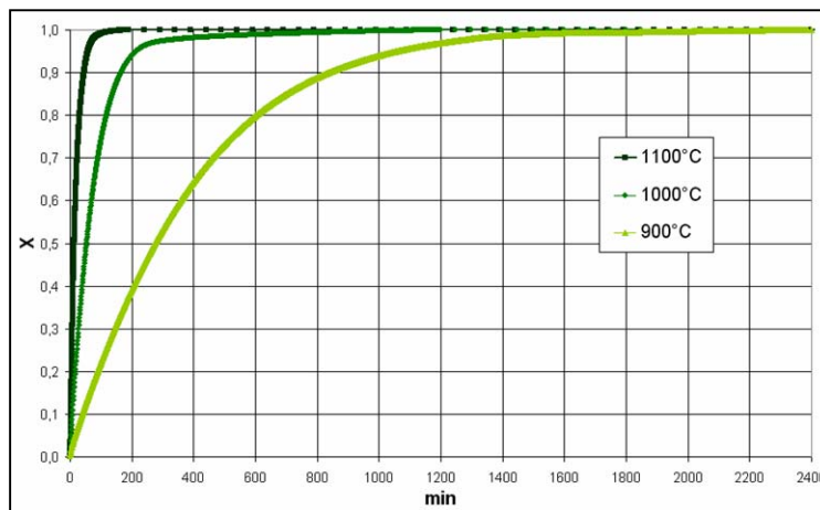
Figura 19: Andamento della conversione X nel tempo per campione di carbone Sulcis
