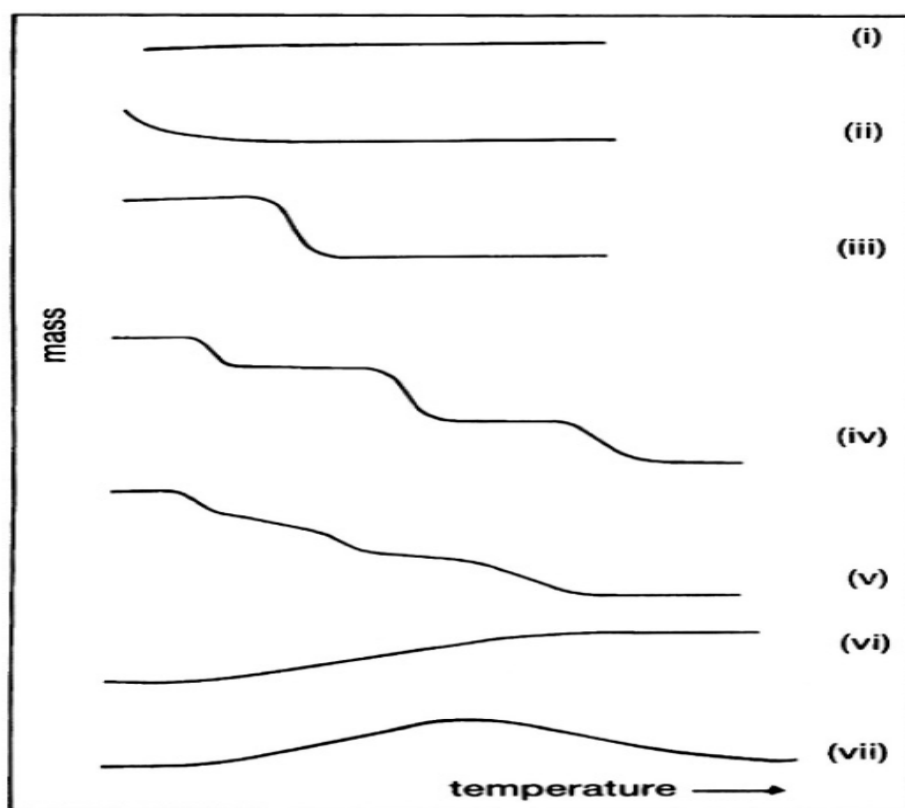
Figura 3: curve-massa temperatura
