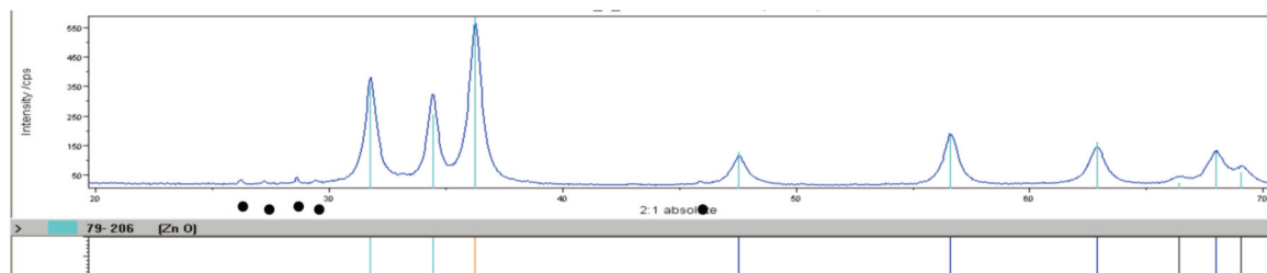
Diffratogramma di raggi X di un campione di sorbente utilizzato per la desolforazione
