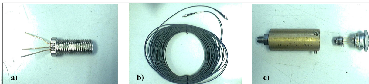
Figura 9 - a) trasmettitore per fibre ottiche HFBR-1204; b) fibra ottica HFBR-3000 con connettori SMA; c) accoppiatore e sensore ottico su connettore Lemo 2C;
