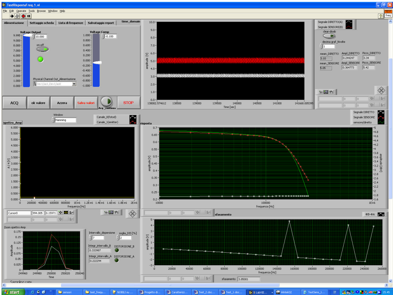
Figura 11 - Pannello frontale di "TestRispostaFreq.1" alla fine del test del sensore numero 1
