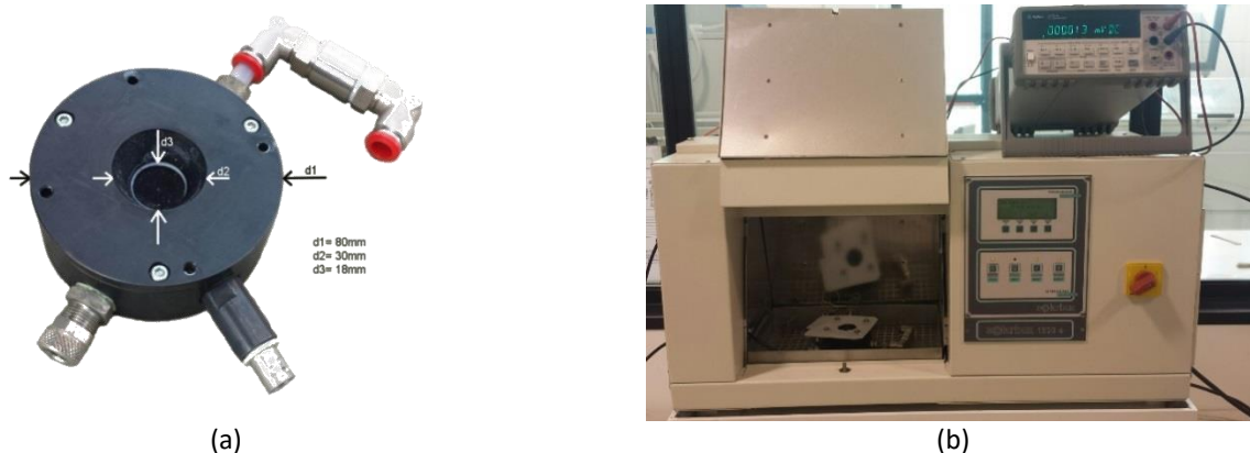
Figura 15: a) Sensore a termopila utilizzato nella fase preliminare di messa a punto della metodica di misura della radiazione concentrata; b) Caratterizzazione del sensore a termopila mediante misure di tensione effettuate in corrispondenza di flussi di radiazione crescenti e generati mediante una SolarBox.
