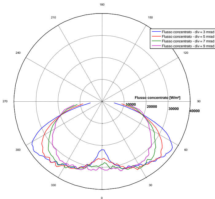
Figura 6. Diagramma polare delle distribuzioni del flusso solare concentrato sul tubo assorbitore, ottenute a diversi errori ottici
