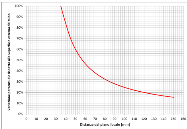
Figura 13: Variazione percentuale del flusso solare concentrato rispetto al valore misurato sulla superficie esterna del ricevitore.
