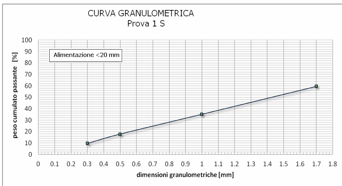
Figura 5.20. Distribuzione granulometrica del prodotto della prova 1S
