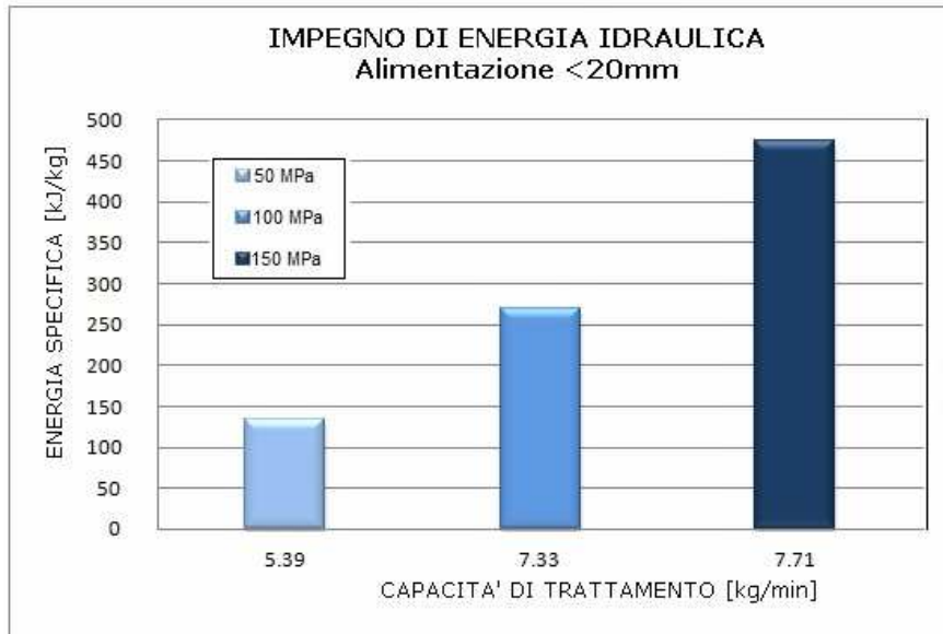
Figura 5.37. Confronto Energia specifica E_s in funzione della capacità di trattamento per diversi livelli di pressione. Diametro ugello: 0,8 mm
