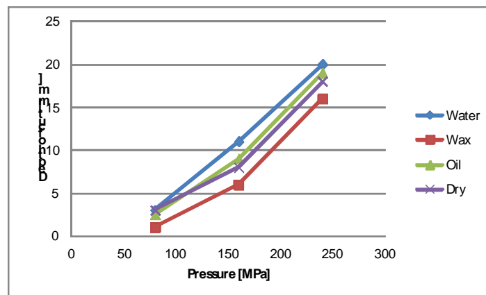
Figura 4.10. Profondità di taglio[mm] alle diverse condizioni sperimentali
