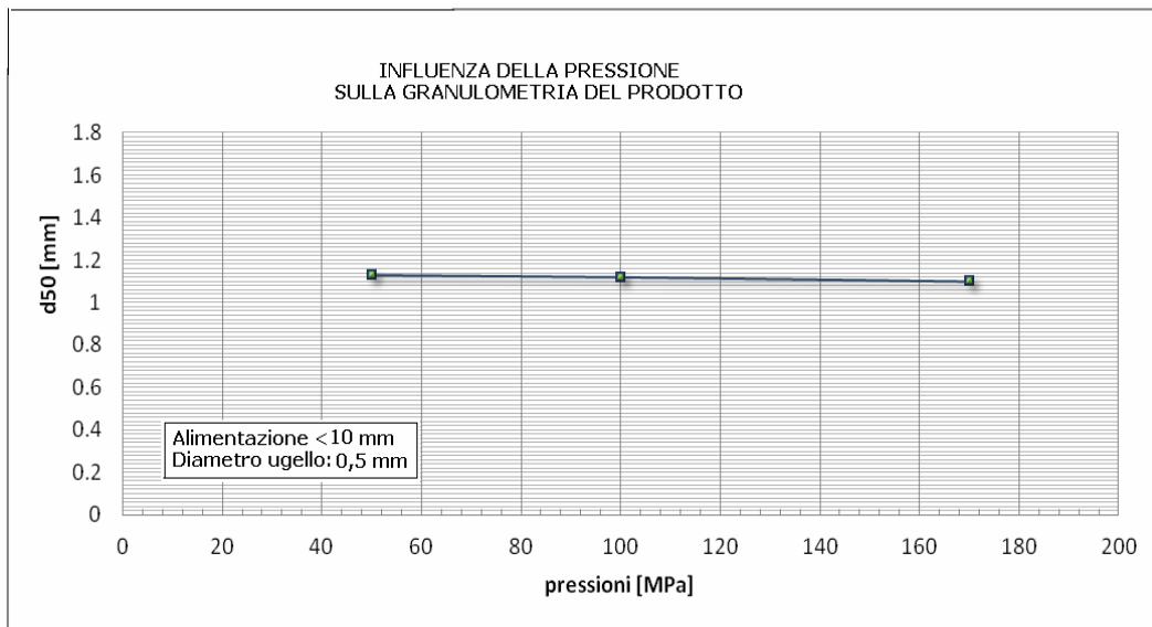
Figura 5.33. Influenza della pressione di generazione dei getti sul grado di finezza del prodotto rappresentato dal parametro d_{50}
