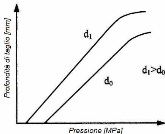
Figura 3.1 . Andamento della velocità di taglio in funzione della pressione
