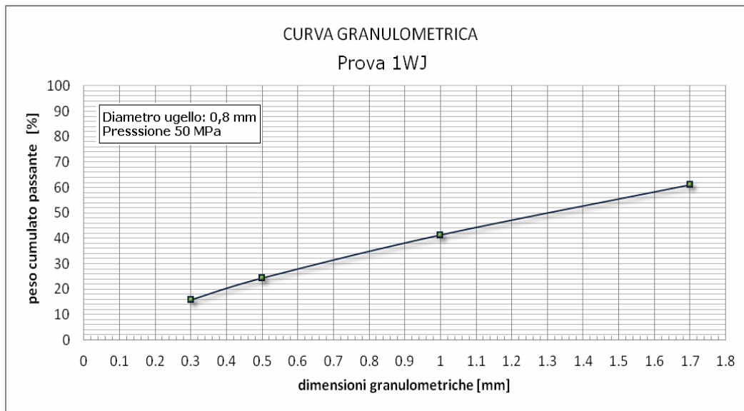
Figura 5.22. Distribuzione granulometrica del prodotto della prova 1WJ
