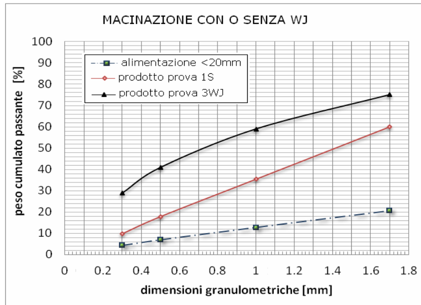
Figura 5.42. Confronto tra macinazione a secco e macinazione water jet. Diametro ugello 0,8 mm
