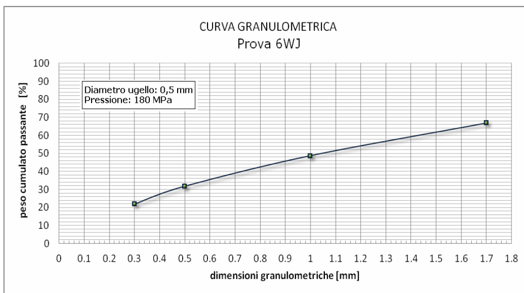
Figura 5.27. Distribuzione granulometrica del prodotto della prova 6WJ
