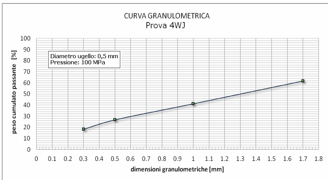
Figura 5.25. Distribuzione granulometrica del prodotto della prova 4WJ
