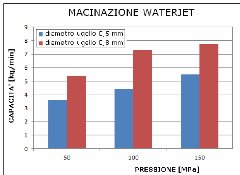
Figura 5.41. Capacità di trattamento in funzione della pressione e del diametro degli ugelli
