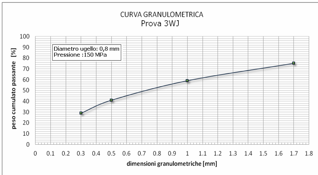
Figura 5.24. Distribuzione granulometrica del prodotto della prova 3WJ
