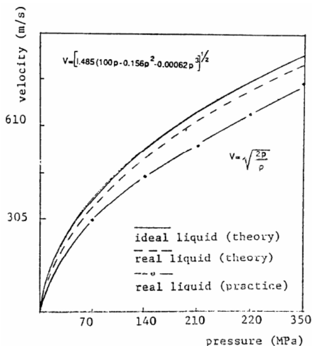
Figura 3.3. Velocità del getto d'acqua in funzione della pressione
