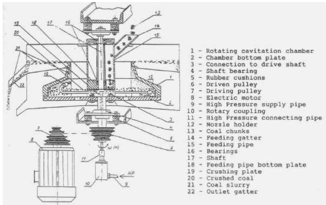
Figura 4.4. Apparecchio di comminuzione basato su fenomeni di cavitazione
