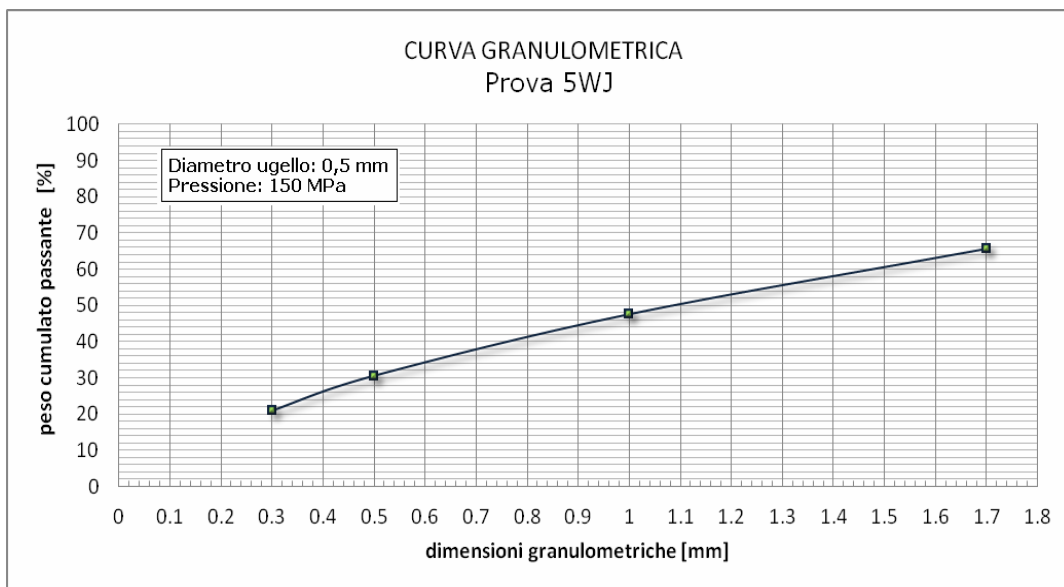
Figura 5.26. Distribuzione granulometrica del prodotto della prova 5WJ
