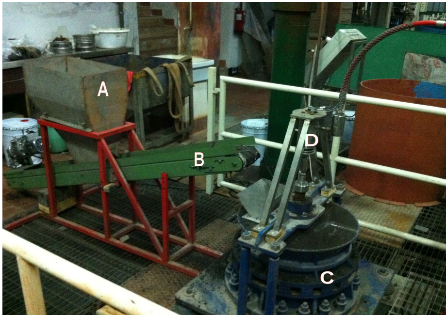
Figura 5.9. Impianto per il trattamento. A) Tramoggia di alimentazione; B) Nastro trasportatore; C) Mulino rotativo; D) Sistema d'immissione dell'acqua
