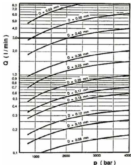
Figura 3.2. Variazione della portata in funzione della pressione e del diametro dell'ugello
