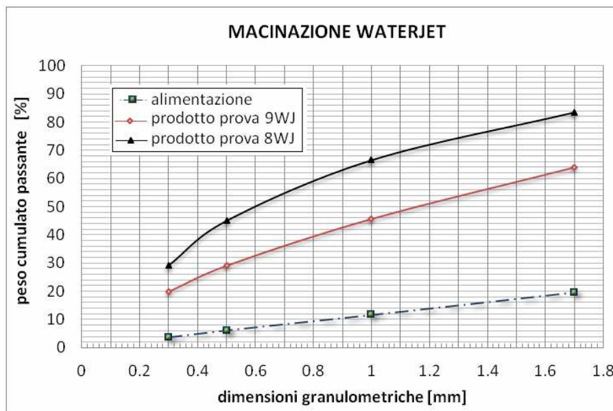
Figura 5.46. Influenza dell'impregnazione con acqua sul grado di finezza del prodotto.
