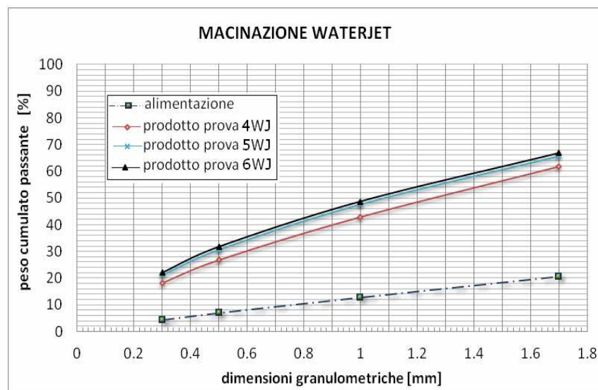
Figura 5.45. Influenza della pressione sul grado di finezza della macinazione.
