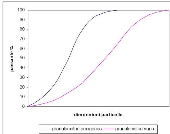
Figura 2.1 Esempi di curve granulometriche
