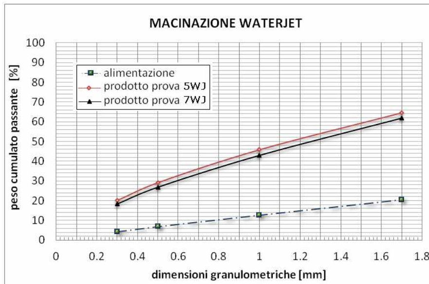
Figura 5.47. Influenza dell'impregnazione con acqua sul grado di finezza del prodotto. Granulometria alimentazione <20mm. Pressione 100 MPa. Diametro ugello 0,5 mm.
