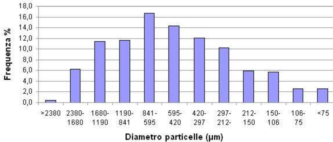
Figura 2.2 Grafico delle frequenze di un analisi granulometrica
