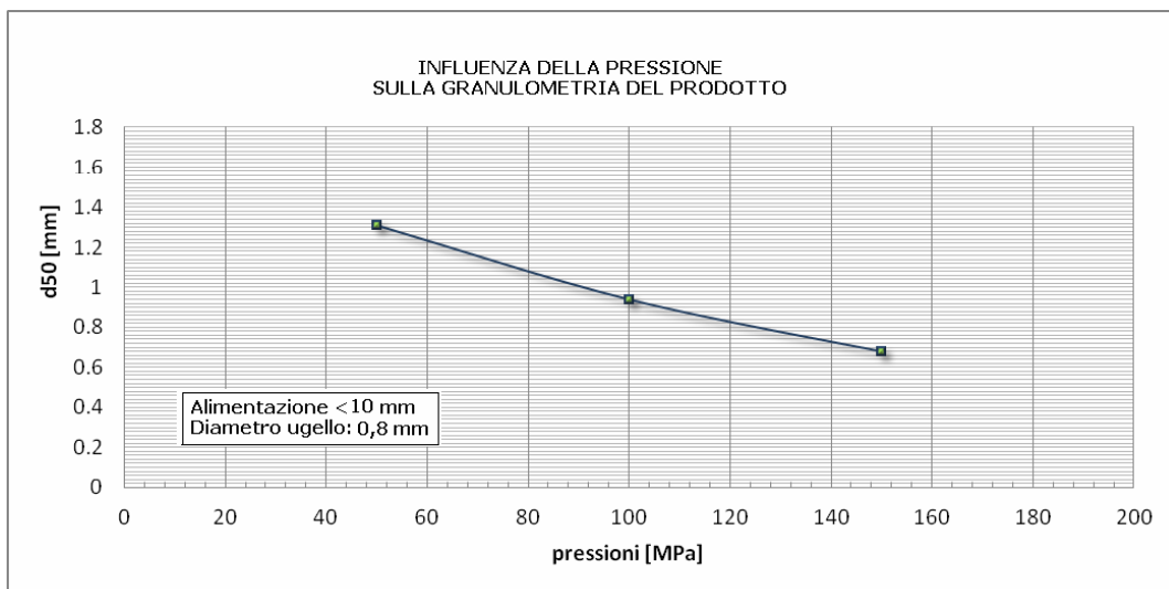
Figura 5.32. Influenza della pressione di generazione dei getti sul grado di finezza del prodotto rappresentato dal parametro d_{50}
