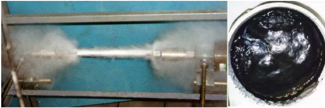
Figura 4.6. Effetto dei getti contrapposti nella micronizzazione del carbone.
