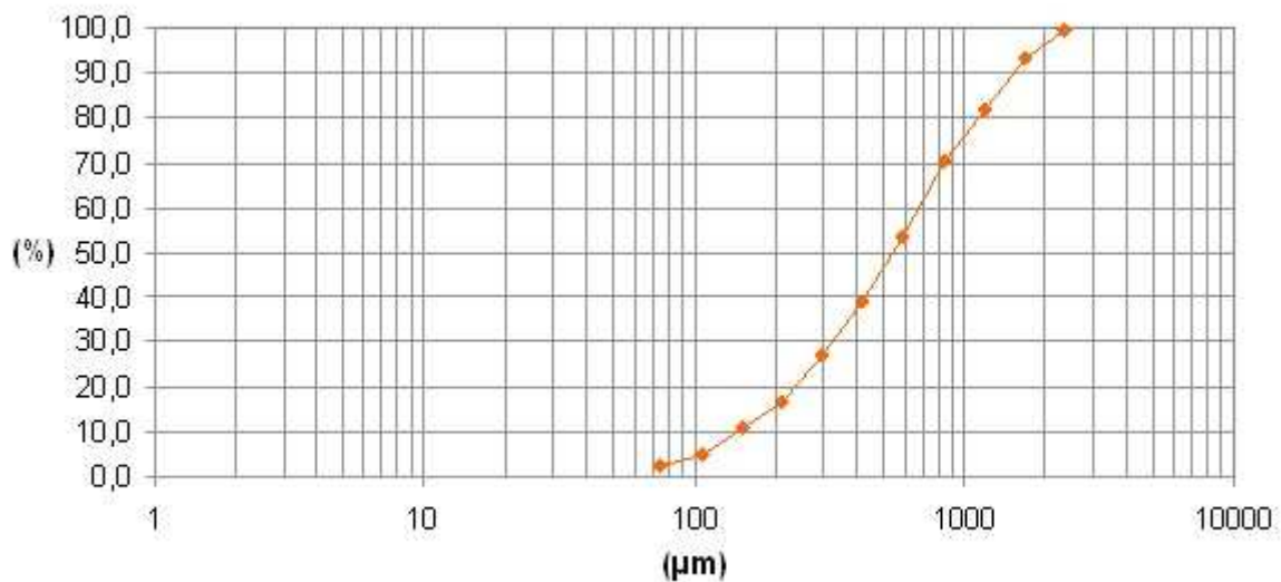
Figura 2.3. Curva cumulativa del passante
