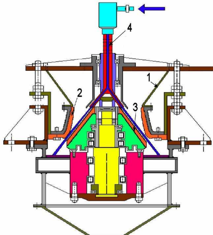
Figura 4.15. Schema del mulino rotativo con getti rotanti ad alta velocità (HERA)
