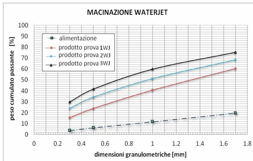
Figura 5.44. Influenza della pressione sul grado di finezza della macinazione.
