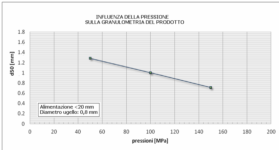
Figura 5.30. Influenza della pressione di generazione dei getti sul grado di finezza del prodotto rappresentato dal parametro d_{50}
