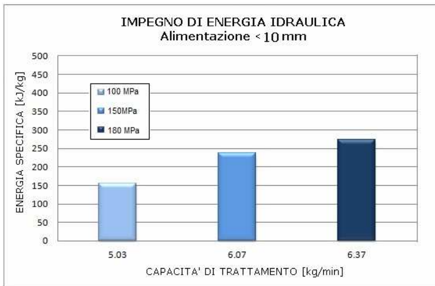
Figura 5.40. Confronto Energia specifica E_s in funzione della capacità di trattamento per diversi livelli di pressione. Diametro ugello: 0,5 mm
