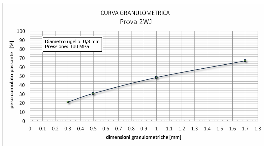
Figura 5.23. Distribuzione granulometrica del prodotto della prova 2WJ
