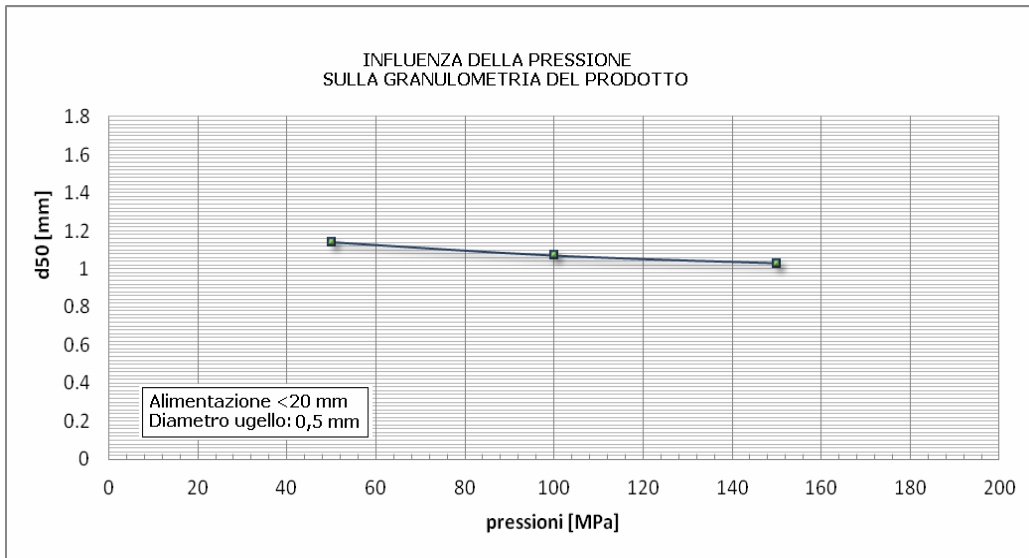
Figura 5.31. Influenza della pressione di generazione dei getti sul grado di finezza del prodotto rappresentato dal parametro d_{50}
