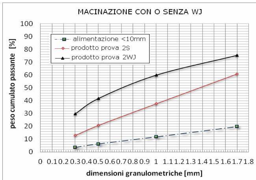
Figura 5.43. Confronto tra macinazione a secco e macinazione water jet. Diametro ugello 0,8 mm
