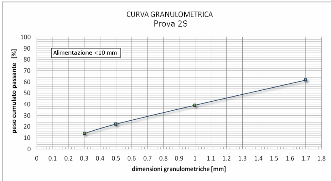
Figura 5.21. Distribuzione granulometrica del prodotto della prova 2S
