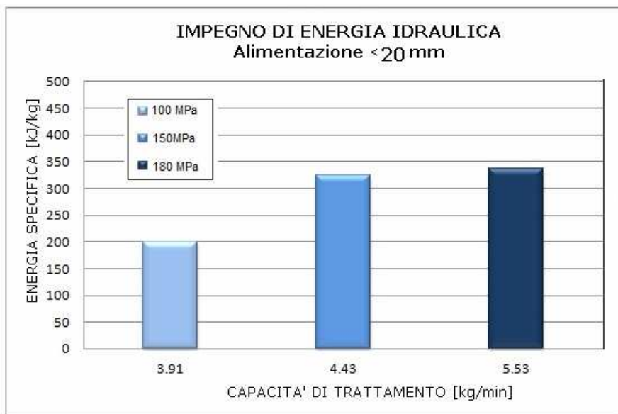
Figura 5.38. Confronto Energia specifica E_s in funzione della capacità di trattamento per diversi livelli di pressione. Diametro ugello: 0,5 mm
