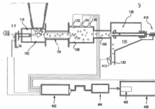
Figura 4.5. Schema dal mulino a getti contrapposti
