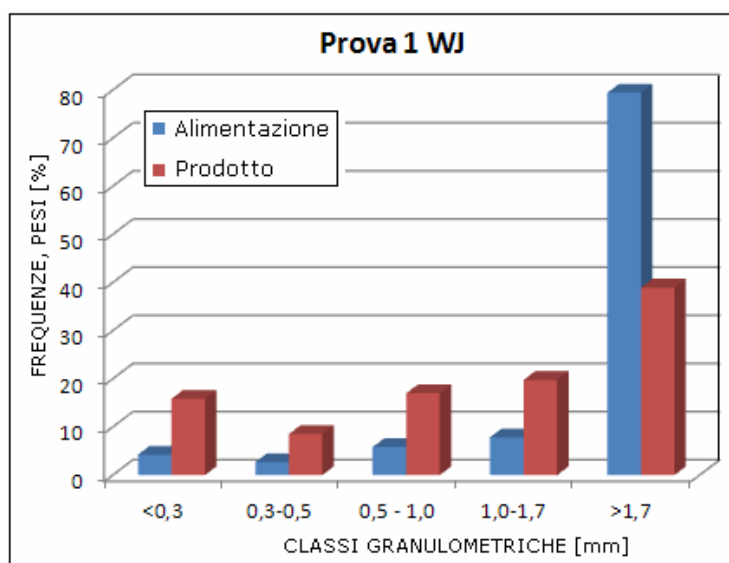
Figura 5.11. Istogramma della granulometria del prodotto della prova di macinazione con sinergia water jet 1W
