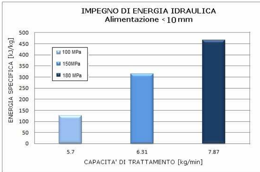
Figura 5.39. Confronto Energia specifica E_s in funzione della capacità di trattamento per diversi livelli di pressione. Diametro ugello: 0,8 mm
