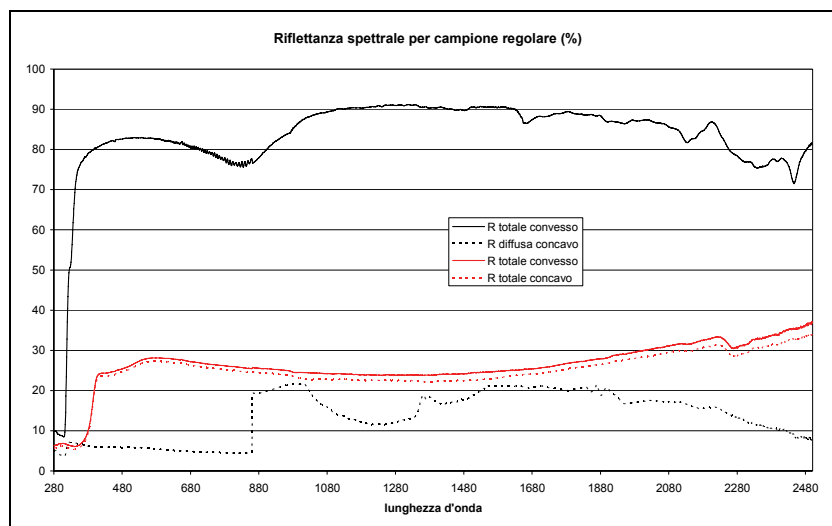
Figura 2. Curve spettrali del campione a comportamento speculare
