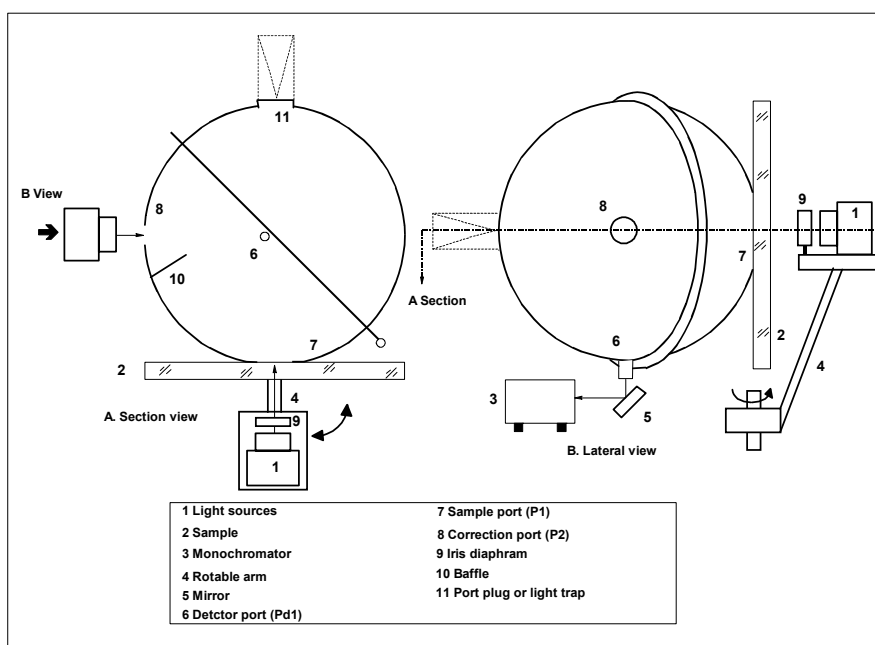
Figura 4 Schema di CATRAM, per misure con campione esterno
