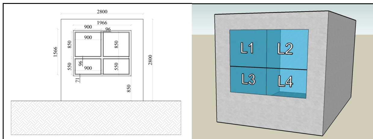
Figura 12 Prospetto sud di una cella di prova
