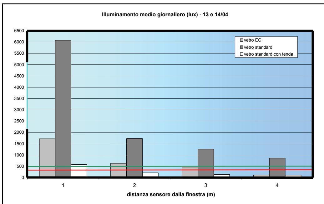
Figura 15 Illuminamento medio di C5 rispetto al vetro standard
