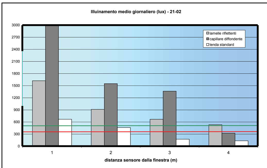
Figura 18 Illuminamento medio di C3 rispetto al vetro standard
