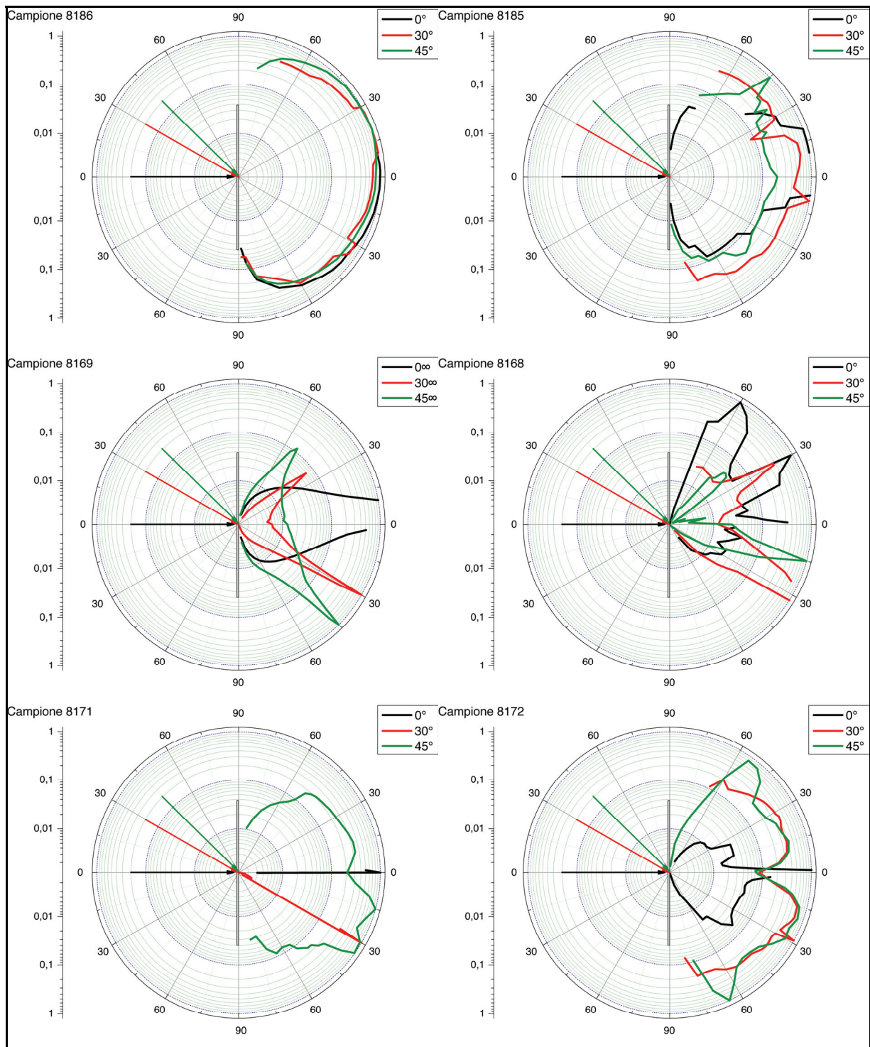
Figura 9 Distribuzione bidirezionale della trasmissione luminosa dei materiali testati
