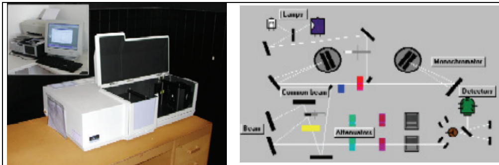
Figura 1. Immagine e schema ottico dello spettrofotometro Perkin Elmer 900
