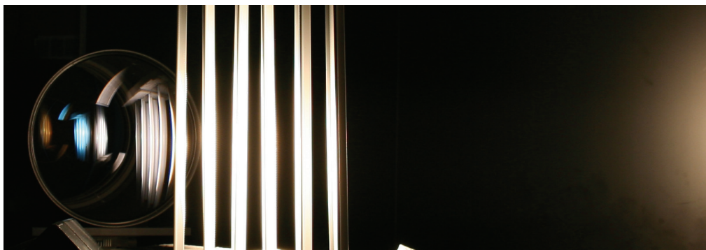
Figura 7 obiettivo telecentrico del goniofotometro
