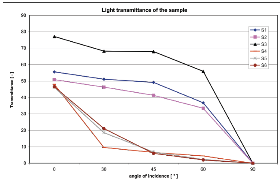
Figura 6 Trasmittanza angolare dei campioni selezionati
