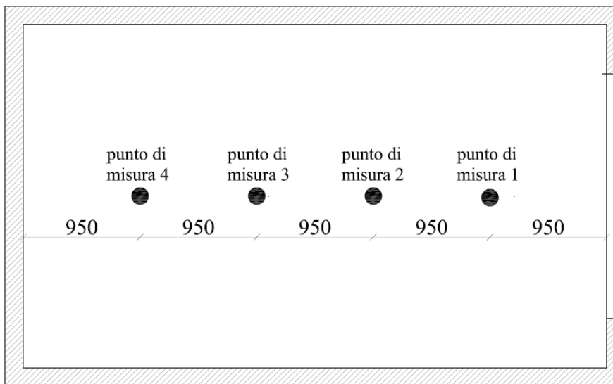
Figura 14 Pianta di una cella con posizione dei sensori di illuminamento
