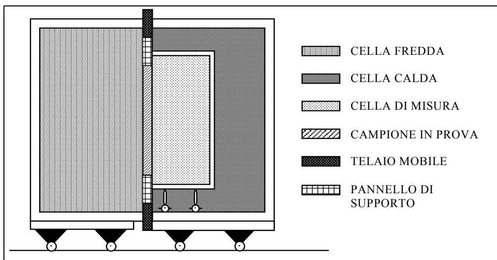
Figura 10. Schema della camera calda con anello di guardia
