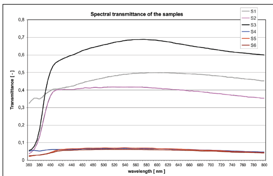
Figura 5 Trasmittanza spettrale dei campioni selezionati
