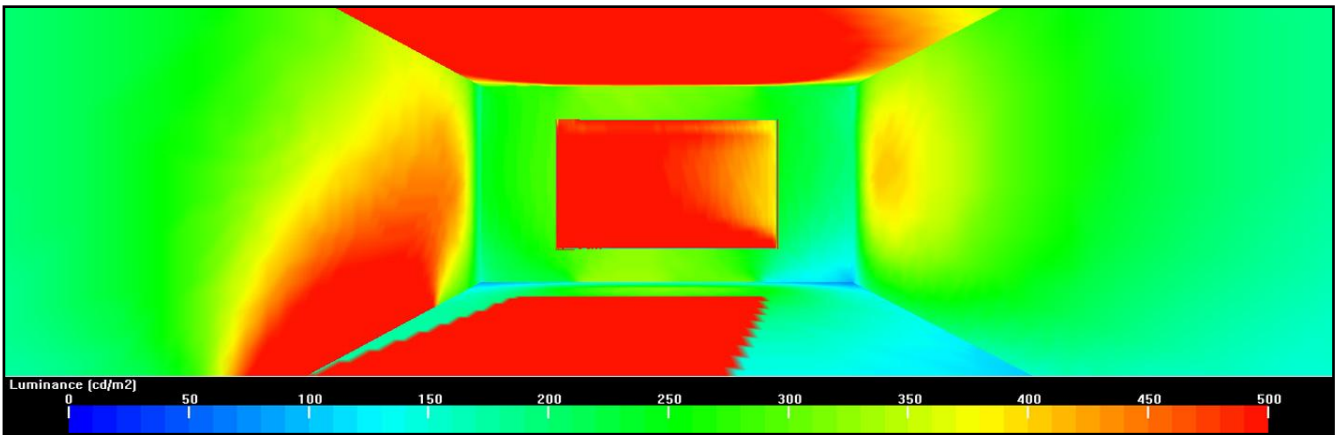
Figura 3.16. Luminanza
