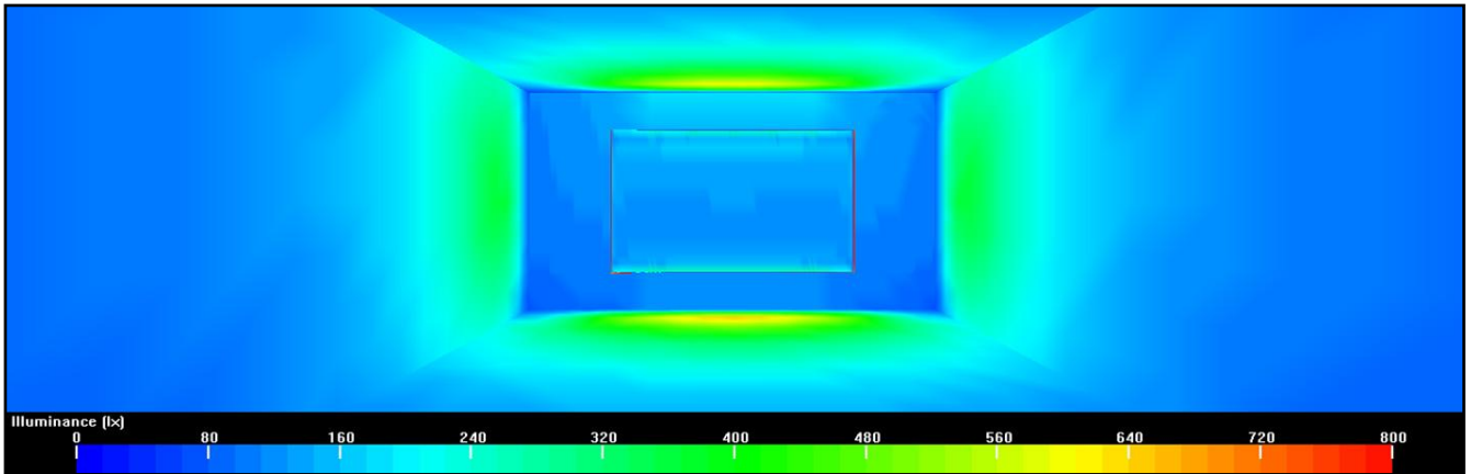
Figura 3.22. Illuminamento
