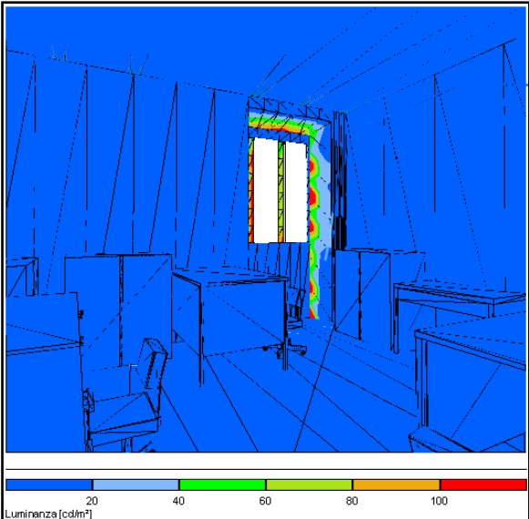
Figura 3.33. Luminanza
