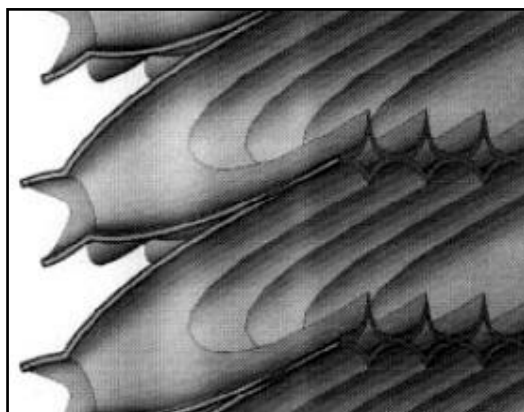
Figura 1.62. Sezione di uno schermo solare anidolico: modello tridimensionale elaborato al computer.
