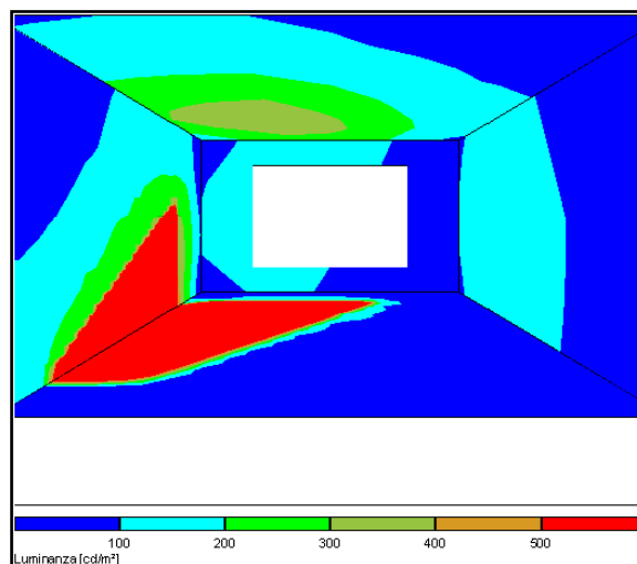
Figura 3.18. Luminanza
