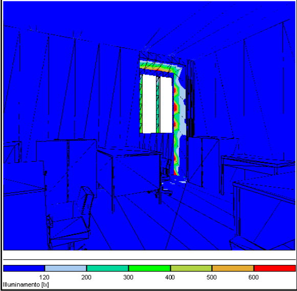
Figura 3.32. Illuminamento
