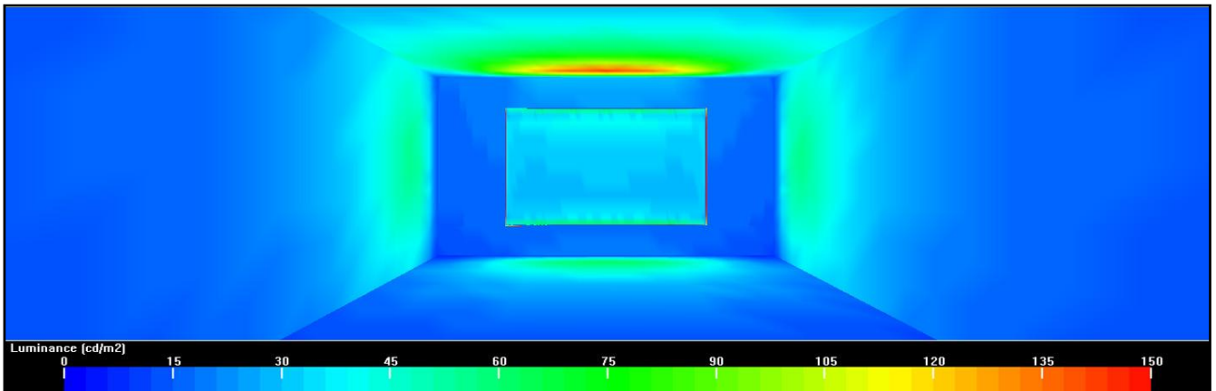
Figura 3.23. Luminanza
