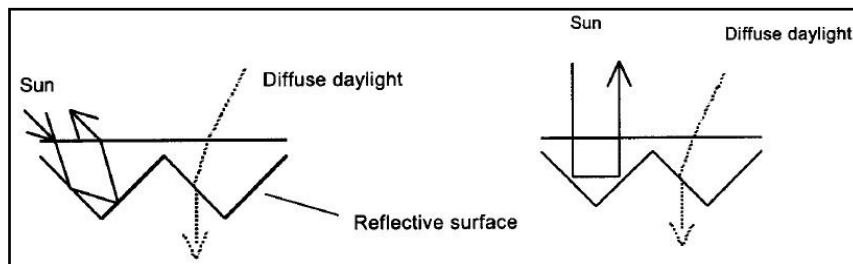
Figura 1.24. Comportamento della componente diretta e diffusa della luce diurna in un pannello prismatico che scherma la luce solare fisso (sinistra) e mobile (destra).
