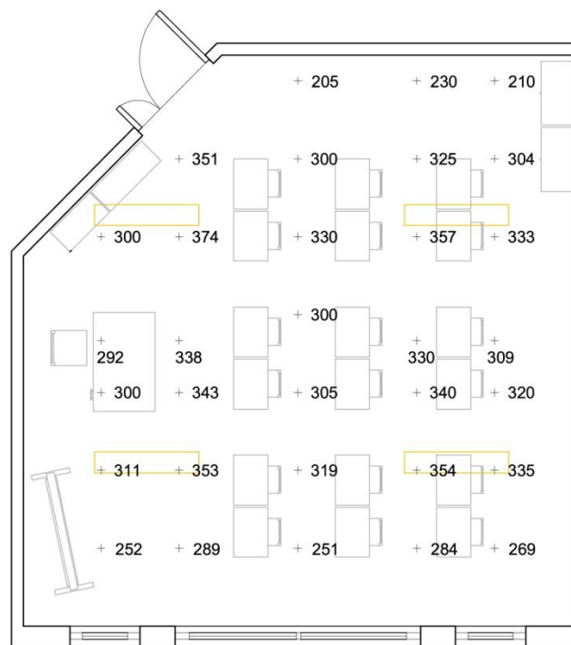
Figura 5.16. Pianta con l'indicazione dei valori di illuminamento sul piano di lavoro prodotti dalla sola illuminazione artificiale (in giallo sono indicati gli apparecchi e la loro disposizione)
