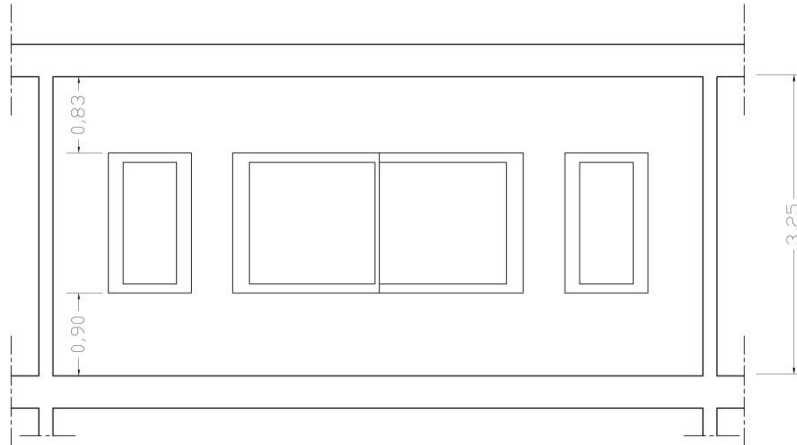
Figura 5.7. Sezione dell'aula oggetto delle misurazioni
