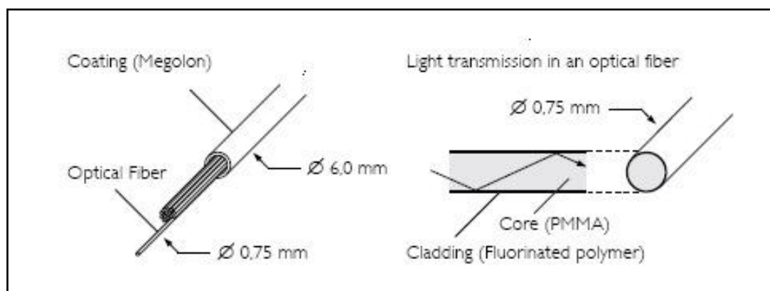
Figura 1.69. Schematizzazione di una fibra ottica e del suo funzionamento
