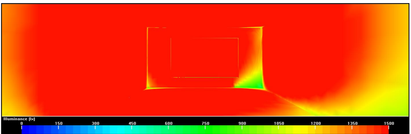
Figura 3.15. Illuminamento
