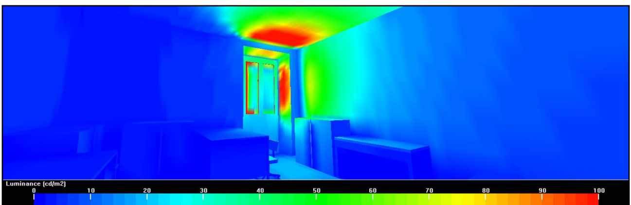
Figura 3.31. Luminanza
