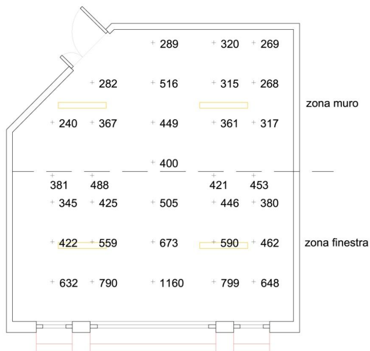
Figura 5.33. 21 Giugno Cielo Sereno ore 12, limite massimo di penetrazione della luce diurna: valori di illuminamento sul piano di lavoro in presenza dei sistemi di daylighting e PSALI
