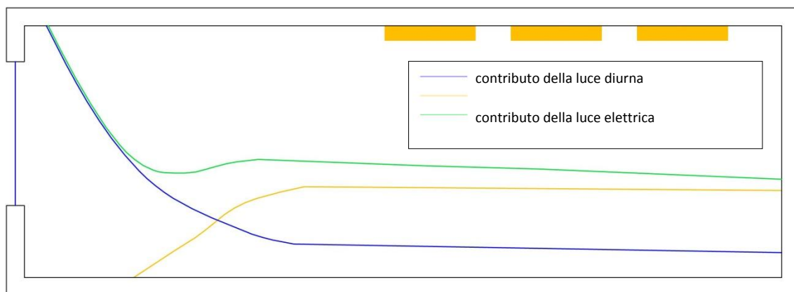
Figura 2.1. Schema PSALI.
