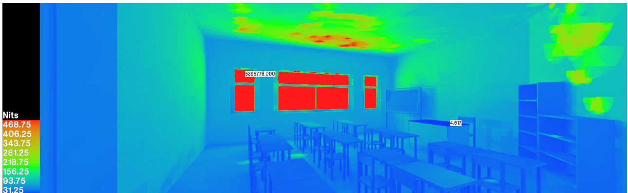
Figura 5.30. 21 Giugno Cielo Sereno ore 12: valori di luminanza in presenza del sistema di daylighting
