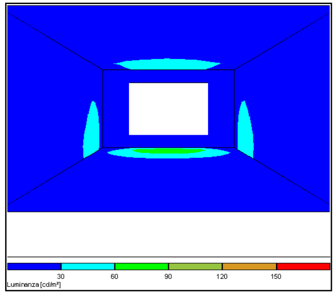
Figura 3.25. Luminanza
