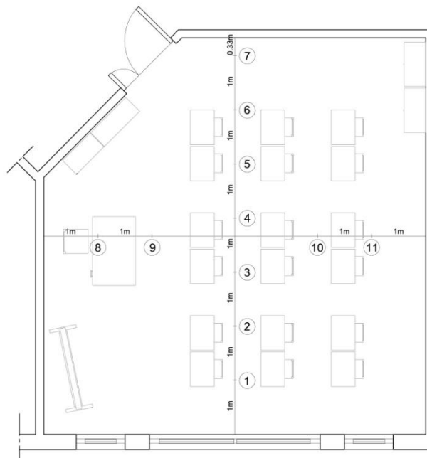
Figura 5.6. Pianta dell'aula oggetto delle misurazioni con l'indicazione dei punti di misura
