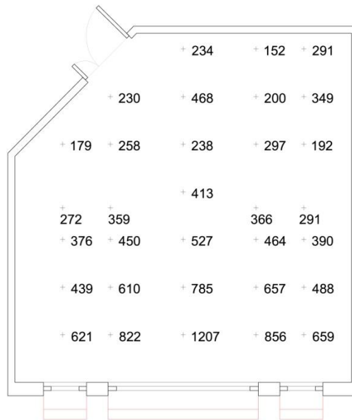
Figura 5.29. 21 Giugno Cielo Sereno ore 12: valori di illuminamento sul piano di lavoro in presenza del sistema di daylighting
