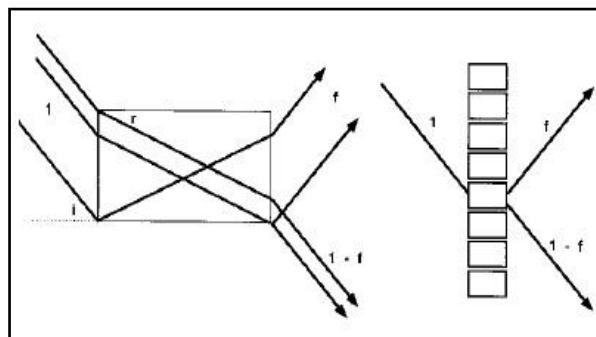
Figura 1.26. Schema di funzionamento di un pannello laser cut
