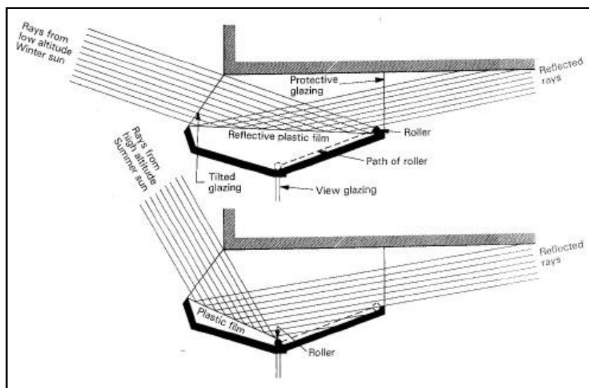
Figura 1.12. Schema di un light-shelf ad inseguimento solare
