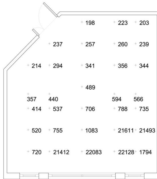
Figura 5.21. 21 Dicembre Cielo Sereno ore 12 Illuminamento sul piano di lavoro
