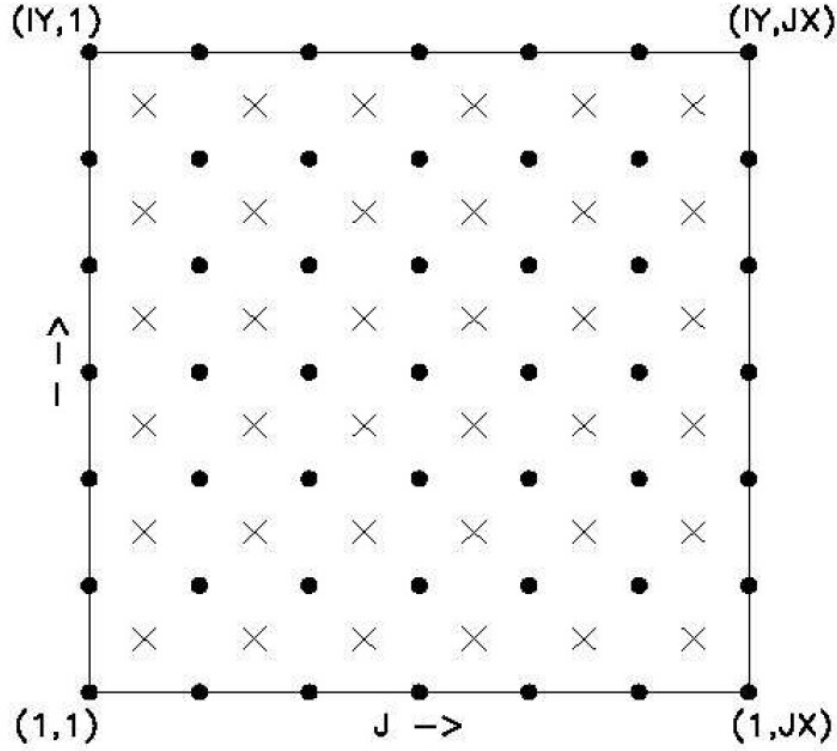
Figura 3: Rappresentazione schematica della griglia orizzontale sfasata di Arakawa-B. Sui punti indicati con il cerchio vengono definite le componenti della velocità orizzontale del vento, sulle croci le restanti variabili scalari.
