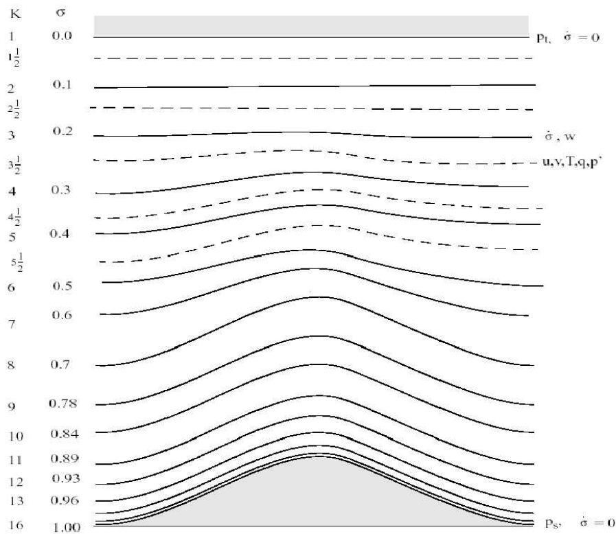
Figura 2: Rappresentazione schematica della struttura verticale del modello RegCM3 nella configurazione adottata per le previste simulazioni sul Mediterraneo
