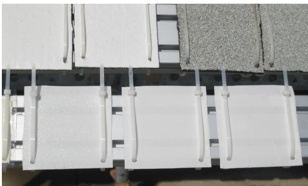
Figura 4. Dettaglio del fissaggio al supporto d'esposizione.
