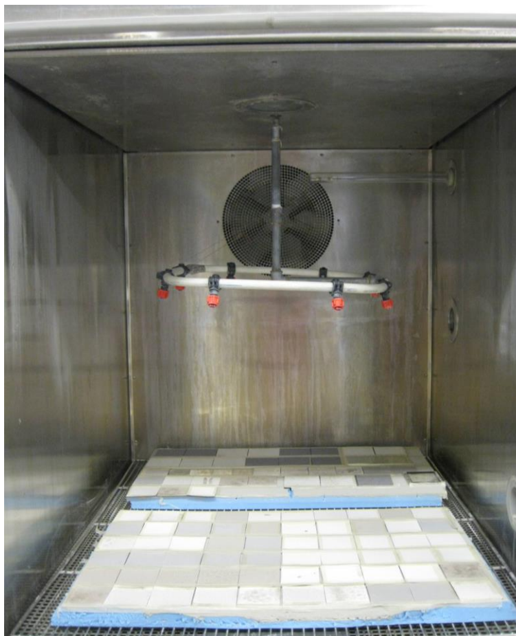
Figura 17. Cella climatica utilizzata al Politecnico di Milano e campioni posizionati all'interno (si tratta degli stessi prodotti esposti naturalmente).
