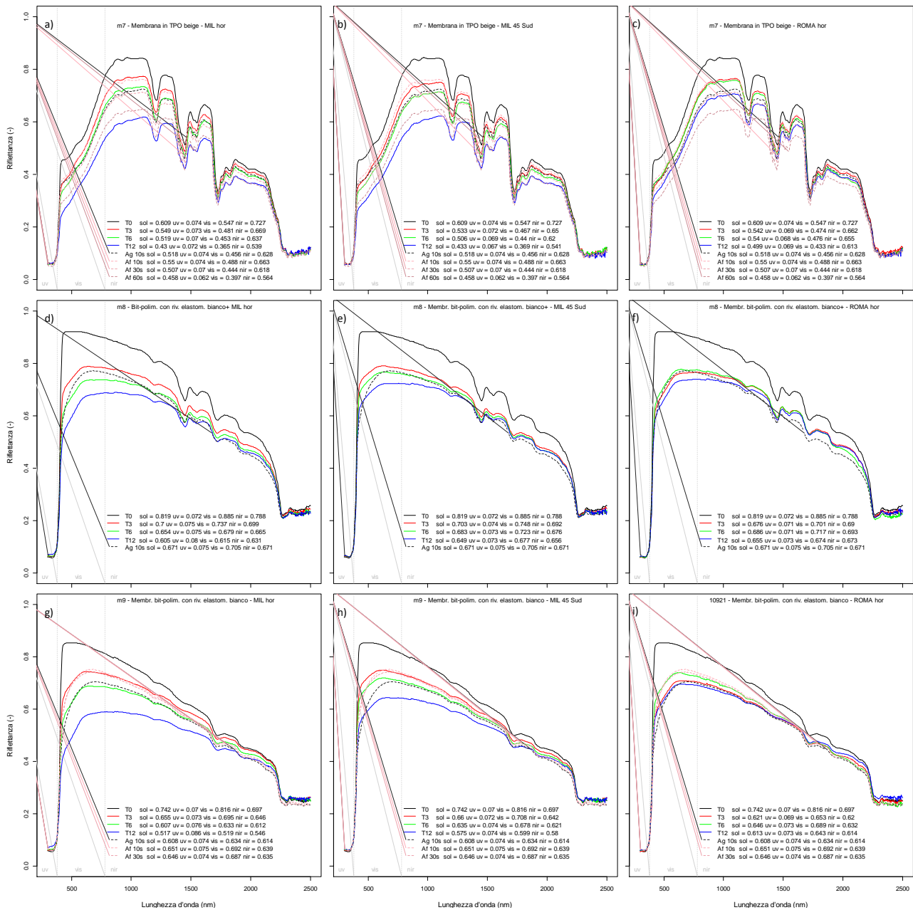
Figura 29. Riflettanza spettrale da 300-2500 nm e valori di riflettanza solare , UV, visibile e NIR calcolati secondo ISO 9050 per le membrane m7, m8, m9 dopo 3, 6 e 12 mesi a Milano (a bassa pendenza e 45° inclinato orientato a sud) e a Roma, e a seguito di sporcamento accelerato. Ag 10 s, Af 10 s, e Af 30 s, e riguardano, rispettivamente, campioni sottoposti a un ciclo di sporcamento di 10 secondi con la miscela generale (Ag 10 s), di 10 secondi (Af 10 s), e 30 secondi (Af 30 s) con la miscela rappresentativa per la Florida.
