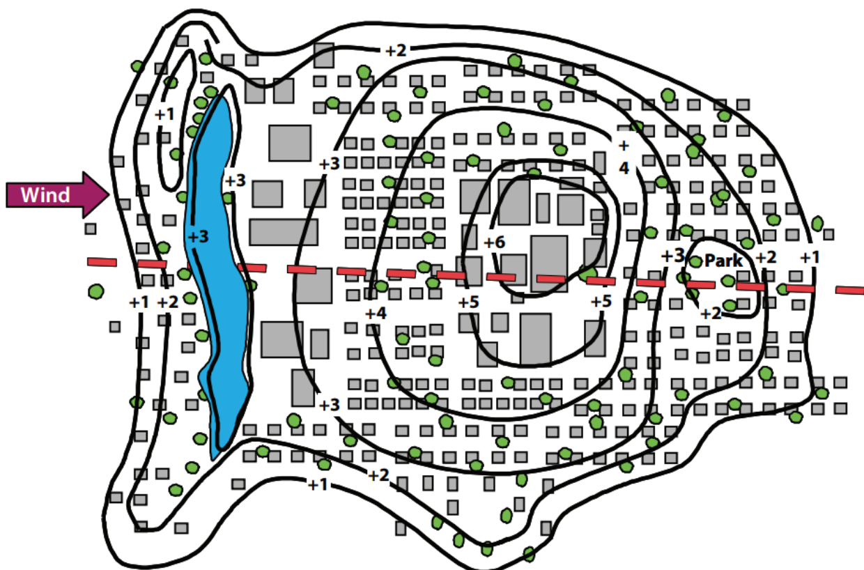
Figura 1: Mappa isoterma concettuale raffigurante una isola di calore urbana in atmosfera notturna (EPA, 2008)
