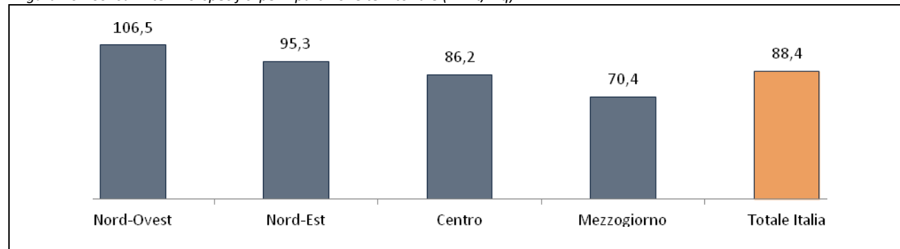
Figura 16 – Consumi termici specifici per ripartizione territoriale (kwht/mq)
