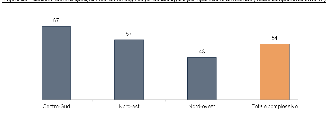
Figura 20 – Consumi elettrici specifici medi annui degli edifici ad uso ufficio per ripartizione territoriale (medie campionarie, kwh/m 2 )
