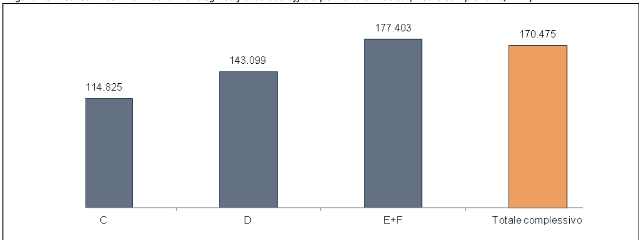
Figura 23 – Consumi termici medi annui degli edifici ad uso ufficio per zona climatica (medie campionarie, kwh )
