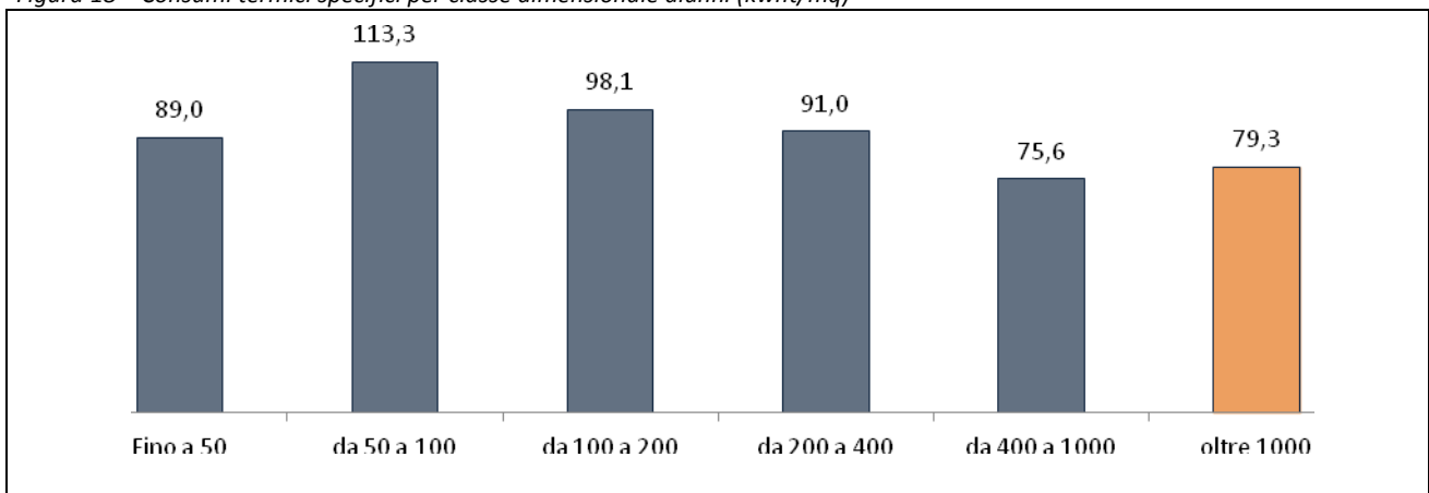
Figura 18 – Consumi termici specifici per classe dimensionale alunni (kwh/mq)
