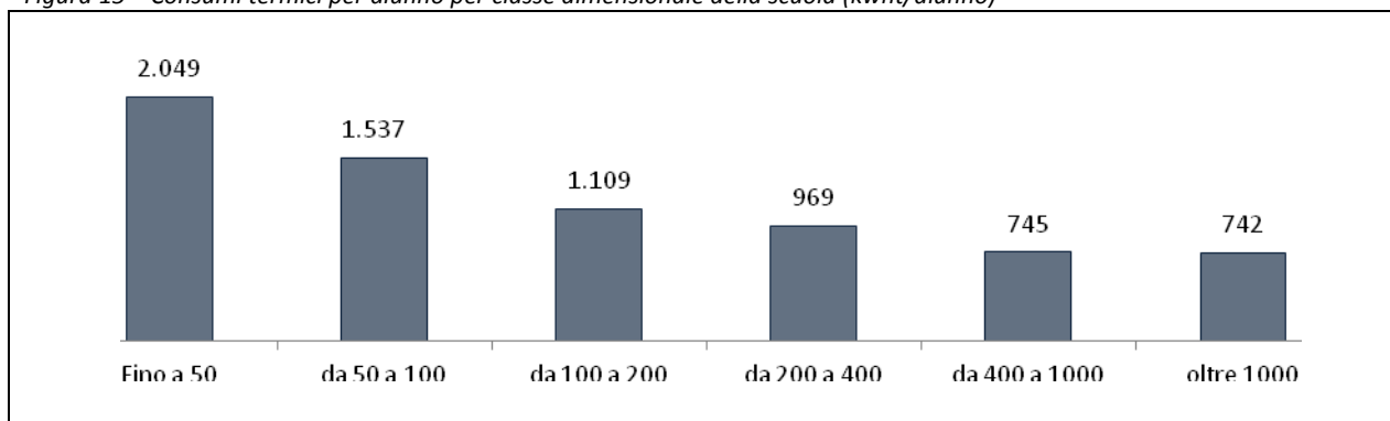
Figura 15 – Consumi termici per alunno per classe dimensionale della scuola (kwht/alunno)
