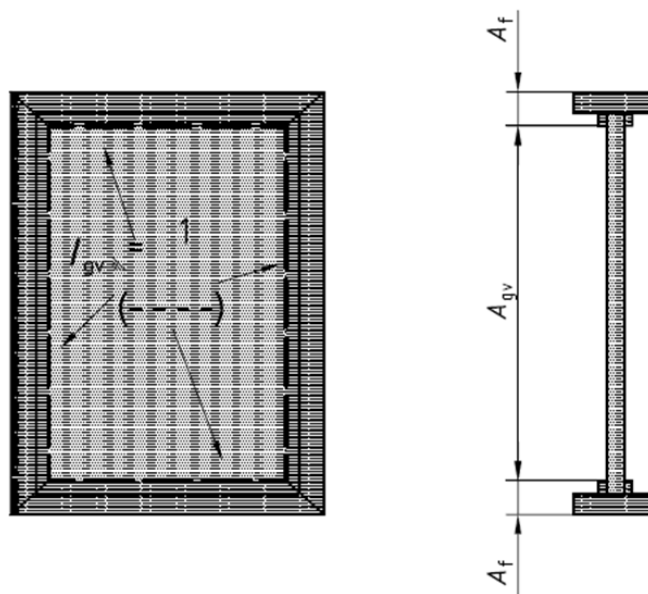
Figura 3. schematizzazione delle aree e del perimetro visibile dei componenti considerati nel calcolo della norma
