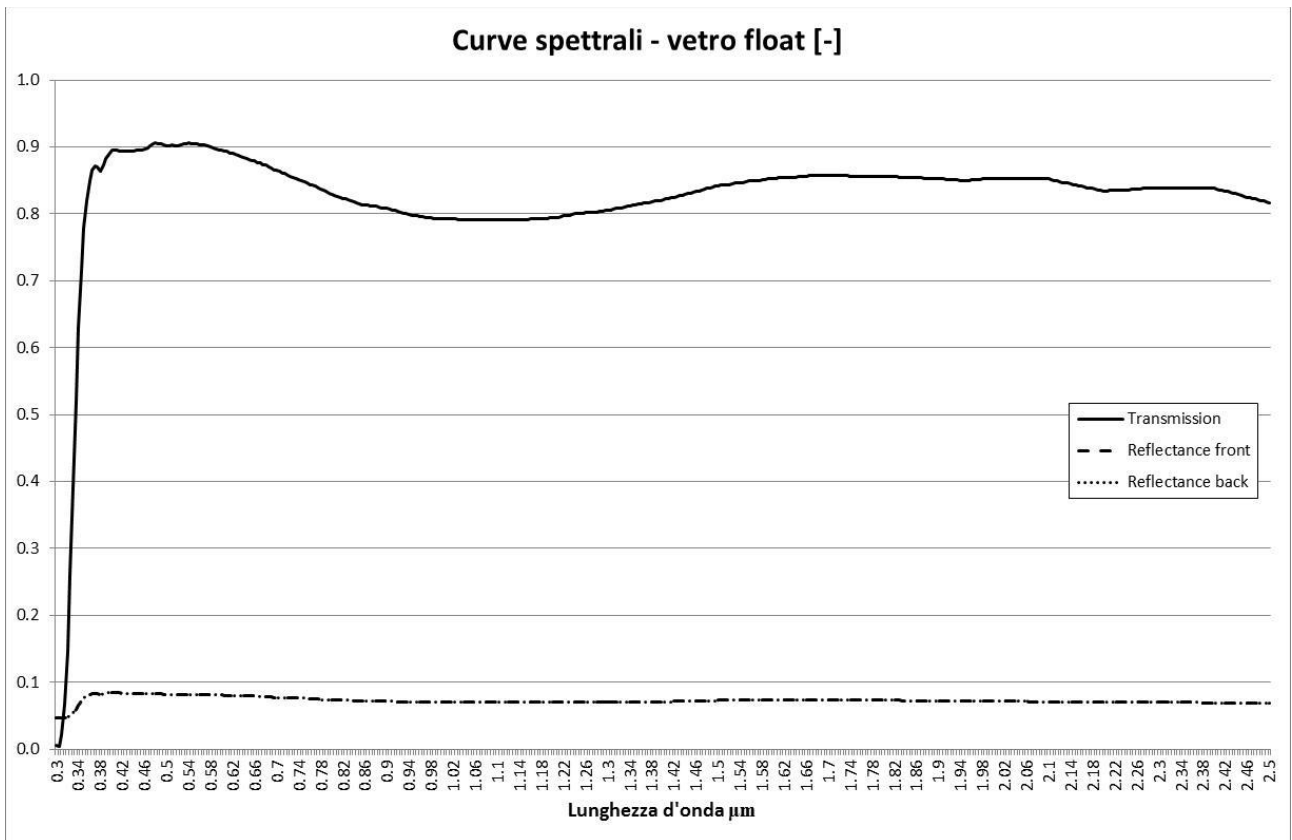
Figura 15. Caratterizzazione spettrale di un vetro float
