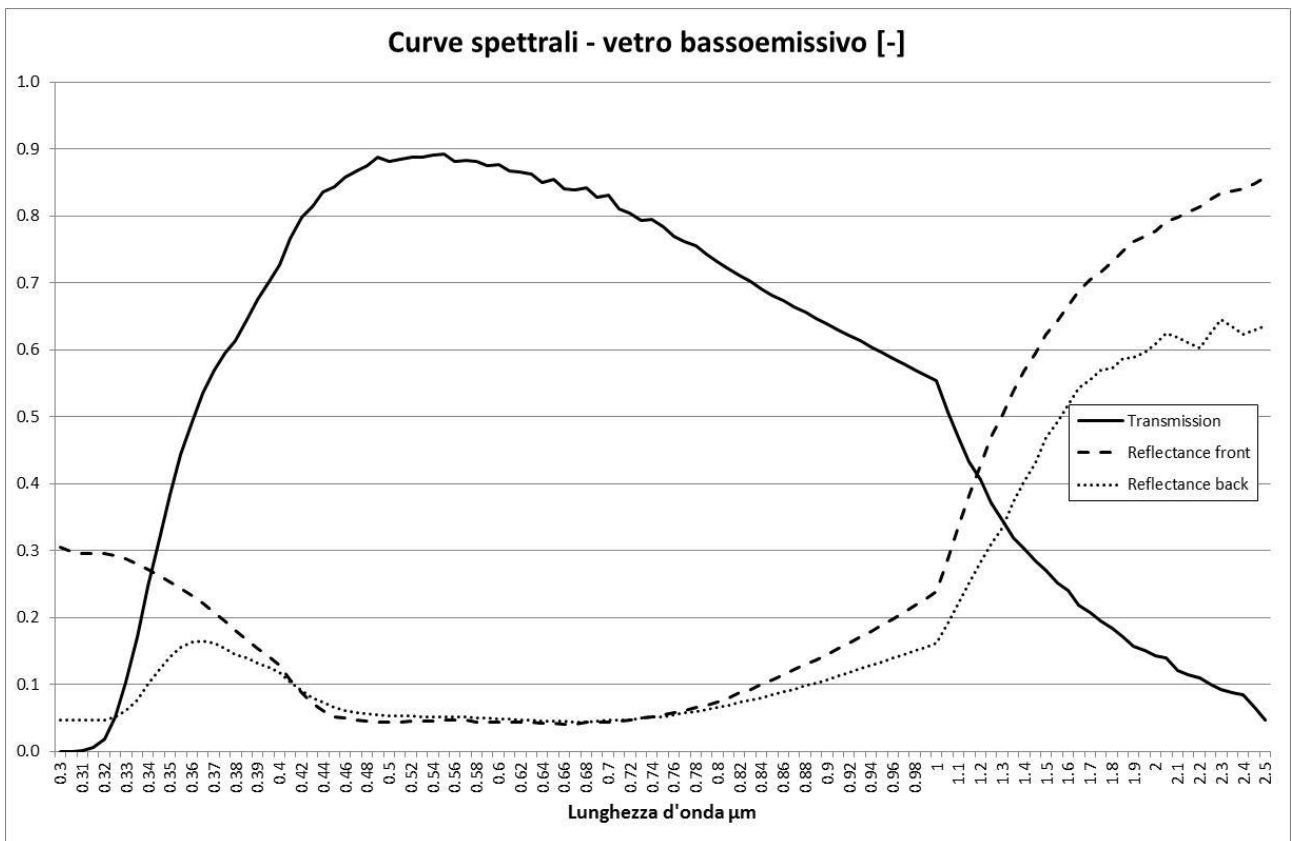
Figura 16. Caratterizzazione spettrale di un vetro bassoemissivo
