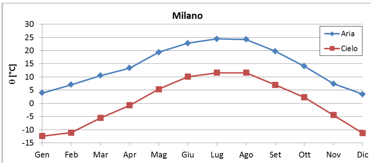
Figura 2.5 Temperatura media mensile dell'aria esterna e della volta celeste, città di Milano
