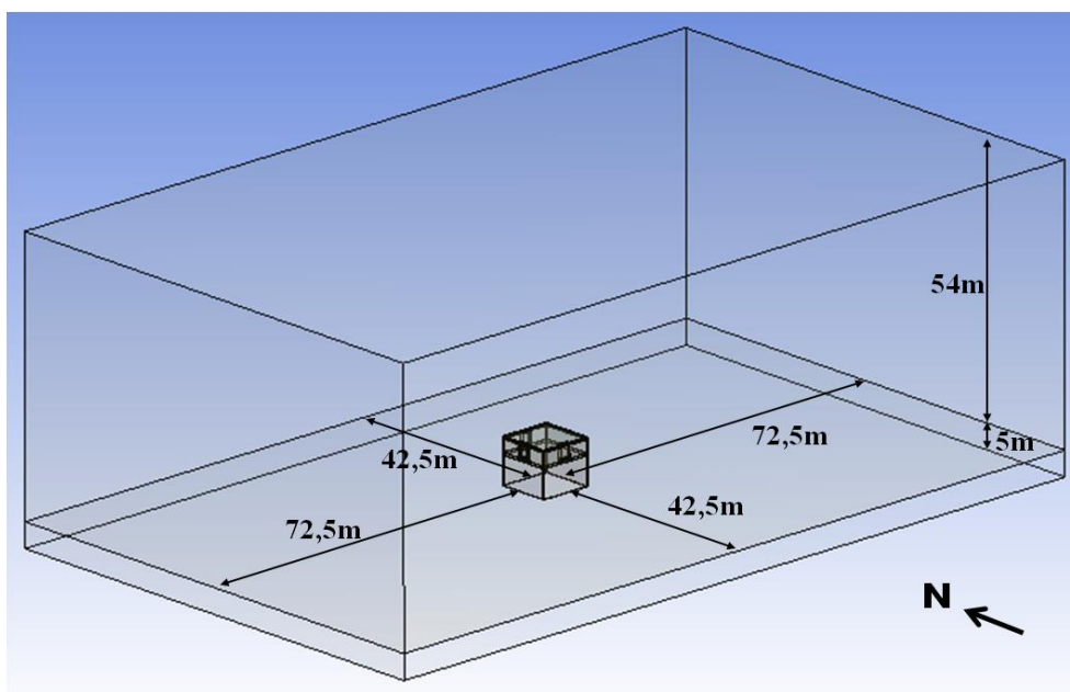
Figura 7: Rappresentazione del dominio di calcolo.
