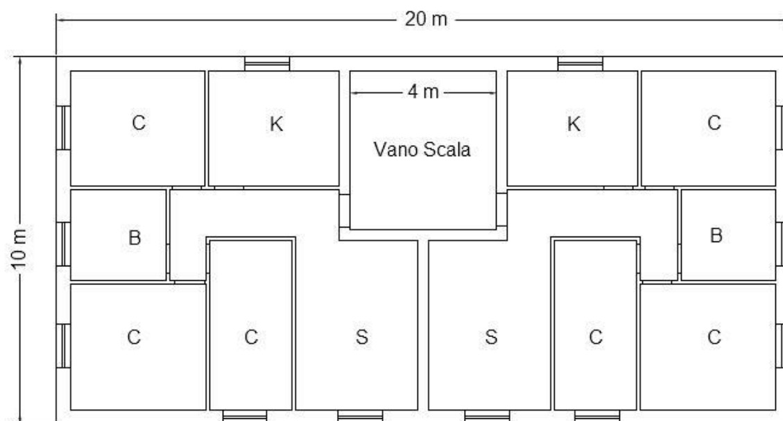
Figura 5: Pianta dell'edificio di riferimento.
