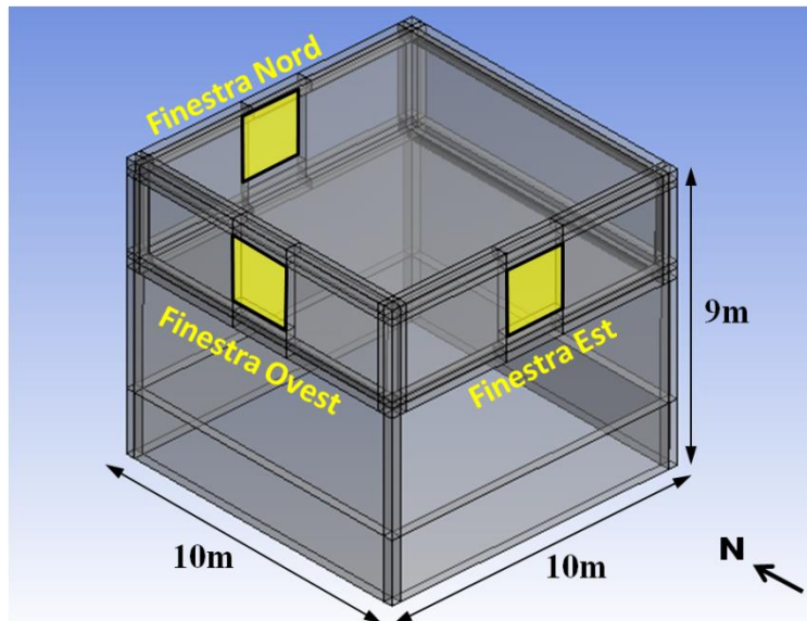
Figura 6: Geometria dell'edificio per l'analisi termo-fluidodinamica.
