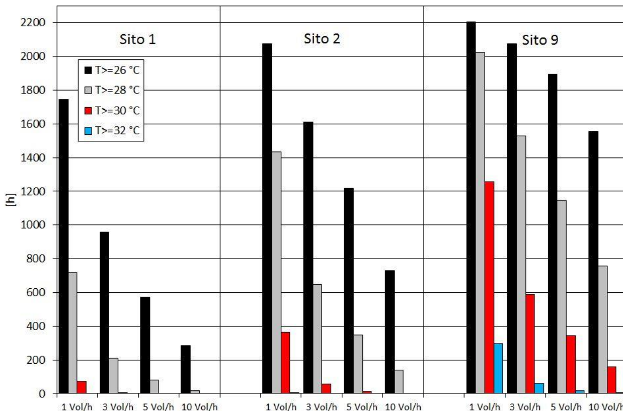
Figura 16: Distribuzione cumulativa delle temperature operative al variare dei ricambi orari per tre siti, configurazione non isolata.
