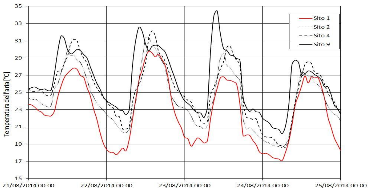
Figura 9: Andamento delle temperature orarie 21/08/2014 ore 00:00 - 25/08/2014 ore 00:00.
