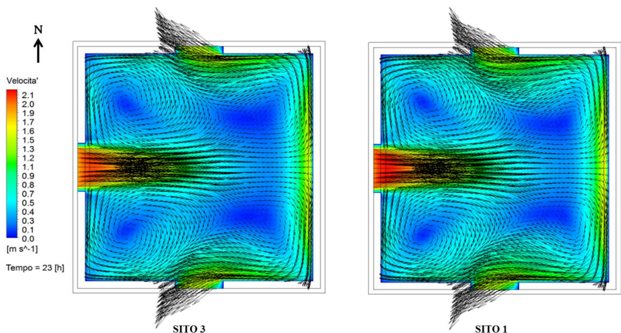
Figura 18: Distribuzione della velocità dell'aria all'interno della casa ad un'altezza di 1,5 metri.
