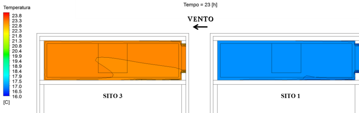
Figura 20: Confronto della temperatura dell'aria interna alla casa fra il sito 1 e 3 alle 23:00.
