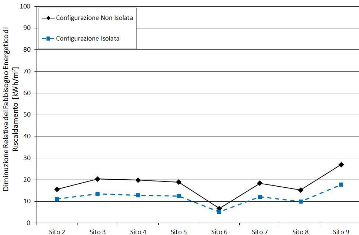
Figura 13: Diminuzione relativa del fabbisogno di riscaldamento.
