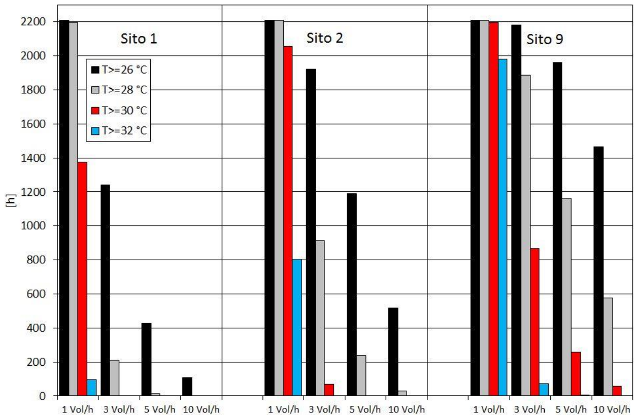
Figura 17: Distribuzione cumulativa delle temperature operative al variare dei ricambi orari per tre siti, configurazione isolata.
