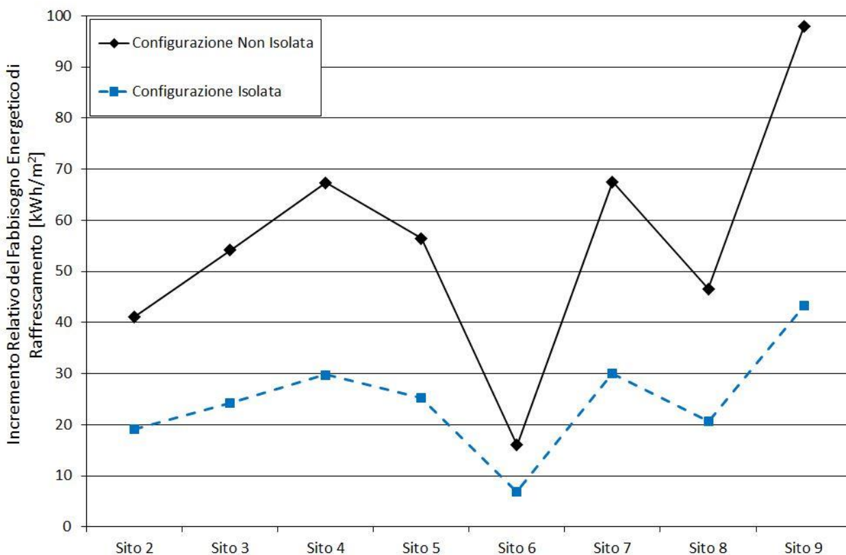
Figura 14: Incremento relativo del fabbisogno di raffrescamento.
