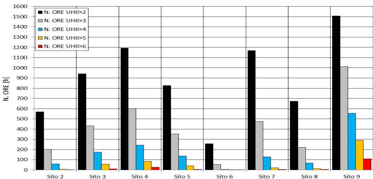
Figura 12: Distribuzione cumulativa dell'intensità dell'isola di calore (riferimento sito 1) nel periodo 01/07/2014 - 20/09/2014.
