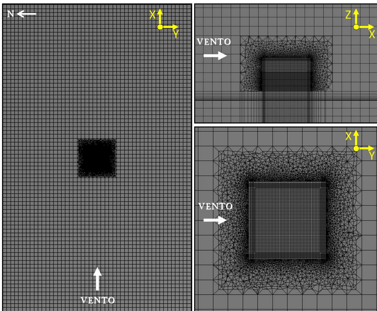
Figura 8: Discretizzazione del dominio di calcolo.
