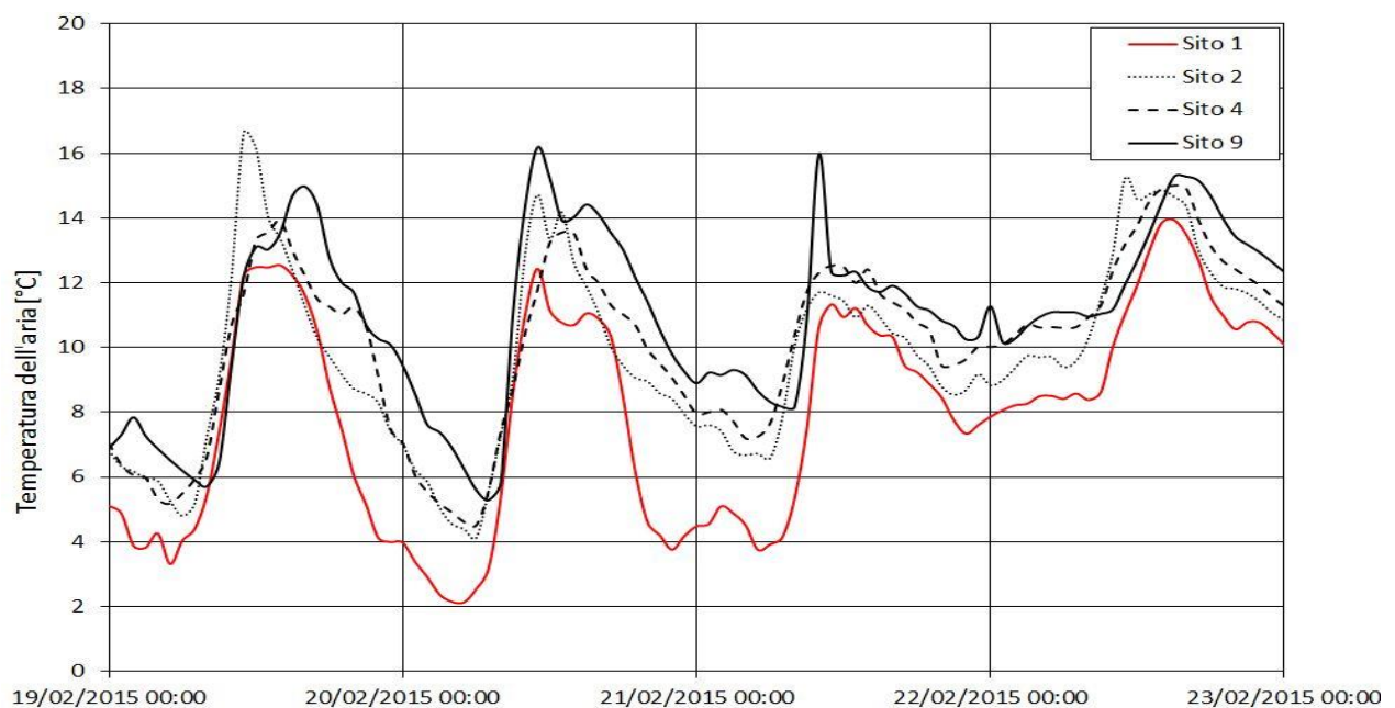
Figura 10: Andamento delle temperature orarie 19/02/2015 ore 00:00 - 23/02/2015 ore 00:00.
