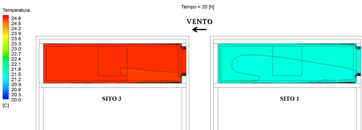
Figura 19: Confronto della temperatura dell'aria interna alla casa fra il sito 1 e 3 alle 20:00.
