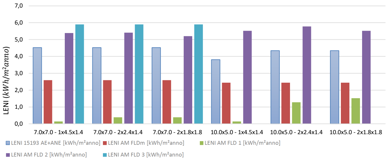
Figura 8. Confronto tra i valori del LENI per le aule scolastiche situate idealmente a Milano (RAI 1/8)
