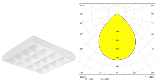
Figura 2. Corpo illuminante previsto nelle aule e relativa curva fotometrica con sorgente LED
