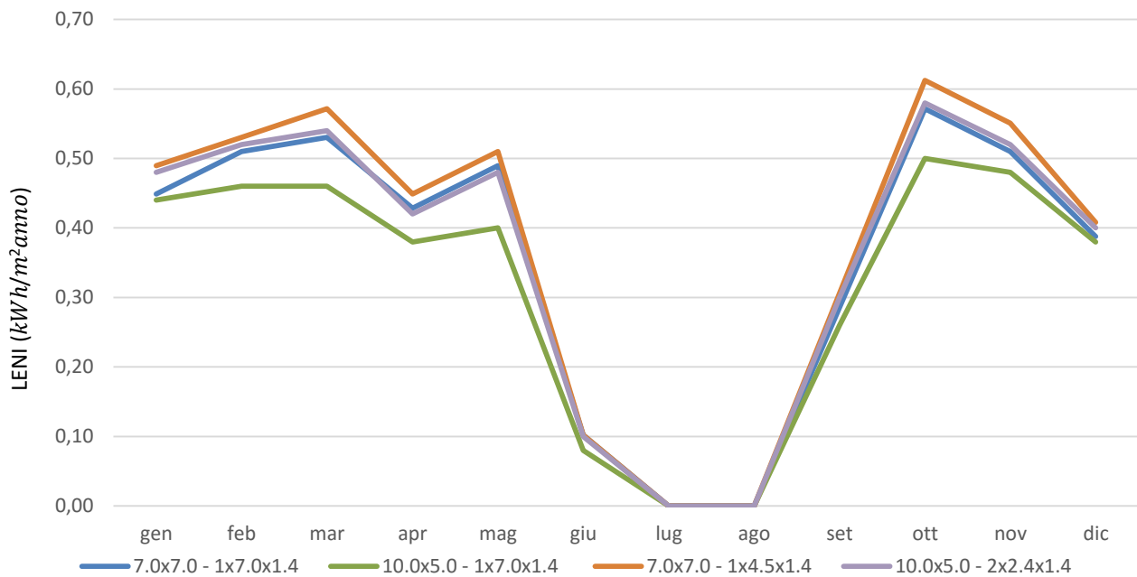
Figura 18. Aule scolastiche (Roma)- LENI mensile calcolato con il Mcc
