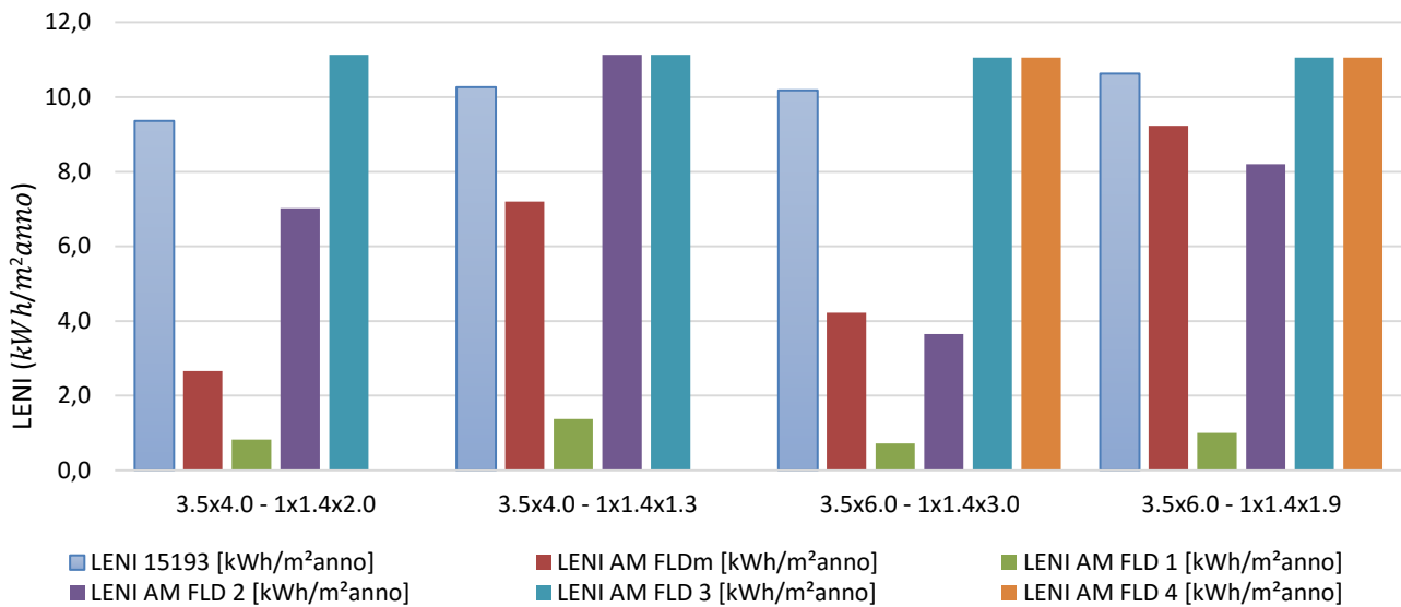
Figura 15. Confronto tra i valori del LENI per gli uffici situati idealmente a Palermo
