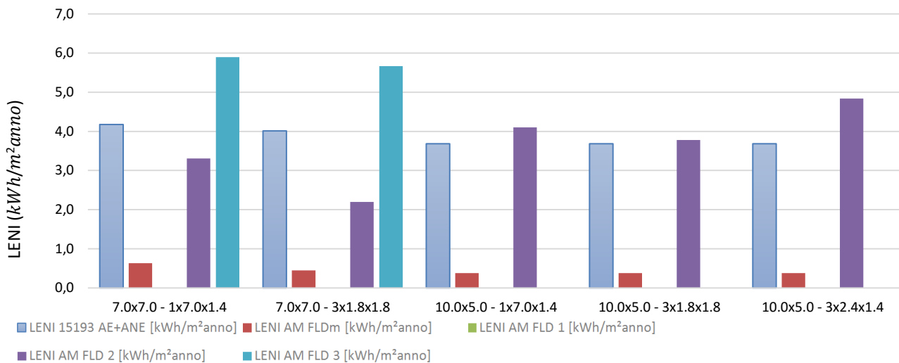
Figura 11. Confronto tra i valori del LENI per le aule scolastiche situate idealmente a Palermo ( RAI 1/5)
