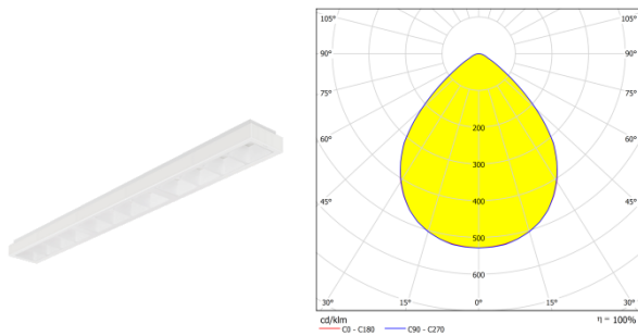
Figura 3. Corpo illuminante installato negli uffici (casi 1 e 3) e curva fotometrica con sorgente LED
