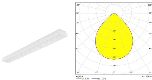
Figura 4. Corpo illuminante installato negli uffici (casi 2 e 4) e curva fotometrica con sorgente LED
