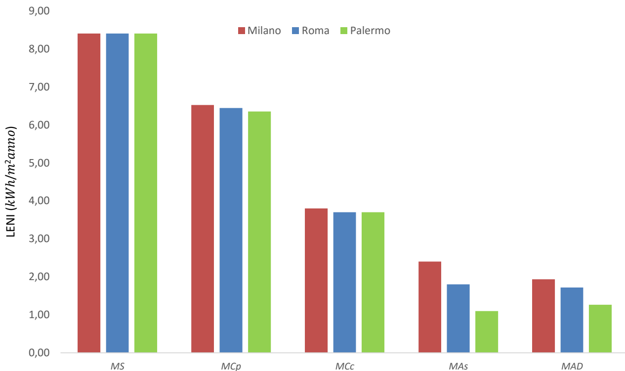
Figura 25. Confronto tra diversi metodi di calcolo del LENI - aula 10.0 x 5.0 m con una finestra a nastro di dimensione 4.5 x 1.4 m, RAI 1/8, calcolato per \bar{E}_m di 300 lux
