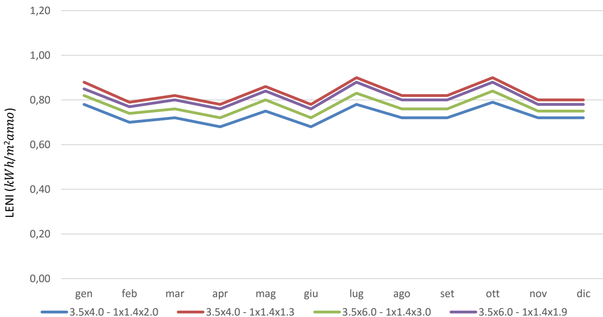
Figura 16. Uffici (ROMA) - LENI mensile calcolato con il Mcc
