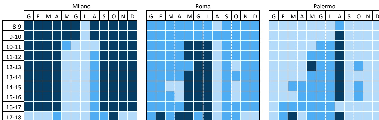
Figura 28. Componente diffusa dei livelli di illuminamento al suolo (satel-light.com): il colore più chiaro corrisponde al valore più alto tra le 3 località
