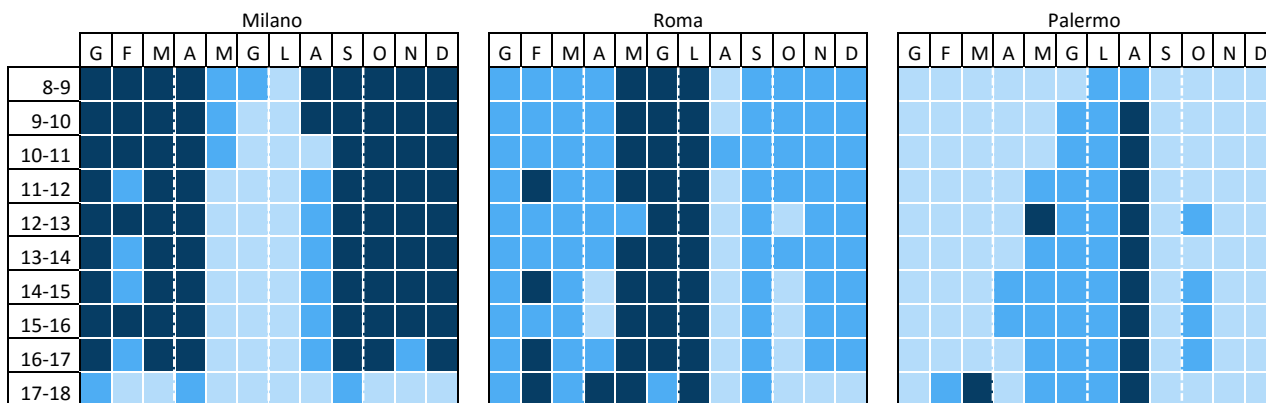
Figura 29. Componente diffusa della radiazione solare al suolo (satel-light.com): il colore più chiaro corrisponde al valore più alto tra le 3 località
