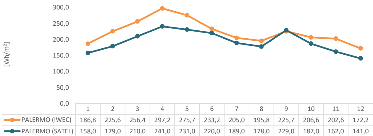
Figura 33. Confronto tra i dati di radiazione diffusa (valore medio mensile) dei file IWECC e di satel-light.com a Palermo tra le 12 e le 13
