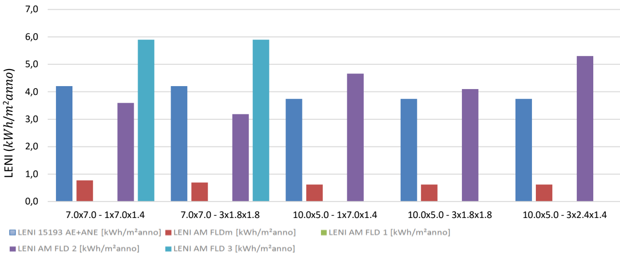
Figura 9. Confronto tra i valori del LENI per le aule scolastiche situate idealmente a Roma (RAI 1/5)
