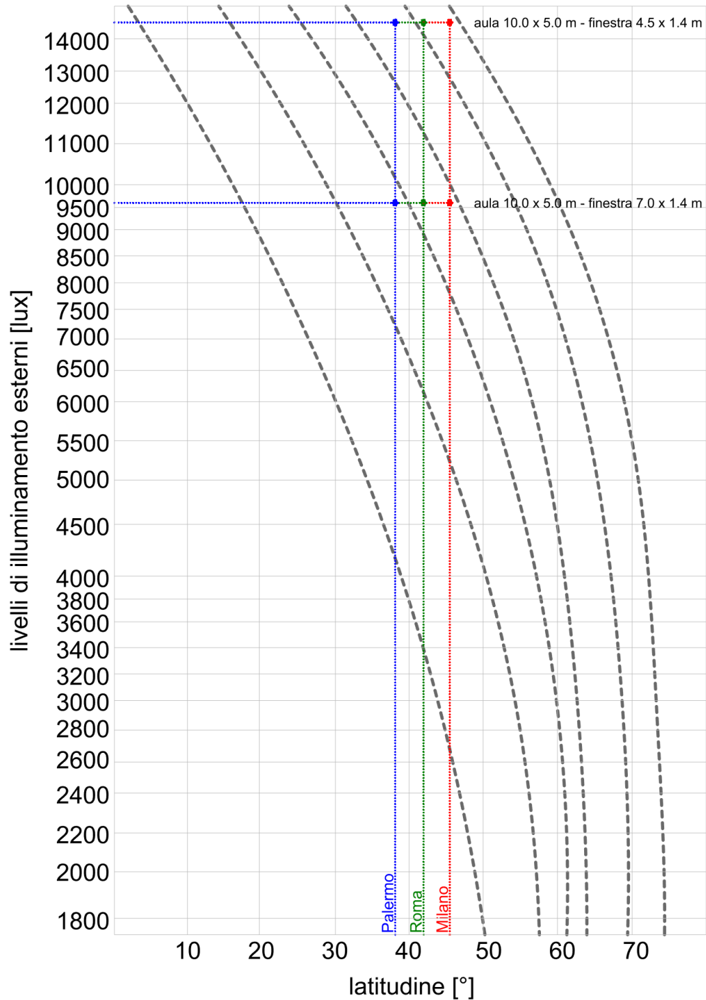
Figura 23. Diagrammi di Dresler con indicazione della latitudine delle tre località prese in esame
