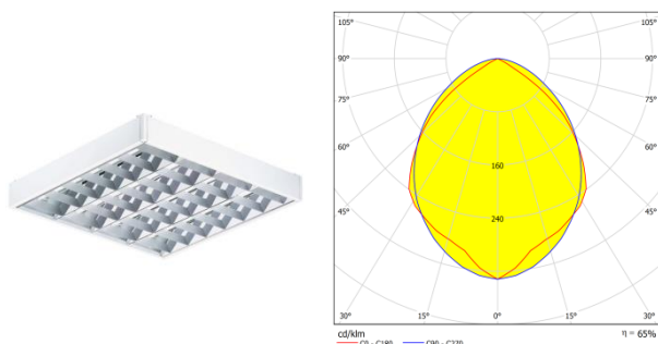
Figura 20. Corpo illuminante previsto nelle aule e relativa curva fotometrica con sorgente T5
