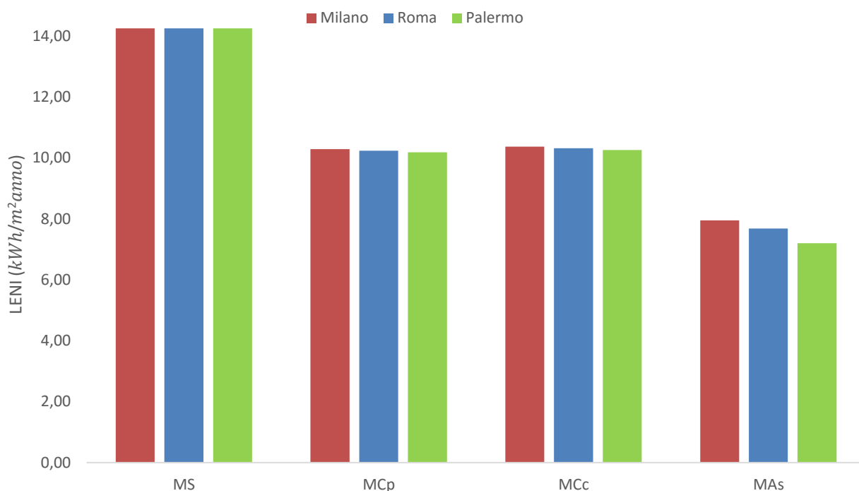
Figura 27. Confronto tra diversi metodi di calcolo LENI - ufficio 3.5 x 4.0 m con una finestra di dimensione 1.3 x 1.4 m, RAI 1/8, calcolato per \bar{E}_m di 500 lux
