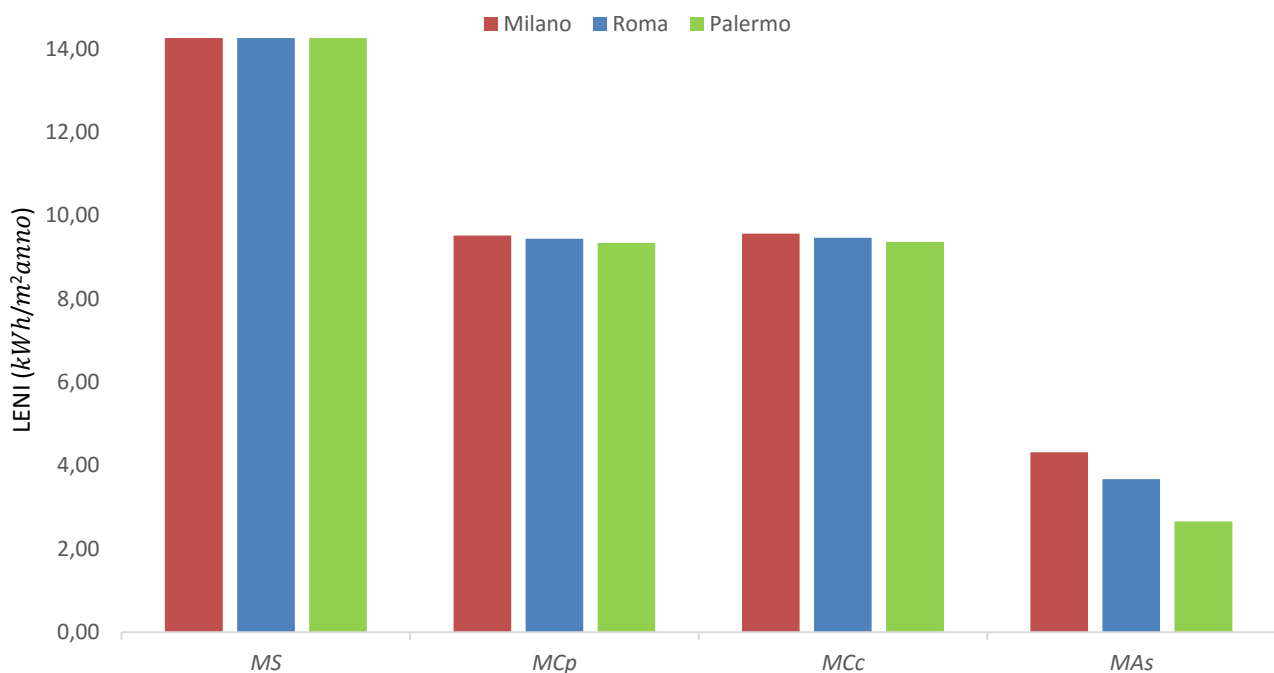
Figura 26. Confronto tra diversi metodi di calcolo LENI - ufficio 3.5 x 4.0 m con una finestra a nastro di dimensione 2.0 x 1.4 m RAI 1/5 , calcolato per \bar{E}_m di 500 lux
