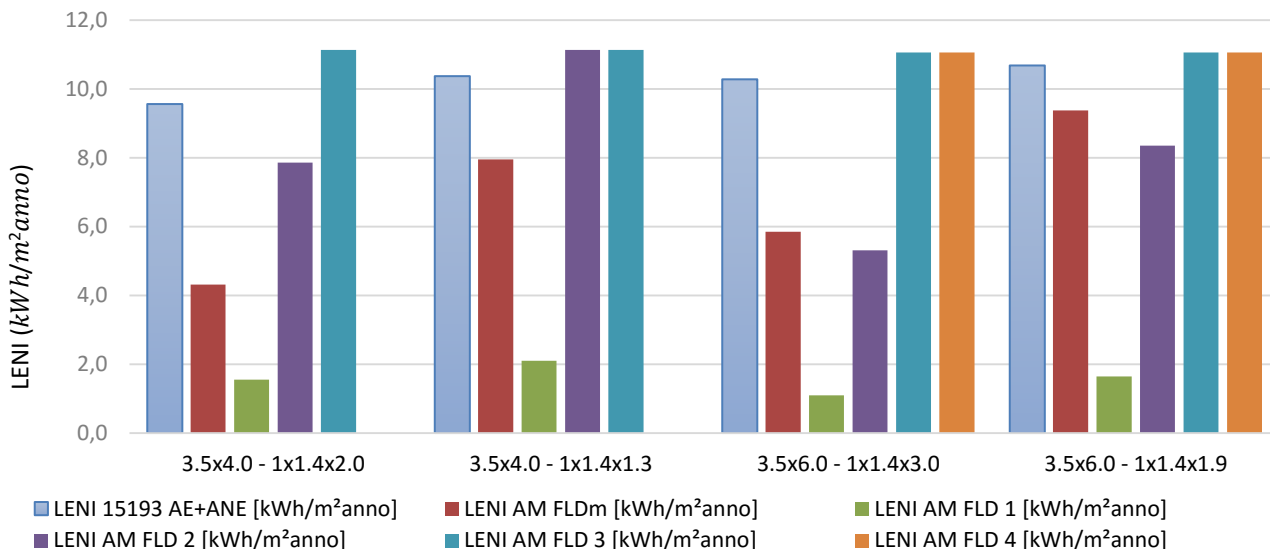
Figura 13. Confronto tra i valori del LENI per gli uffici situati idealmente a Milano
