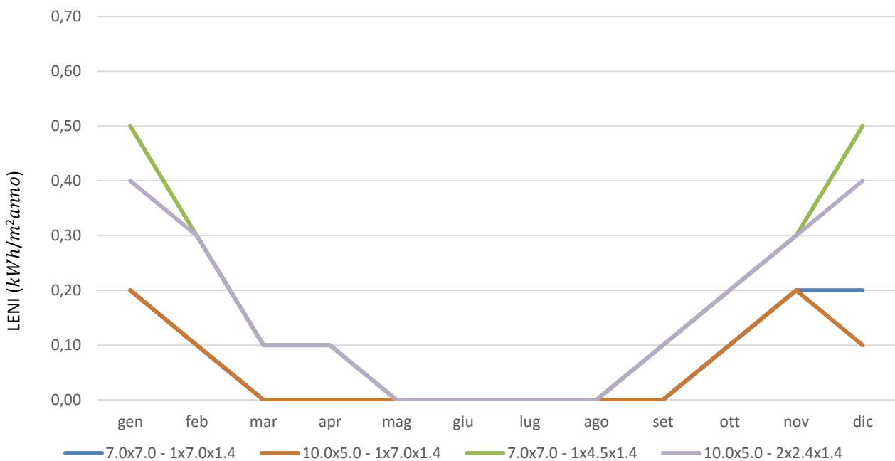
Figura 19. Aule scolastiche (Roma) - LENI mensile calcolato con il MAs
