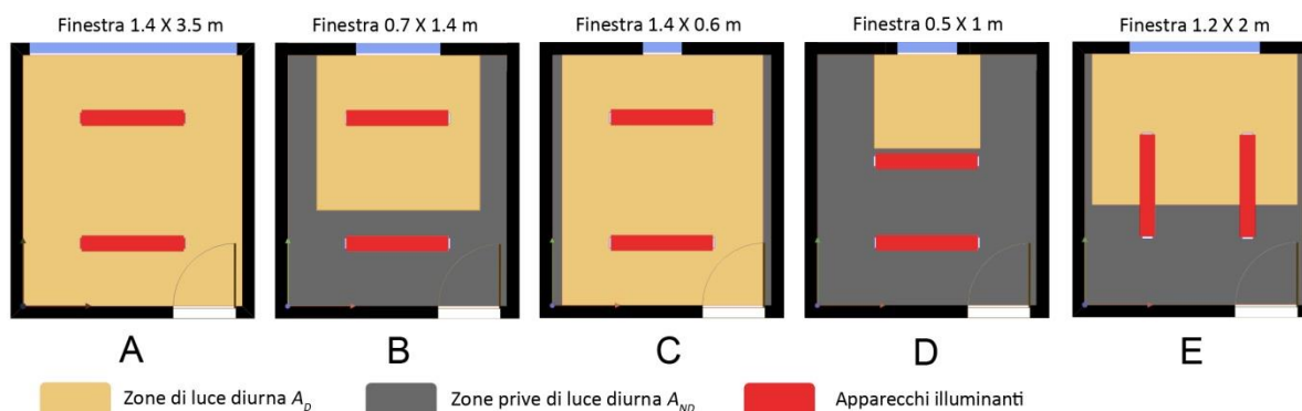
Figura 1. Possibili ripartizioni delle potenze degli apparecchi nelle zone di luce diurna A_D e delle zone prive di luce diurna A_{ND} - Caso esemplificativo di un locale di dimensioni 3,5 x 4 m e finestra di dimensioni variabili
