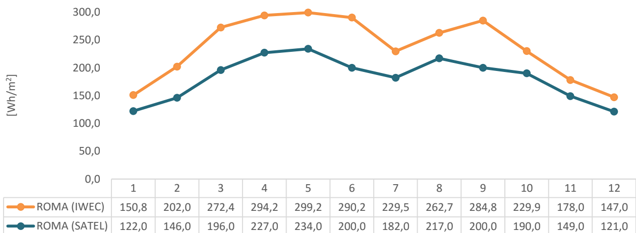
Figura 32. Confronto tra i dati di radiazione diffusa (valore medio mensile) dei file IWECC e di satel-light.com a Roma tra le 12 e le 13
