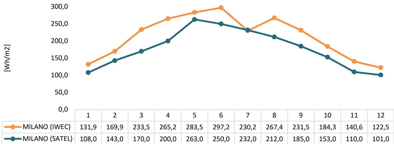
Figura 31. Confronto tra i dati di radiazione diffusa (valore medio mensile) dei file IWECC e di satel-light.com a Milano tra le 12 e le 13
