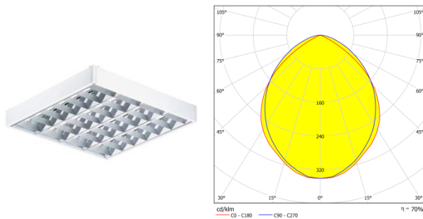
Figura 21. Corpo illuminante previsto nelle aule e relativa curva fotometrica con sorgente T8
