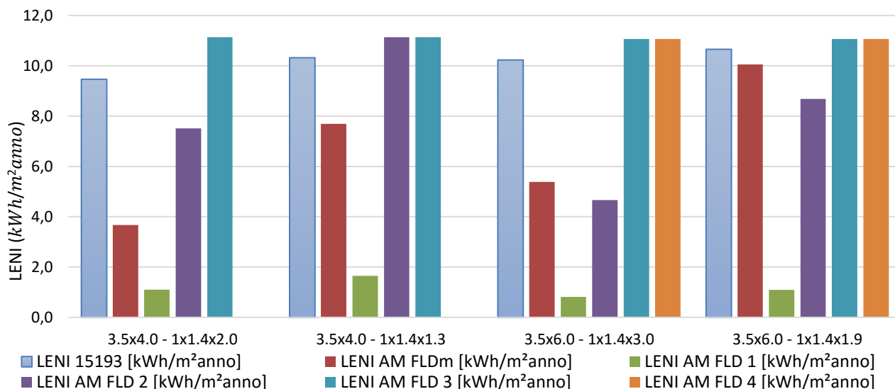
Figura 14. Confronto tra i valori del LENI per gli uffici situati idealmente a Roma
