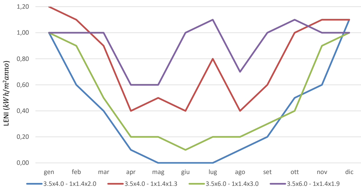
Figura 17. Uffici (Roma) - LENI mensile calcolato con il MAS
