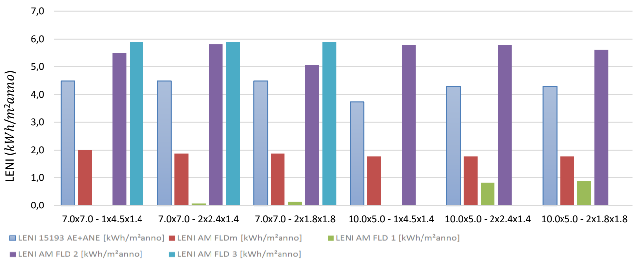
Figura 10. Confronto tra i valori del LENI per le aule scolastiche situate idealmente a Roma (RAI 1/8)
