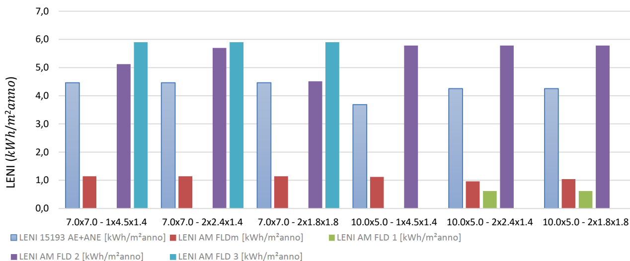
Figura 12. Confronto tra i valori del LENI per le aule scolastiche situate idealmente a Palermo ( RAI 1/8)
