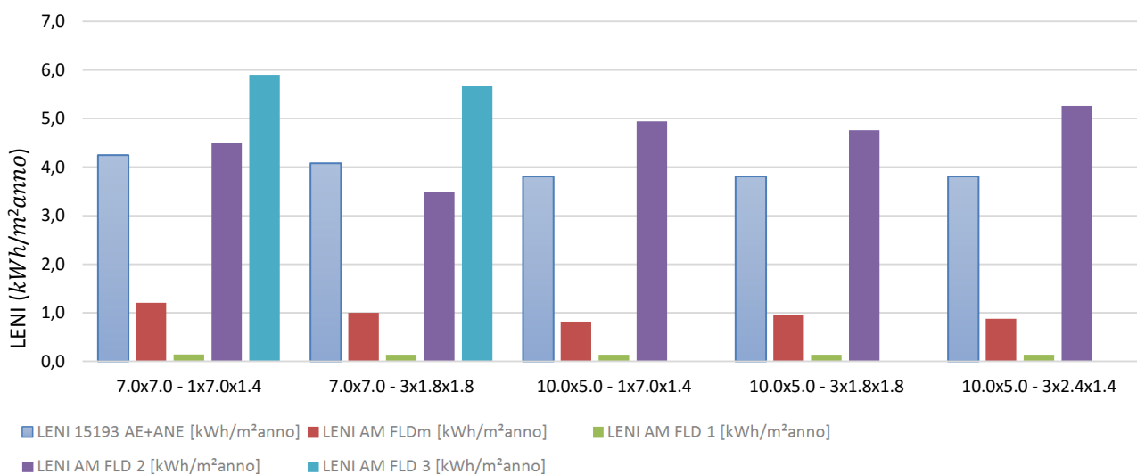
Figura 7. Confronto tra i valori del LENI per le aule scolastiche situate idealmente a Milano (RAI 1/5)
