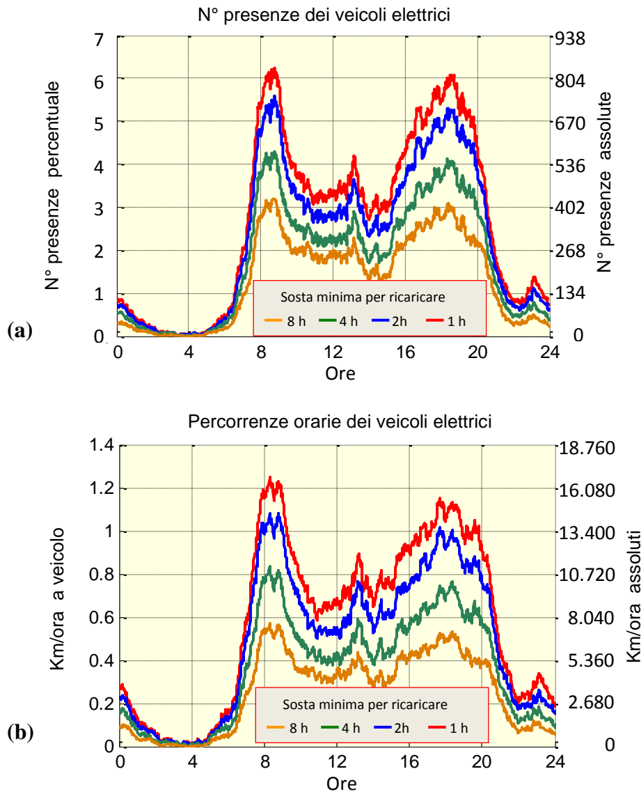
Figura 10 – Presenze e percorrenze orarie dei possibili VE di classe ‘Small’ ottenibili dal campione di riferimento nella giornata di lunedì 2 maggio. Le diverse curve dipendono dalla strategia di ricarica determinata dalla scelta della sosta minima per effettuare la ricarica del VE.
