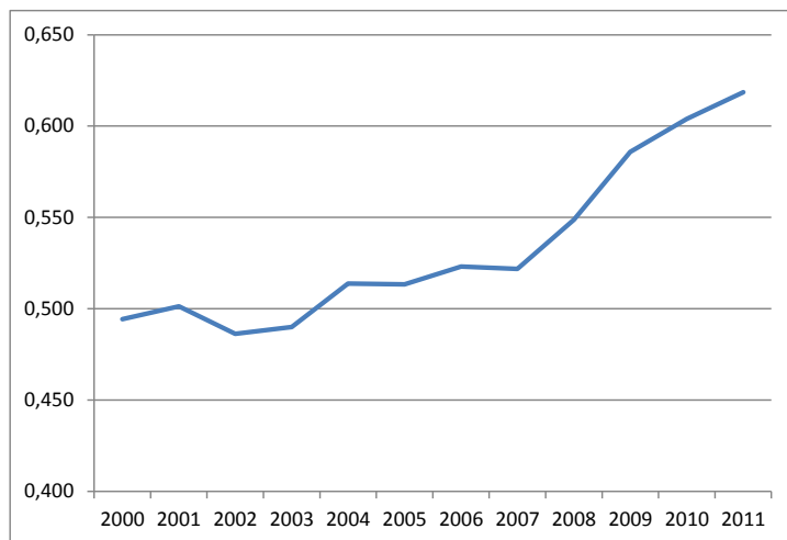
Figura 19: Produttività netta del parco elettrico italiano, 2000 – 2011 (Fonte: elaborazione ENEA su dati ISPRA, 2012)
