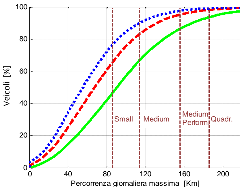
Figura 5 – La curva verde mostra la percentuale del CdR che nel mese non supera mai una percorrenza giornaliera. Lo stesso risultato, escludendo per ogni veicolo il giorno con la massima percorrenza, è mostrato dalla curva rossa mentre in azzurro si ha la curva escludendo i 2 giorni con la max percorrenza. Le linee verticali rappresentano l'autonomia delle varie classi di veicoli elettrici.
