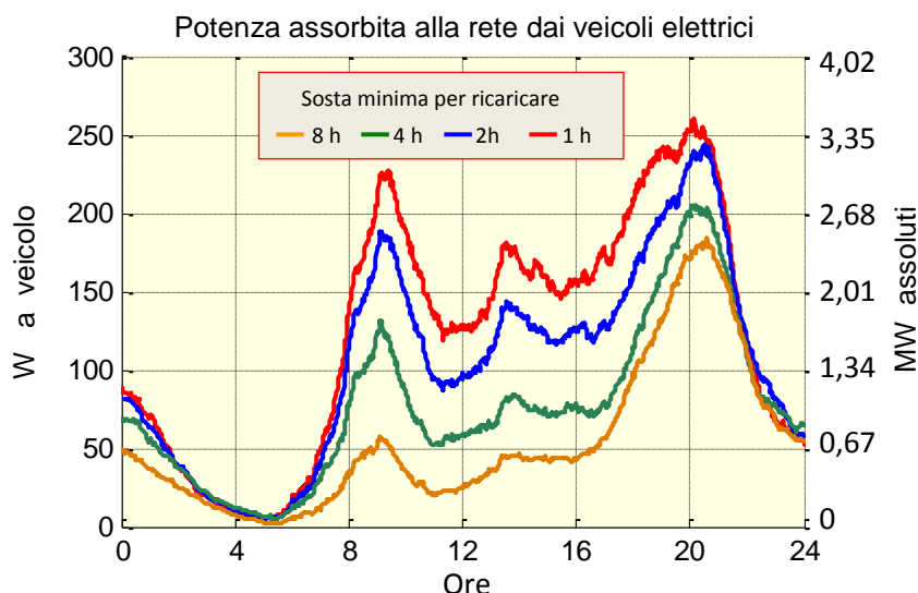
Figura 11 – Carico assorbito dalla rete elettrica per alimentare i VE di classe ‘Small’ con le percorrenze del grafico precedente con le curve dipendenti dalla diversa strategia di ricarica del VE
