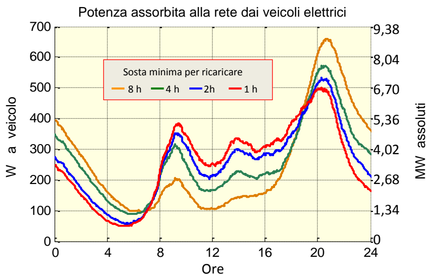
Figura 13 – Carico assorbito dalla rete elettrica per alimentare i VE di classe ‘Large’ con le percorrenze del grafico precedente con le curve dipendenti dalla diversa strategia di ricarica del VE
