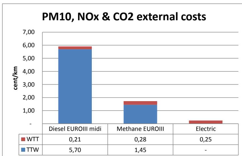
Figura 23: Costo esterno unitario delle emissioni di NOx, PM and CO2 per bus urbani di diverse motorizzazioni (Stime ENEA da diverse fonti dati )
