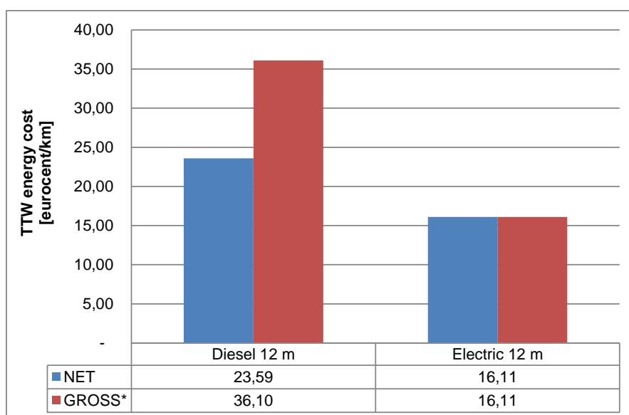
Figura 18: Costi energetici di esercizio per bus urbani diesel ed elettrici, al netto ed al lordo delle accise (Fonte: elaborazione ENEA su dati vari)
