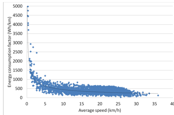
Figura 21: Consumo specifico in funzione della velocità media di viaggio (Fonte dati: sperimentazione CTL-ENEA nell'ambito del progetto Smartcities)
