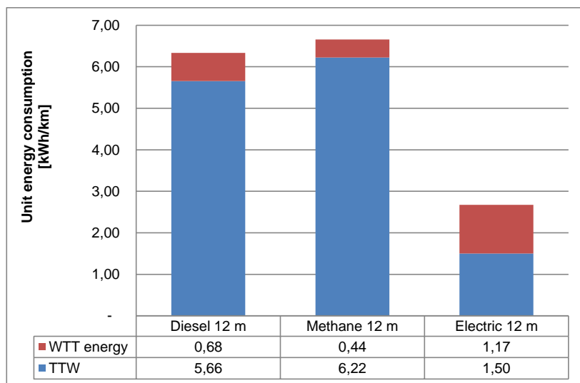
Figura 17: Consumo specifico caratteristico di bus urbani per tipo di motorizzazione Tank-to-wheel (TTW) e Well-to-Tank (WTT) (Fonte dati: ENEA)
