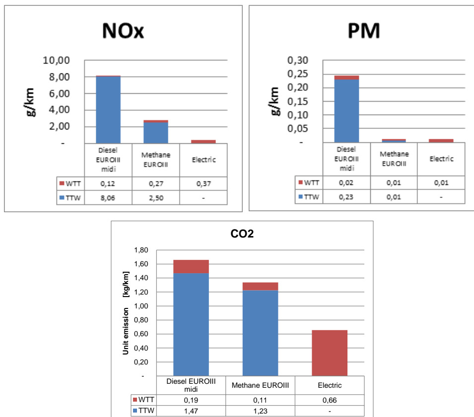
Figura 22: Emissioni specifiche Tank-to-wheel e Well-to-Tank Urban dei bus urbani per tipo di motorizzazione (Fonte: ENEA and ISPRA, 2011)
