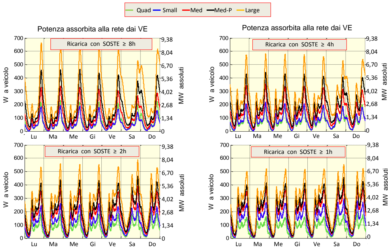
Figura 9 – Nella prima settimana di maggio, per le 5 classi di VE, riportate in legenda, nei 4 grafici sono riportate le potenze assorbite dalla rete elettrica per alimentare i VE con le percorrenze ottenute dai VE sottoposti alle 4 differenti soste di ricarica considerate.
