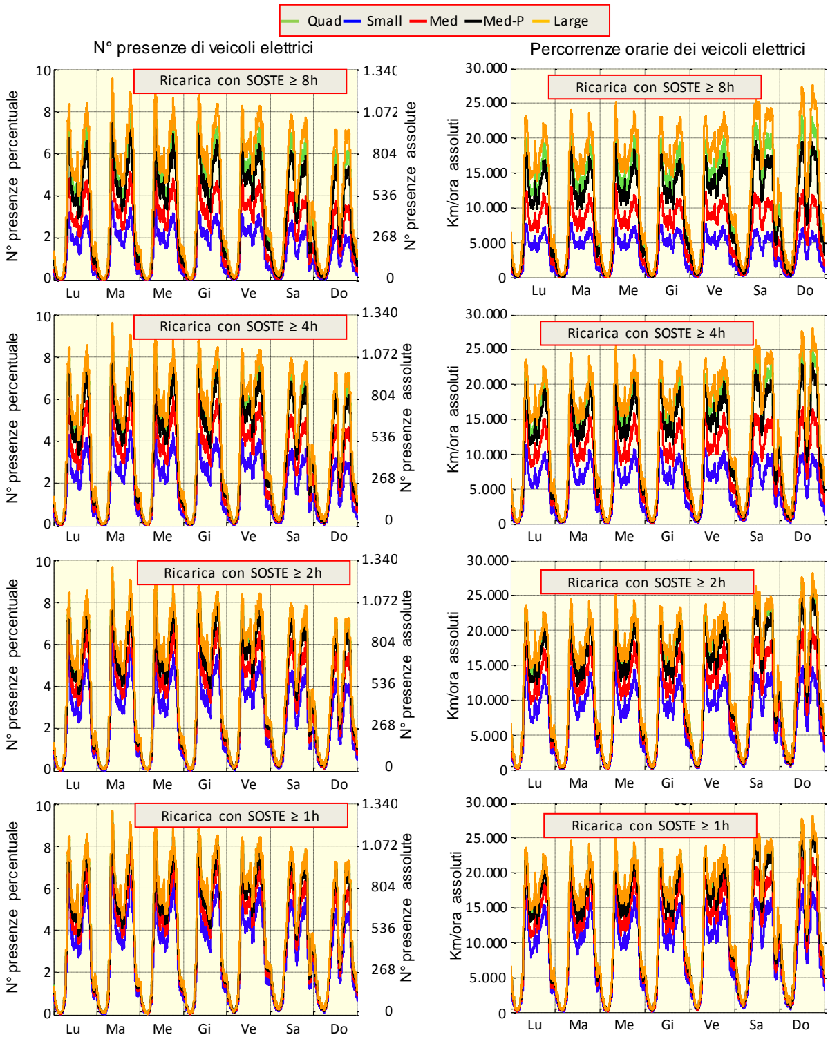
Figura 7 – Nella prima settimana di maggio, per le 5 classi di VE, riportate in leggenda, nei grafici a sx sono rappresentati il numero di possibili presenze di VE per ognuna delle 4 soste minime previste per la ricarica. A dx sono rappresentate le relative percorrenze orarie. Le ordinate sono riportate a sx con valori percentuali e a dx in assoluto.
