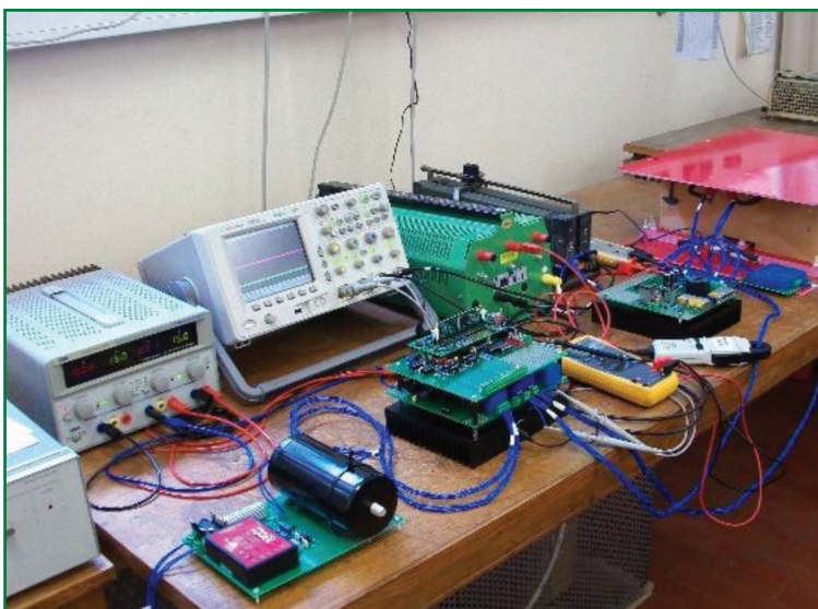
Banco prova del sistema contactless
