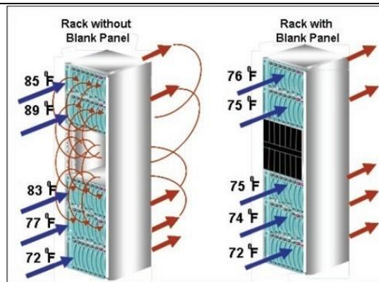
Figura 39: Importanza dei pannelli di chiusura degli spazi vuoti per evitare ricircoli di aria calda [24]
