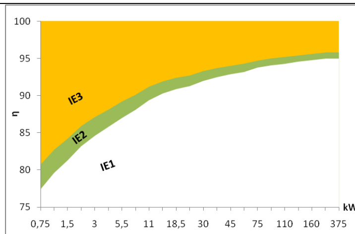
Figura 26: Classi di efficienza motori a 2 poli
