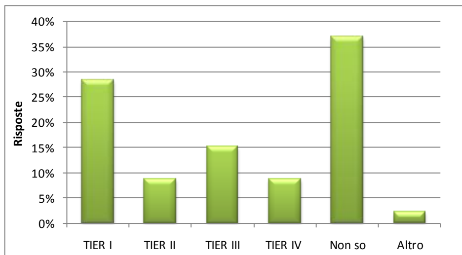
Figura 72 Livello di ridondanza dell'alimentazione elettrica
