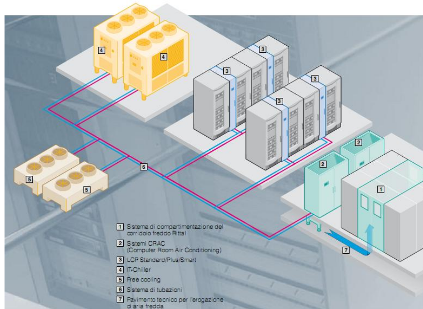
Figura 47: Esempio di sistema di raffreddamento a liquido all'interno di armadi rack 3 integrato con un sistema tradizionale a pavimento flottante 2 [56]
