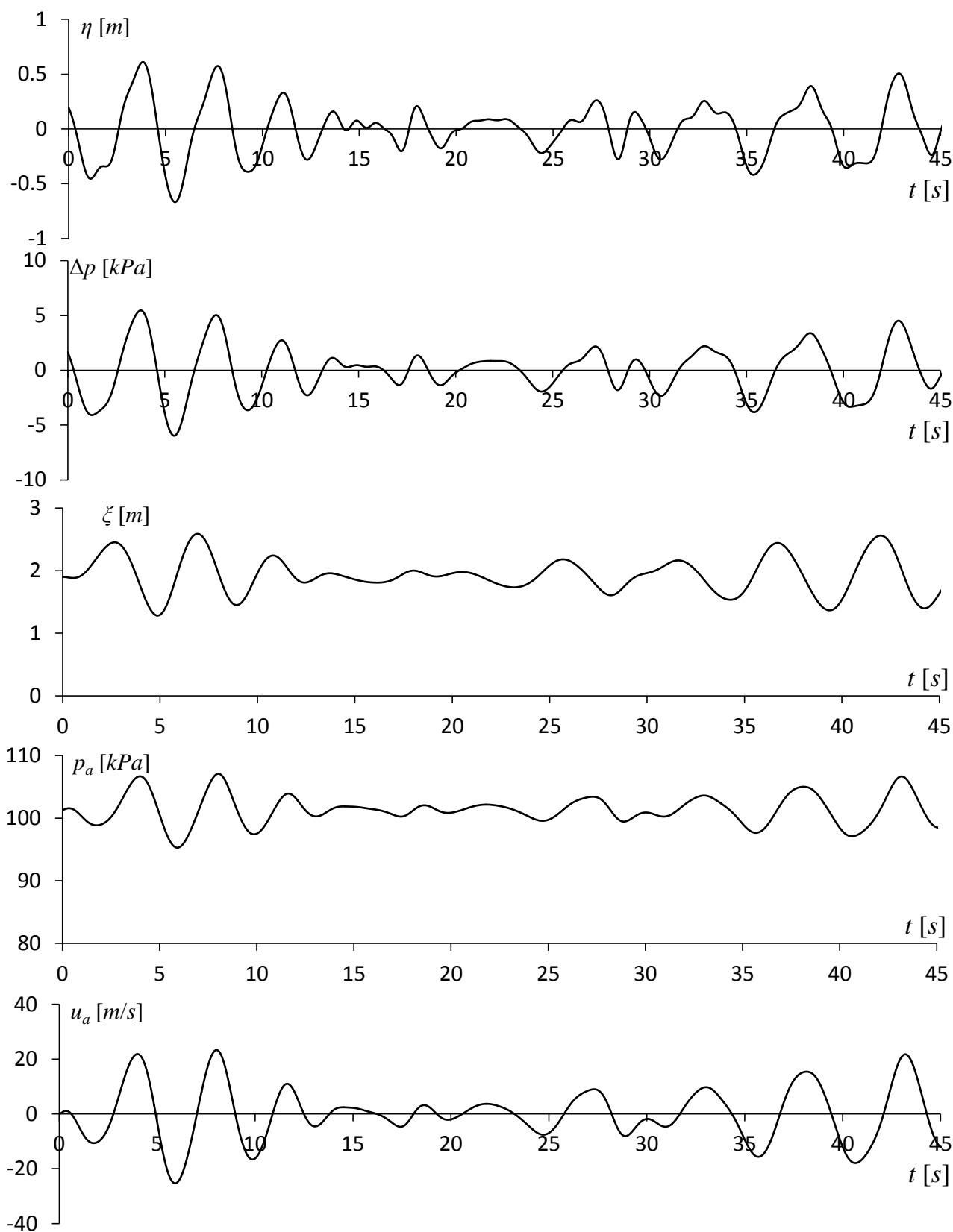
Figura 17. Registrazioni relative ad uno stato di mare con spettro di frequenza JONSWAP medio e altezza significativa H_s=1.2m , per REWEC3 con camera partizionata. In particolare, dal pannello superiore si ha: superficie libera di fronte alla parete (pannello 1); fluttuazione di pressione all’imboccatura (pannello 2); superficie libera nella camera di assorbimento misurata dalla cima della camera (pannello 3); pressione nella camera d’aria (pannello 4); velocità dell’aria nel condotto ospitante la turbina (pannello 5).
