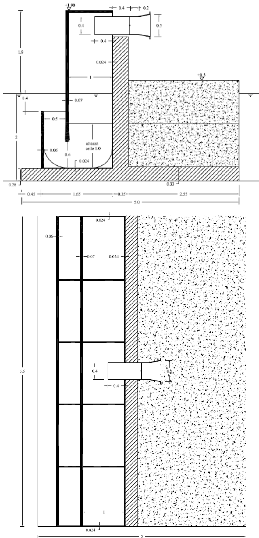
Figura 6. Sezione trasversale (in alto) e pianta (in basso) del modello di U-OWC utilizzato presso il NOEL. Quote e dimensioni sono espresse in metri – progetti Wavenergy.it finanziato dal polo NET e POSEIDONE.
