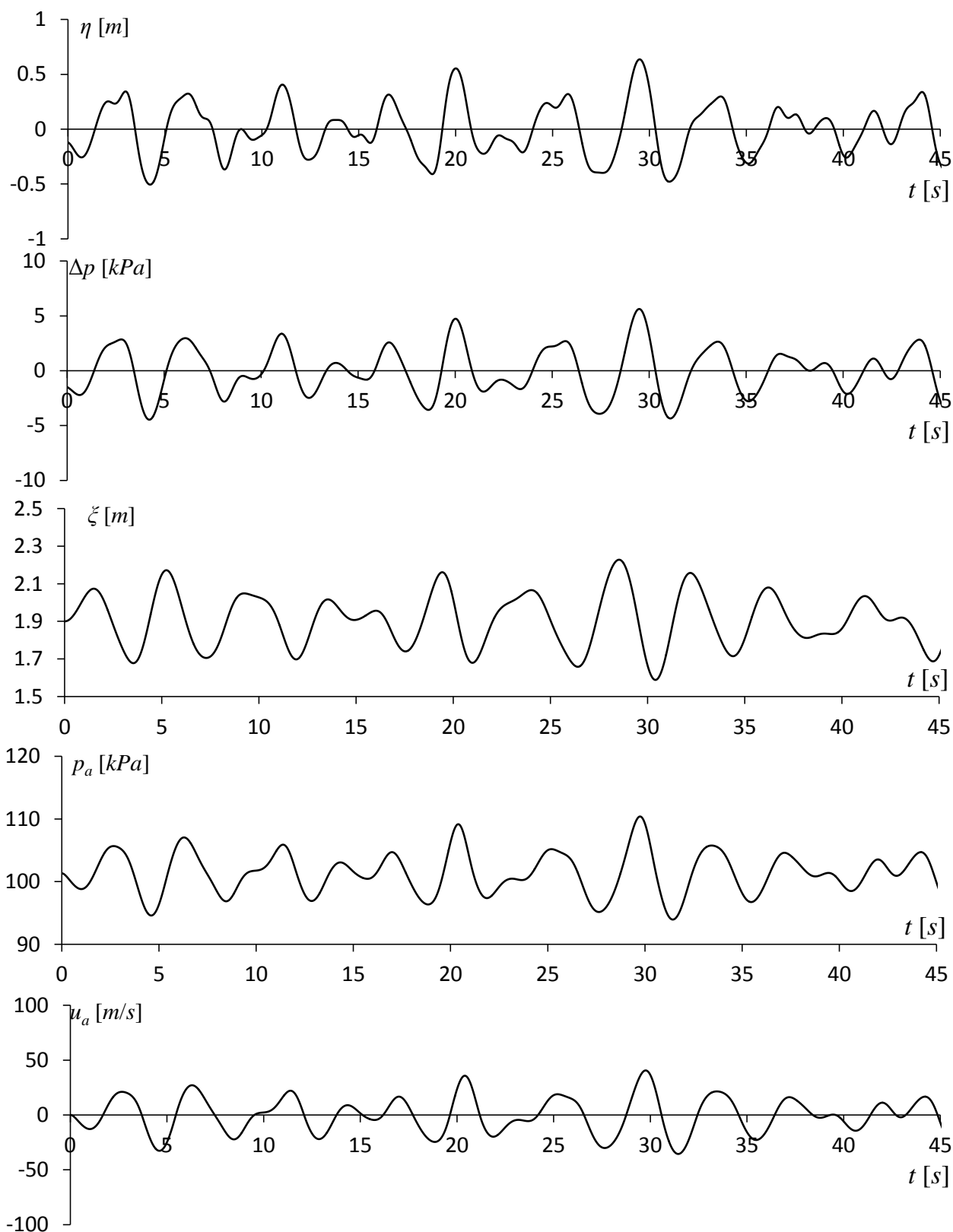
Figura 11. Regrazioni relative ad uno stato di mare con spettro di frequenza JONSWAP medio e altezza significativa H_s=1.0m . In particolare, dal pannello superiore si ha: superficie libera di fronte alla parete (pannello 1); fluttuazione di pressione all'imboccatura (pannello 2); superficie libera nella camera di assorbimento misurata dalla cima della camera (pannello 3); pressione nella camera d'aria (pannello 4); velocità dell'aria nel condotto ospitante la turbina (pannello 5). [Simulazioni eseguite nell'ambito del progetto POSEIDONE].
