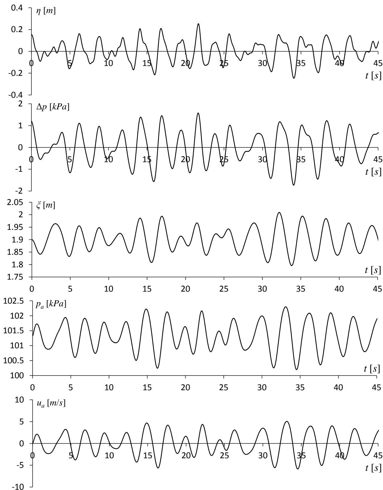
Figura 13. Registrazioni relative ad uno stato di mare con spettro di frequenza JONSWAP medio e altezza significativa H_s=0.4\text{m} , per REWEC3 con camera partizionata. In particolare, dal pannello superiore si ha: superficie libera di fronte alla parete (pannello 1); fluttuazione di pressione all'imboccatura (pannello 2); superficie libera nella camera di assorbimento misurata dalla cima della camera (pannello 3); pressione nella camera d'aria (pannello 4); velocità dell'aria nel condotto ospitante la turbina (pannello 5).
