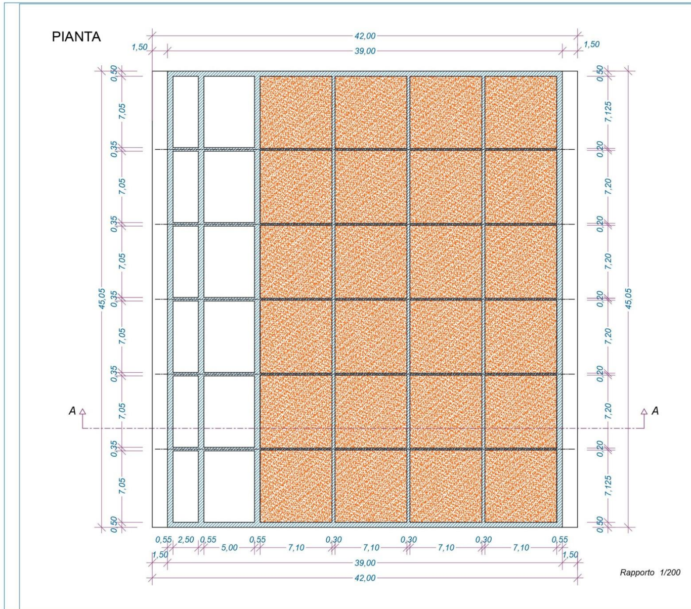
Figura A.2 Pianta dell'U-OWC incorporato in diga portuale per la località di Capo dell'Argentiera (Sardegna Nord-Ovest).
