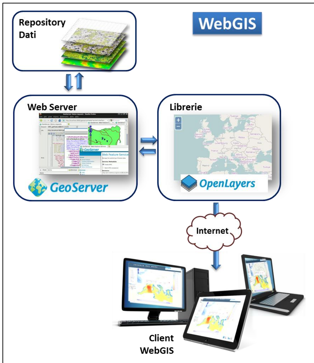
Figura 42. Architettura logica del WebGIS implementato
