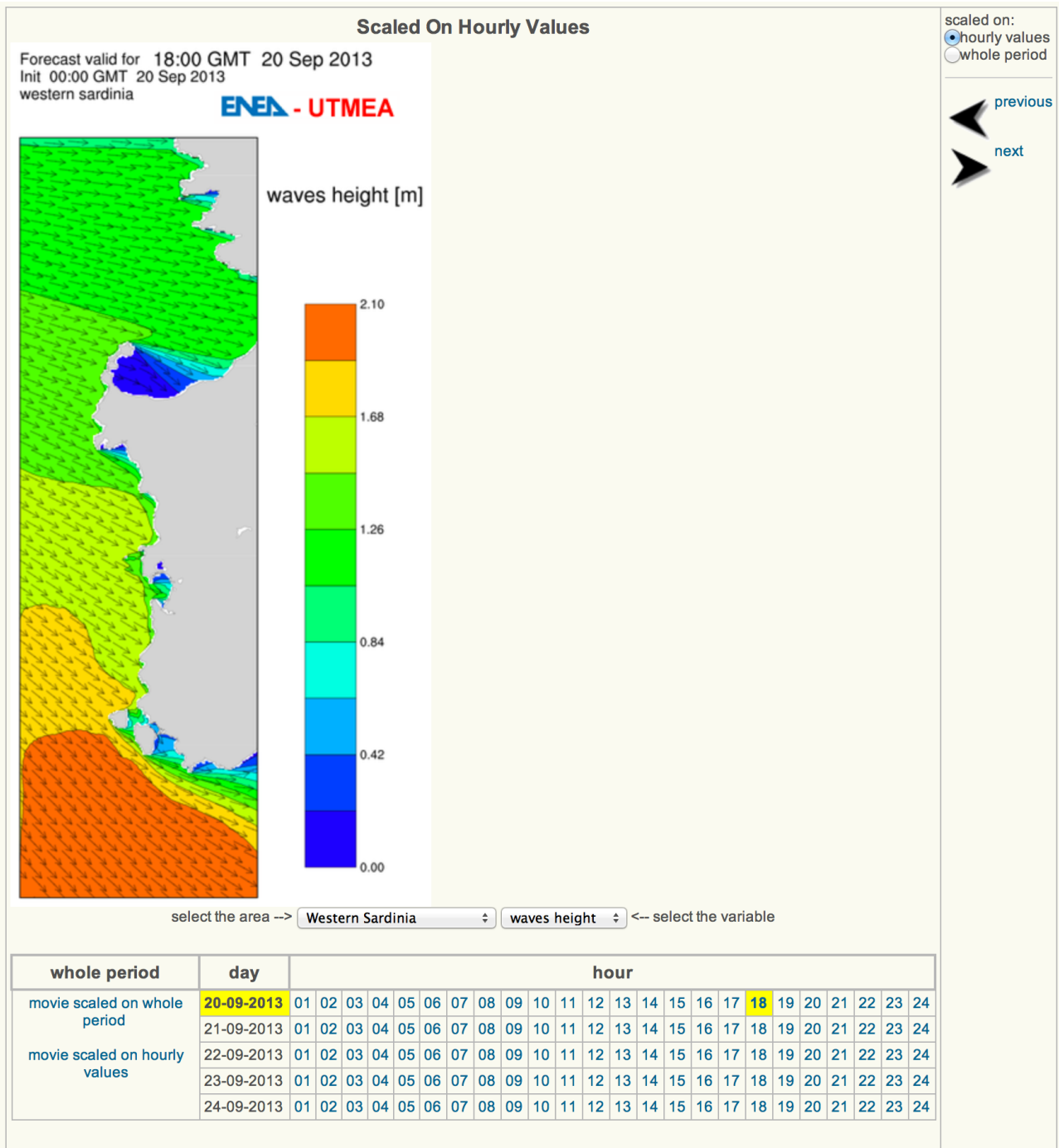
Figura 13. Esempio di previsione di altezza significativa delle onde per la zona ovest della Sardegna tratta dal sito UTMEA.
