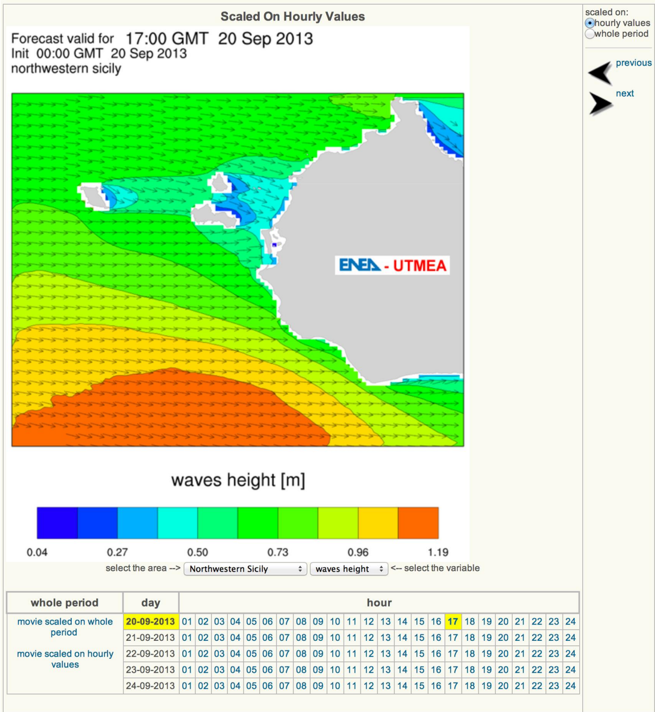
Figura 19. Esempio di previsione di altezza significativa delle onde per l'area nord-occidentale della Sicilia tratta dal sito UTMEA.
