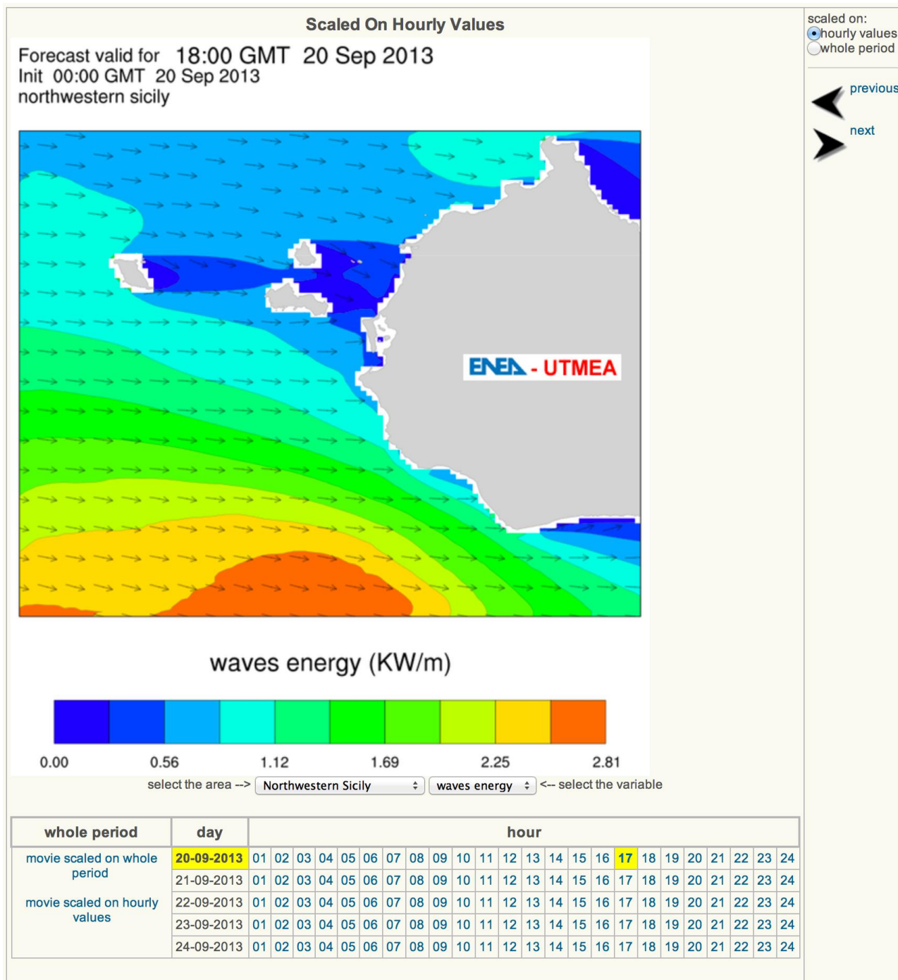
Figura 18. Esempio di previsione di energia delle onde per la zona nord-occidentale della Sicilia tratta dal sito UTMEA.
