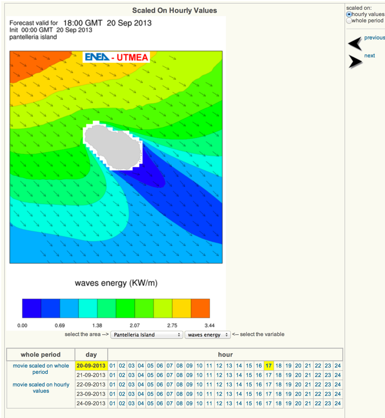
Figura 14. Esempio di previsione di energia delle onde per l'isola di Pantelleria tratta dal sito UTMEA.
