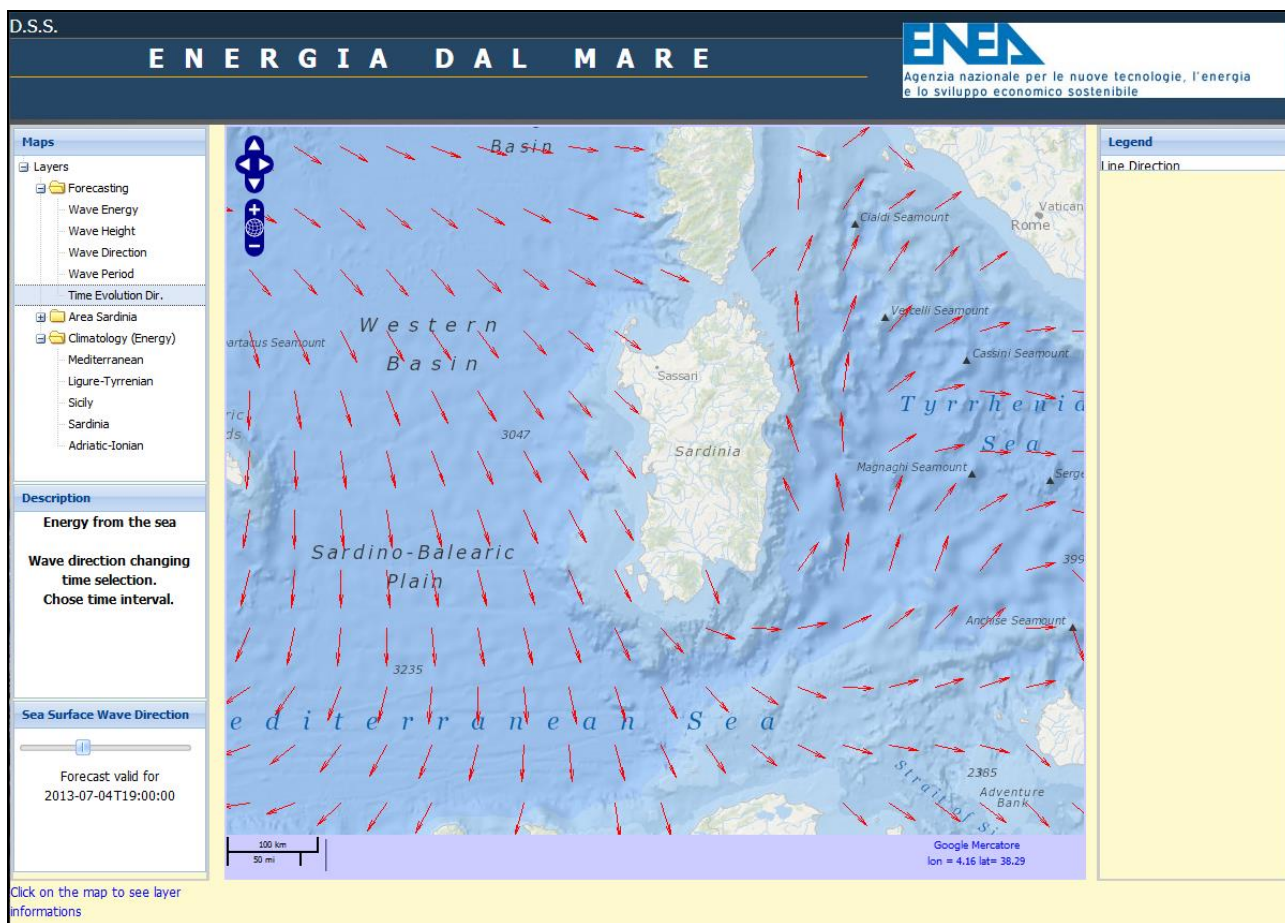
Figura 47. Evoluzione temporale della direzione delle onde (sequenza oraria attivabile mediante comando “slider”, in basso a sinistra).
