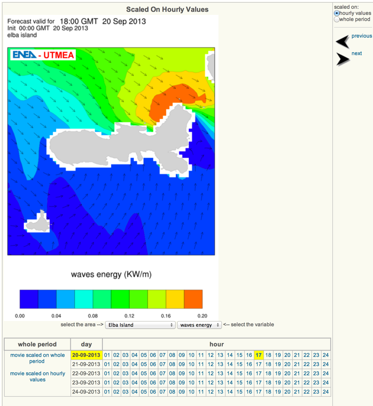
Figura 24. Esempio di previsione di energia delle onde per la zona dell'isola d'Elba tratta dal sito UTMEA.
