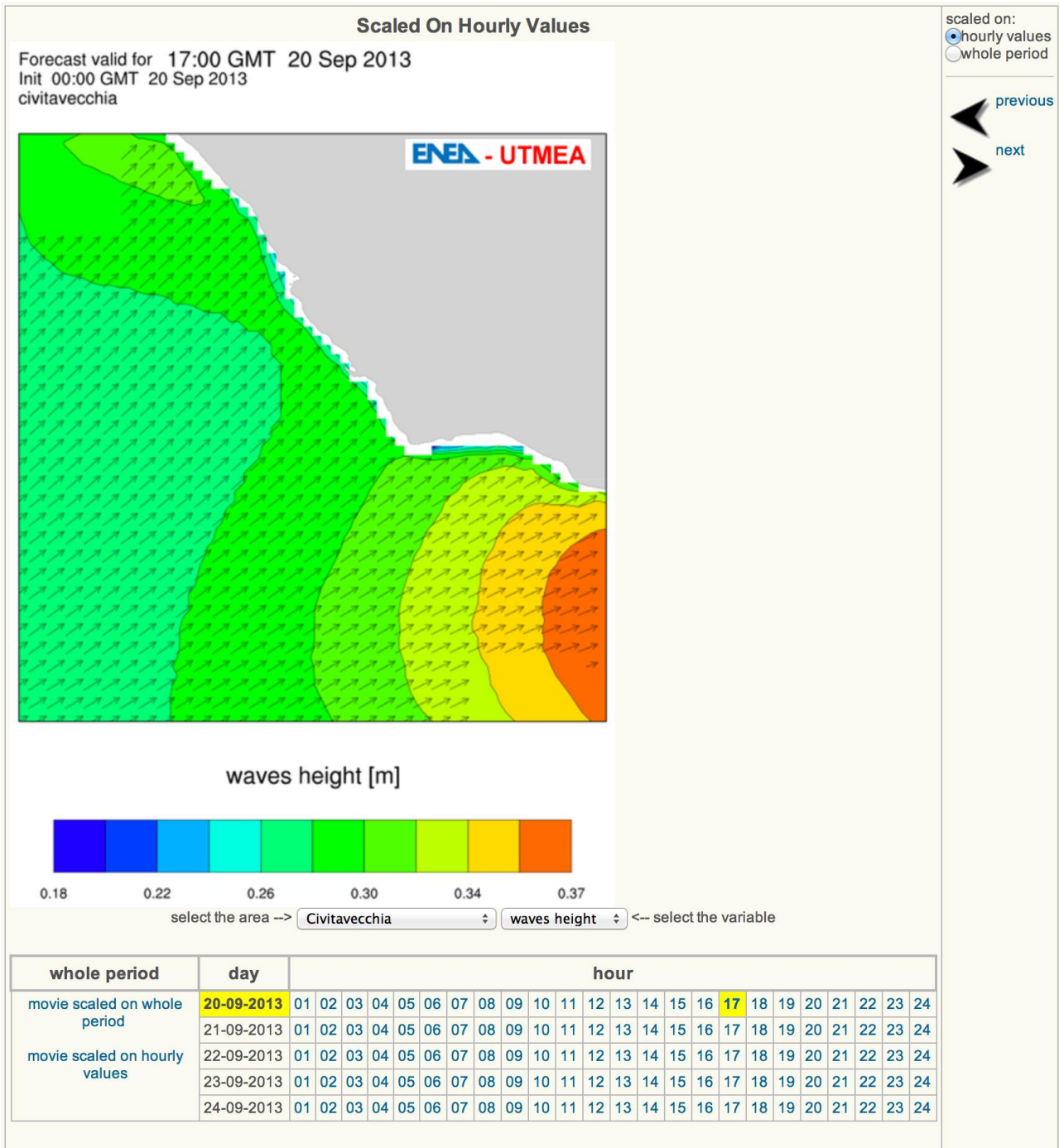
Figura 21. Esempio di previsione di altezza significativa delle onde per la zona di Civitavecchia tratta dal sito UTMEA.
