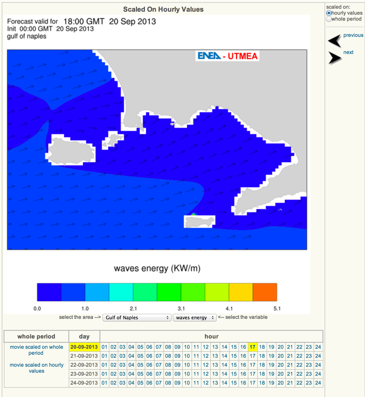
Figura 28. Esempio di previsione di energia delle onde per la zona del Golfo di Napoli tratta dal sito UTMEA.
