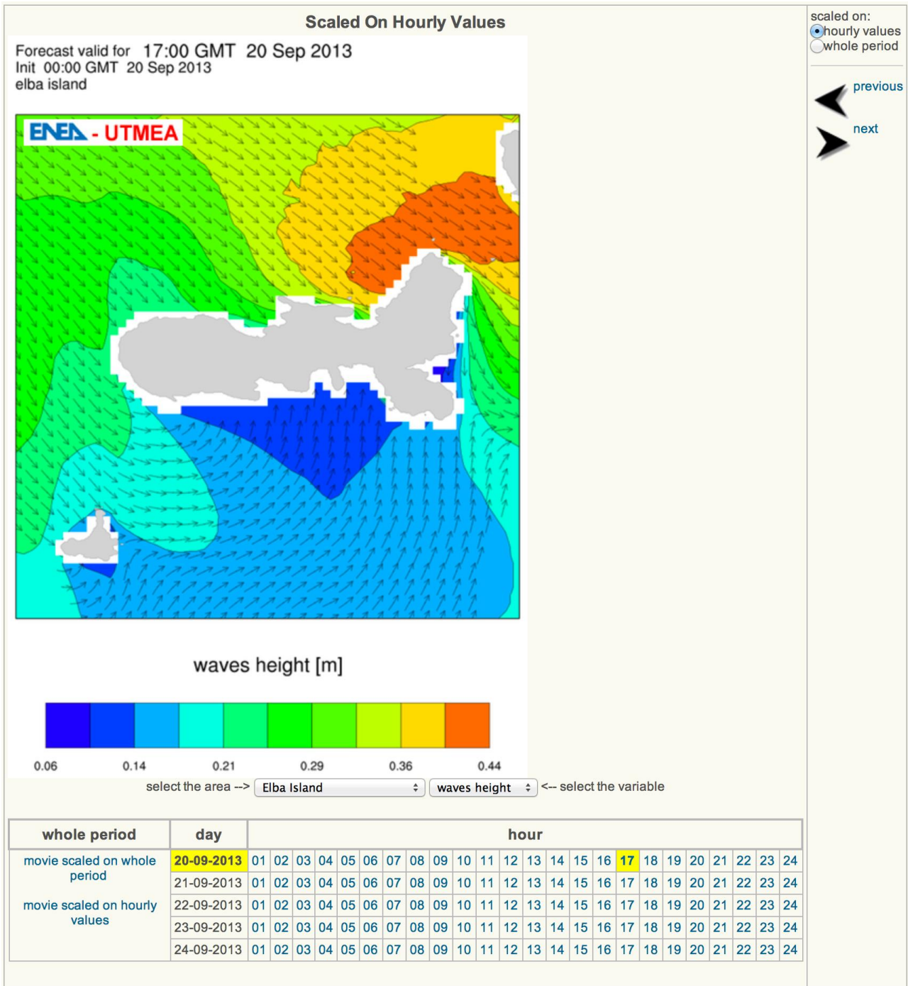
Figura 25. Esempio di previsione di altezza significativa delle onde per la zona dell'isola d'Elba tratta dal sito UTMEA.
