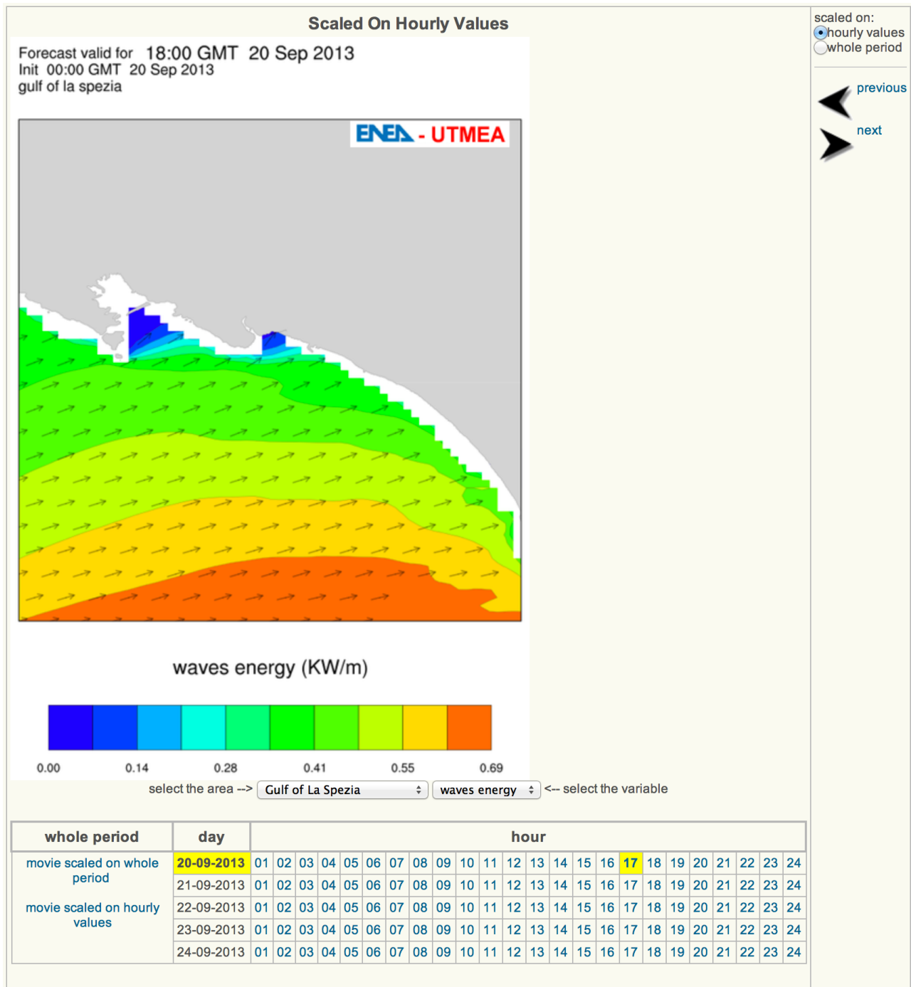
Figura 22. Esempio di previsione di energia delle onde per la zona del Golfo di La Spezia tratta dal sito UTMEA
