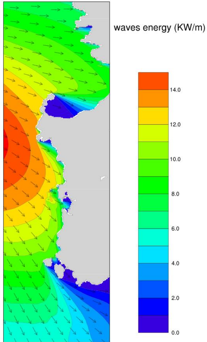
Figura 32. Esempio di previsione di energia per il sottobacino della Sardegna. Previsione per le ore 12 del giorno 13 settembre 2013.
