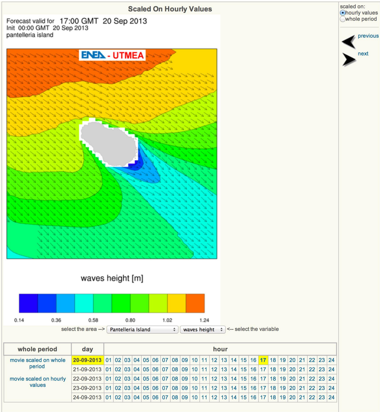
Figura 15. Esempio di previsione di altezza significativa delle onde per l'isola di Pantelleria tratta dal sito UTMEA.
