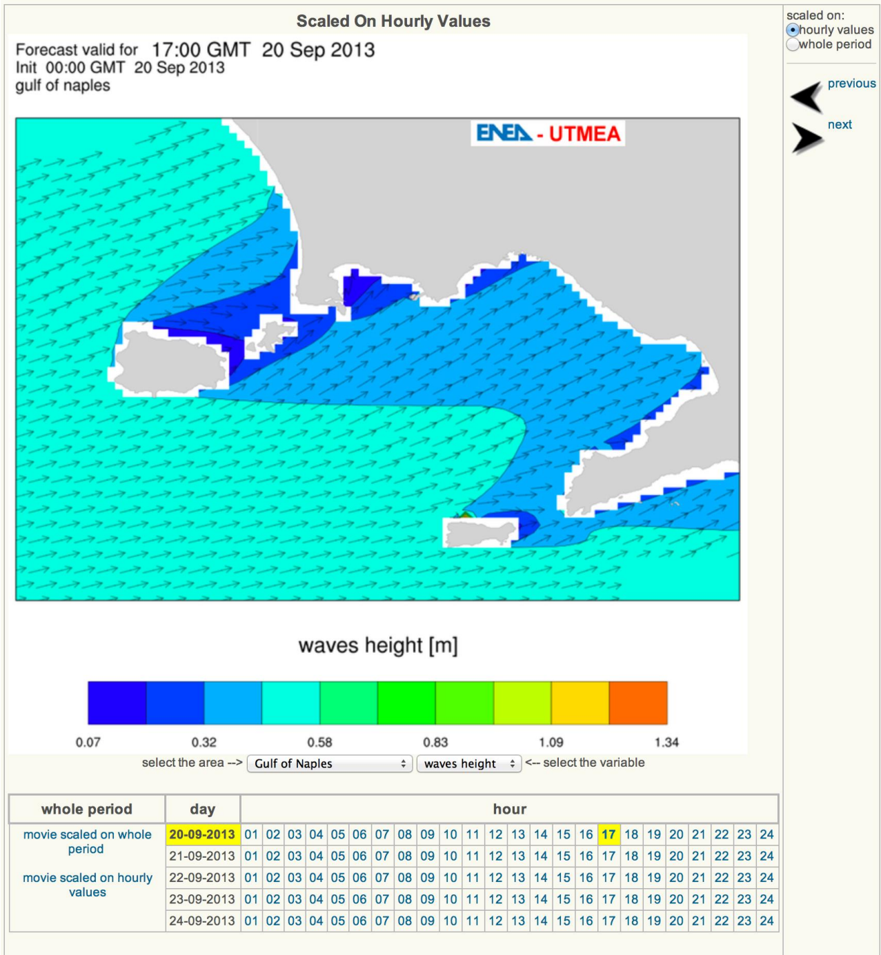
Figura 29. Esempio di previsione di altezza significativa delle onde per la zona del Golfo di Napoli tratta dal sito UTMEA.
