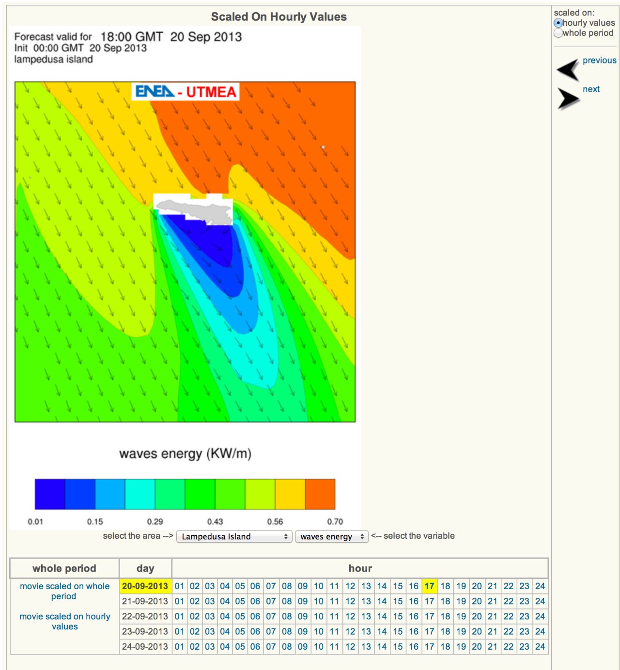
Figura 16. Esempio di previsione di energia delle onde per l'isola di Lampedusa tratta dal sito UTMEA.
