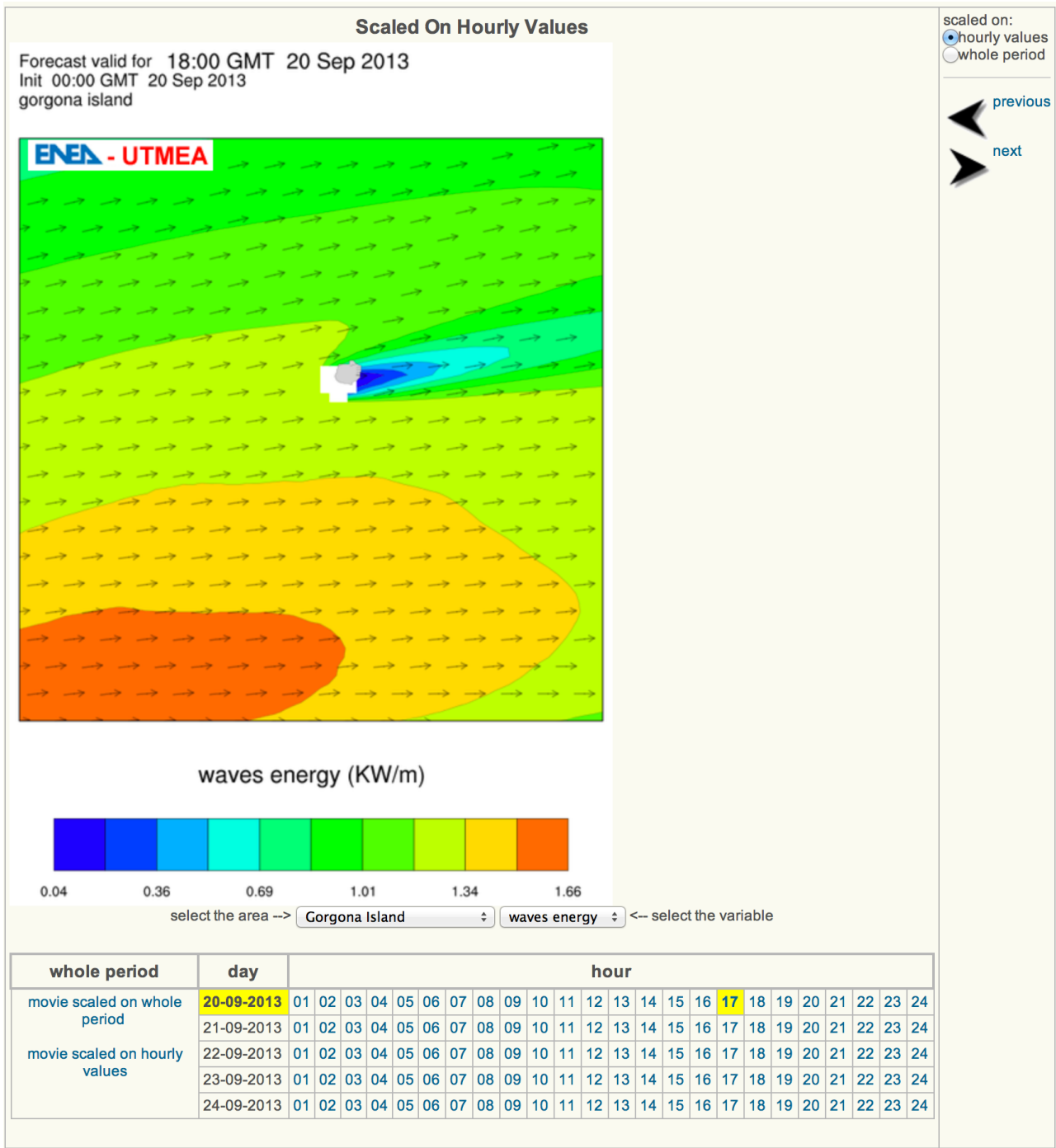
Figura 30. Esempio di previsione di energia delle onde per la zona dell'isola di Gorgona tratta dal sito UTMEA.
