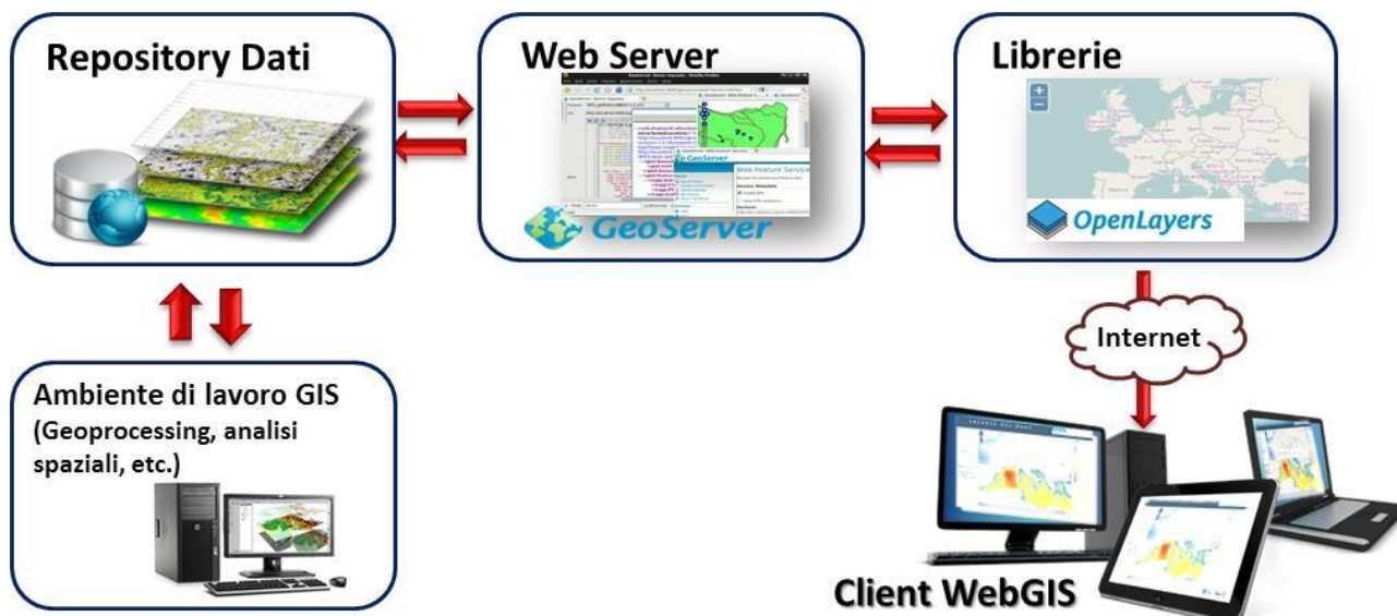
Figura 1. Schema architetturale dell'applicazione WebGIS "Waves Energy"
