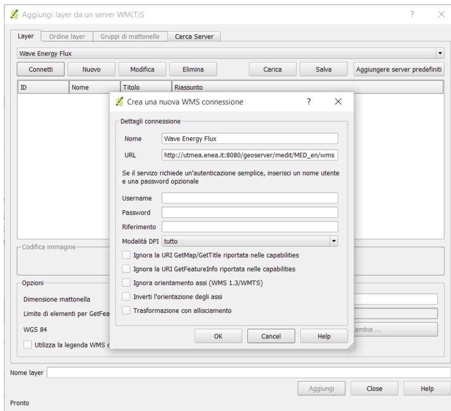
Figura 9. Finestra di dialogo di QGIS per la definizione di un servizio WMS e l'inserimento di un servizio o di un layer da visualizzare nel proprio client standalone
