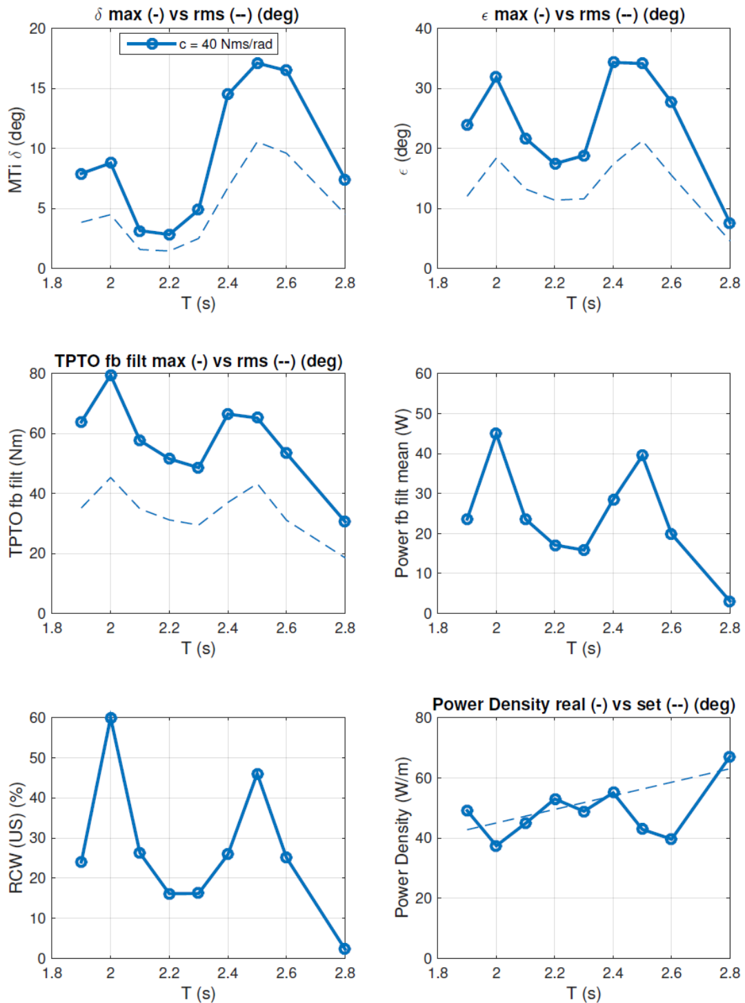
Figura 30 – risposta in frequenza per c = 40 Nms/rad.
